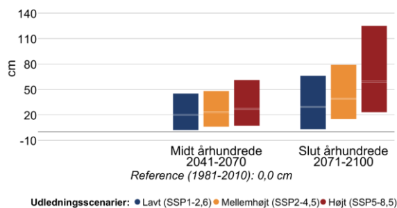
Figur 12 Ændring i middelvandstand (venstre) og hyppigheden af stormflod for Skagerrakkyst sydlige i fremtidsperioderne 2041-2070 og 2071-2100 under forskellige udledningsscenarier. Den grå linje viser referenceværdien for nutiden (1981-2010). En stormflod defineres her som en forhøjet vandstand, der statistisk set kun forekommer én gang hvert 20. år i perioden 1981-2010. Bemærk også at denne indikator kappes ved 60 stormfloder per 20 år.
