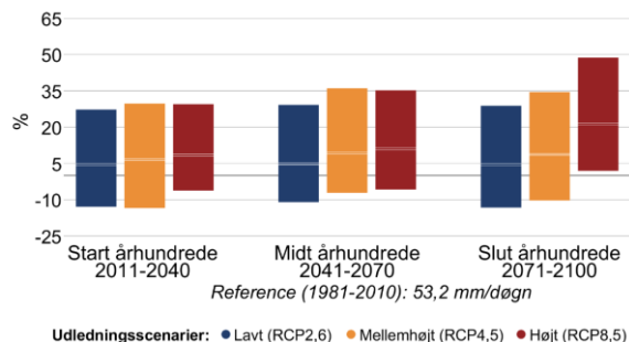
Figur 7 Procentvis ændring af ekstremnedbør hen over året mellem 1981-2010 og fremtidsperioderne 2011-2040, 2041-2070 og 2071-2100 under forskellige udledningsscenarier i Thisted Kommune. Til venstre 10-årshændelsen for døgnnedbør, til højre frekvensen af skybrud.
