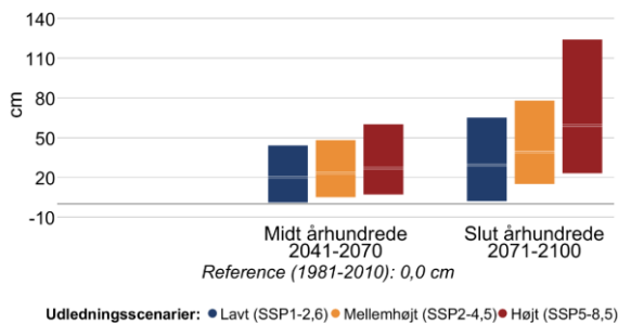
Figur 16 Ændring i middelvandstand (venstre) og hyppigheden af stormflod for Limfjorden ved Thisted i fremtidsperioderne 2041-2070 og 2071-2100 under forskellige udledningsscenarier. Den grå linje viser referenceværdien for nutiden (1981-2010). En stormflod defineres her som en forhøjet vandstand, der statistisk set kun forekommer én gang hvert 20. år i perioden 1981-2010. Bemærk også at denne indikator kappes ved 60 stormfloder per 20 år.
