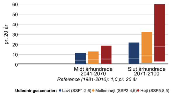
Figur 16 Ændring i middelvandstand (venstre) og hyppigheden af stormflod for Limfjorden ved Thisted i fremtidsperioderne 2041-2070 og 2071-2100 under forskellige udledningsscenarier. Den grå linje viser referenceværdien for nutiden (1981-2010). En stormflod defineres her som en forhøjet vandstand, der statistisk set kun forekommer én gang hvert 20. år i perioden 1981-2010. Bemærk også at denne indikator kappes ved 60 stormfloder per 20 år.
