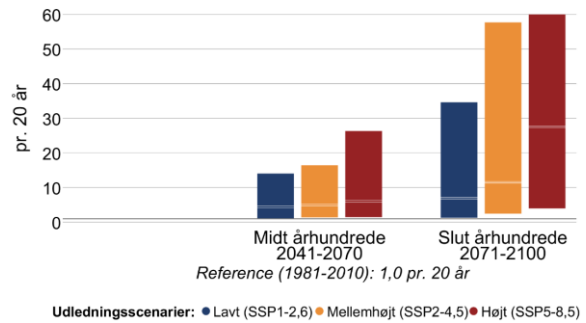
Figur 14 Ændring i middelvandstand (venstre) og hyppigheden af stormflod for Limfjorden ved Lemvig i fremtidsperioderne 2041-2070 og 2071-2100 under forskellige udledningsscenarier. Den grå linje viser referenceværdien for nutiden (1981-2010). En stormflod defineres her som en forhøjet vandstand, der statistisk set kun forekommer én gang hvert 20. år i perioden 1981-2010. Bemærk også at denne indikator kappes ved 60 stormfloder per 20 år.
