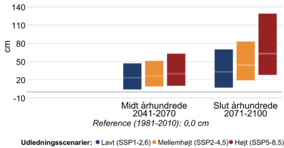
Figur 14 Ændring i middelvandstand (venstre) og hyppigheden af stormflod for Limfjorden ved Lemvig i fremtidsperioderne 2041-2070 og 2071-2100 under forskellige udledningsscenarier. Den grå linje viser referenceværdien for nutiden (1981-2010). En stormflod defineres her som en forhøjet vandstand, der statistisk set kun forekommer én gang hvert 20. år i perioden 1981-2010. Bemærk også at denne indikator kappes ved 60 stormfloder per 20 år.
