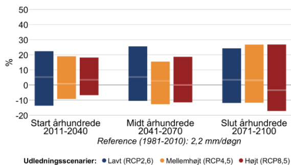
Figur 6 Procentvis ændring af middelnedbør mellem 1981-2010 og fremtidsperioderne 2011-2040, 2041-2070 og 2071-2100 under forskellige udledningsscenarier i Thisted Kommune. Til venstre sommer (jun-aug), til højre vinter (dec-feb).
