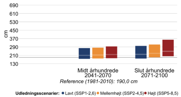
Figur 17 Højden af 20- (venstre) og 100-års (højre) stormflodhændelser for Limfjorden ved Thisted i fremtidsperioderne 2041-2070 og 2071-2100 under forskellige udledningsscenarier. Den grå linje viser referenceværdien for nutiden (1981-2010).
