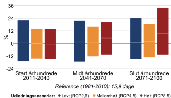
Figur 8 Procentvis ændring af tørre dage om sommeren (jun-aug) mellem 1981-2010 og fremtidsperioderne 2011-2040, 2041-2070 og 2071-2100 under forskellige udledningsscenarier i Thisted Kommune. Til venstre antallet af tørre dage med mindre end 1 mm nedbør, til højre længden af den længste sammenhængende tørre periode.
