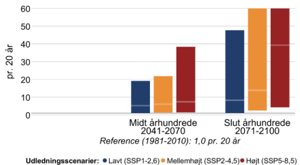
Figur 12 Ændring i middelvandstand (venstre) og hyppigheden af stormflod for Skagerrakkyst sydlige i fremtidsperioderne 2041-2070 og 2071-2100 under forskellige udledningsscenarier. Den grå linje viser referenceværdien for nutiden (1981-2010). En stormflod defineres her som en forhøjet vandstand, der statistisk set kun forekommer én gang hvert 20. år i perioden 1981-2010. Bemærk også at denne indikator kappes ved 60 stormfloder per 20 år.
