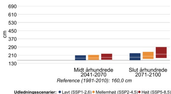
Figur 13 Højden af 20- (venstre) og 100-års (højre) stormflodhændelser for Skagerrakkyst sydlige i fremtidsperioderne 2041-2070 og 2071-2100 under forskellige udledningsscenarier. Den grå linje viser referenceværdien for nutiden (1981-2010).
