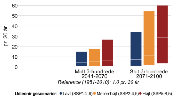
Figur 10 Ændring i middelvandstand (venstre) og hyppigheden af stormflod for Vestkysten ud for Limfjorden i fremtidsperioderne 2041-2070 og 2071-2100 under forskellige udledningsscenarioer. Den grå linje viser referenceværdien for
