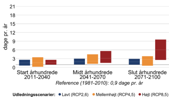
Figur 3 Ændring af gennemsnitstemperatur og antallet af hedebløgedage hen over året mellem 1981-2010 og fremtidsperioderne 2011-2040, 2041-2070 og 2071-2100 under forskellige udledningsscenarier i Thisted Kommune.
