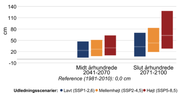
Figur 10 Ændring i middelvandstand (venstre) og hyppigheden af stormflod for Vestkysten ud for Limfjorden i fremtidsperioderne 2041-2070 og 2071-2100 under forskellige udledningsscenarioer. Den grå linje viser referenceværdien for
