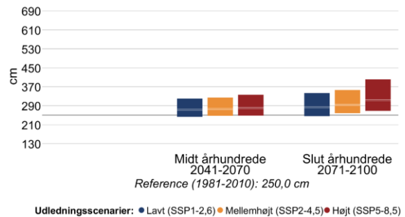
Figur 11 Højden af 20- (venstre) og 100-års (højre) stormflodhændelser for Vestkysten ud for Limfjorden i fremtidsperioderne 2041-2070 og 2071-2100 under forskellige udledningsscenarier. Den grå linje viser referenceværdien for nutiden (1981-2010).
