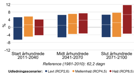
Figur 8 Procentvis ændring af tørre dage om sommeren (jun-aug) mellem 1981-2010 og fremtidsperioderne 2011-2040, 2041-2070 og 2071-2100 under forskellige udledningsscenarier i Thisted Kommune. Til venstre antallet af tørre dage med mindre end 1 mm nedbør, til højre længden af den længste sammenhængende tørre periode.
