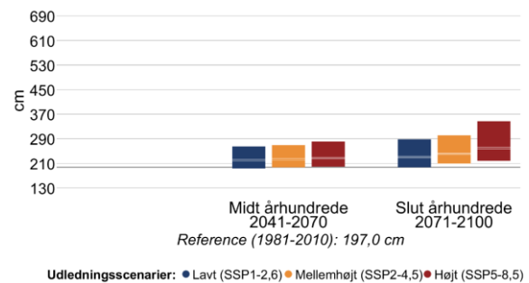
Figur 15 Højden af 20- (venstre) og 100-års (højre) stormflodhændelser for Limfjorden ved Lemvig i fremtidsperioderne 2041-2070 og 2071-2100 under forskellige udledningsscenarier. Den grå linje viser referenceværdien for nutiden (1981-2010).
