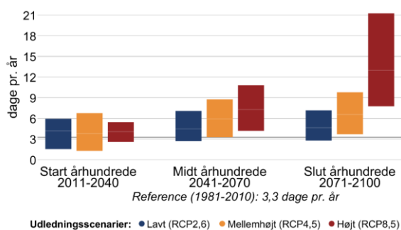
Figur 3 Ændring af gennemsnitstemperatur og antallet af hedebløgedage hen over året mellem 1981-2010 og fremtidsperioderne 2011-2040, 2041-2070 og 2071-2100 under forskellige udledningsscenarier i Tårnby Kommune.
