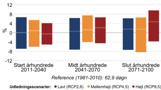
Figur 8 Procentvis ændring af tørre dage om sommeren (jun-aug) mellem 1981-2010 og fremtidsperioderne 2011-2040, 2041-2070 og 2071-2100 under forskellige udledningsscenarier i Tårnby Kommune. Til venstre antallet af tørre dage med mindre end 1 mm nedbør, til højre længden af den længste sammenhængende tørre periode.
