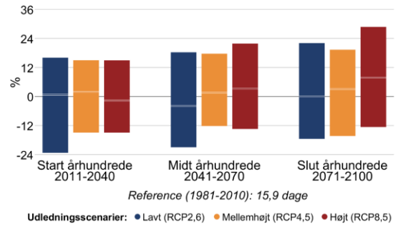
Figur 8 Procentvis ændring af tørre dage om sommeren (jun-aug) mellem 1981-2010 og fremtidsperioderne 2011-2040, 2041-2070 og 2071-2100 under forskellige udledningsscenarier i Tårnby Kommune. Til venstre antallet af tørre dage med mindre end 1 mm nedbør, til højre længden af den længste sammenhængende tørre periode.
