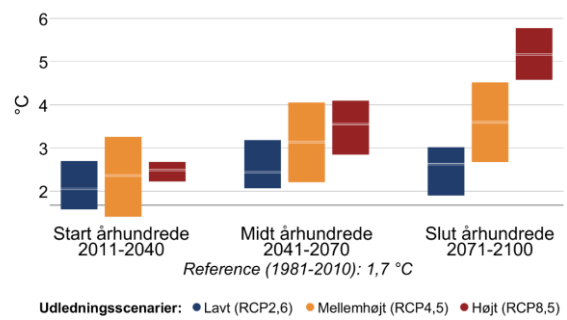
Figur 4 Gennemsnitstemperatur for sommer (jun-aug) og vinter (dec-feb) i fremtidsperioderne 2011-2040, 2041-2070 og 2071-2100 under forskellige udledningsscenarier i Tårnby Kommune. Den grå linje viser referenceværdien for nutiden (1981-2010).
