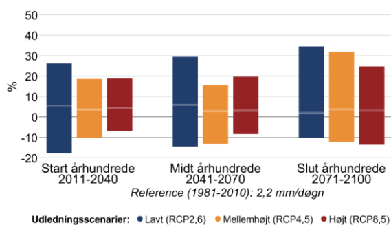
Figur 6 Procentvis ændring af middelnedbør mellem 1981-2010 og fremtidsperioderne 2011-2040, 2041-2070 og 2071-2100 under forskellige udledningsscenarier i Tårnby Kommune. Til venstre sommer (jun-aug), til højre vinter (dec-feb).
