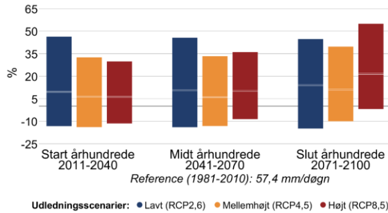
Figur 7 Procentvis ændring af ekstremnedbør hen over året mellem 1981-2010 og fremtidsperioderne 2011-2040, 2041-2070 og 2071-2100 under forskellige udledningsscenarier i Tårnby Kommune. Til venstre 10-årshændelsen for døgnnedbør, til højre frekvensen af skybrud.
