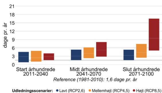
Figur 3 Ændring af gennemsnitstemperatur og antallet af hedebølgedage hen over året mellem 1981-2010 og fremtidsperioderne 2011-2040, 2041-2070 og 2071-2100 under forskellige udledningsscenarier i Svendborg Kommune.
