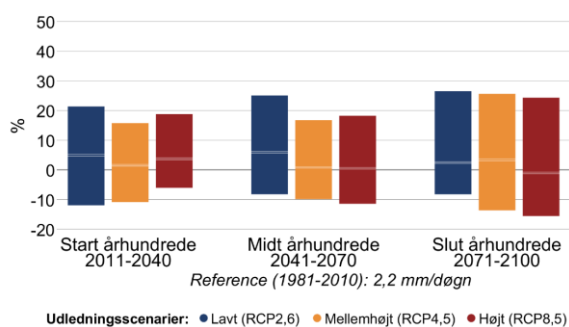
Figur 6 Procentvis ændring af middelnedbør mellem 1981-2010 og fremtidsperioderne 2011-2040, 2041-2070 og 2071-2100 under forskellige udledningsscenarier i Svendborg Kommune. Til venstre sommer (jun-aug), til højre vinter (dec-feb).
