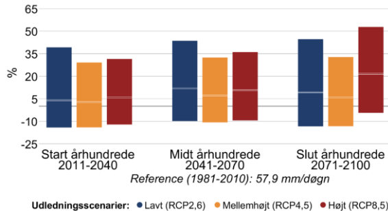
Figur 7 Procentvis ændring af ekstremnedbør hen over året mellem 1981-2010 og fremtidsperioderne 2011-2040, 2041-2070 og 2071-2100 under forskellige udledningsscenarier i Svendborg Kommune. Til venstre 10-årshændelsen for døgnnedbør, til højre frekvensen af skybrud.
