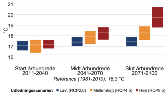
Figur 4 Gennemsnitstemperatur for sommer (jun-aug) og vinter (dec-feb) i fremtidsperioderne 2011-2040, 2041-2070 og 2071-2100 under forskellige udledningsscenarier i Svendborg Kommune. Den grå linje viser referenceværdien for nutiden (1981-2010).
