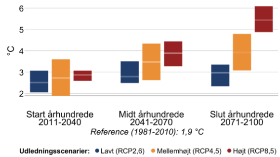
Figur 4 Gennemsnitstemperatur for sommer (jun-aug) og vinter (dec-feb) i fremtidsperioderne 2011-2040, 2041-2070 og 2071-2100 under forskellige udledningsscenarier i Svendborg Kommune. Den grå linje viser referenceværdien for nutiden (1981-2010).
