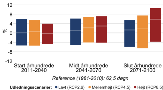
Figur 8 Procentvis ændring af tørre dage om sommeren (jun-aug) mellem 1981-2010 og fremtidsperioderne 2011-2040, 2041-2070 og 2071-2100 under forskellige udledningsscenarier i Svendborg Kommune. Til venstre antallet af tørre dage med mindre end 1 mm nedbør, til højre længden af den længste sammenhængende tørre periode.
