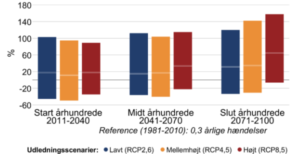
Figur 7 Procentvis ændring af ekstremnedbør hen over året mellem 1981-2010 og fremtidsperioderne 2011-2040, 2041-2070 og 2071-2100 under forskellige udledningsscenarier i Svendborg Kommune. Til venstre 10-årshændelsen for døgnnedbør, til højre frekvensen af skybrud.
