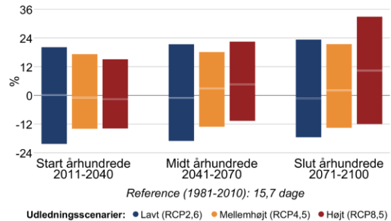
Figur 8 Procentvis ændring af tørre dage om sommeren (jun-aug) mellem 1981-2010 og fremtidsperioderne 2011-2040, 2041-2070 og 2071-2100 under forskellige udledningsscenarier i Svendborg Kommune. Til venstre antallet af tørre dage med mindre end 1 mm nedbør, til højre længden af den længste sammenhængende tørre periode.
