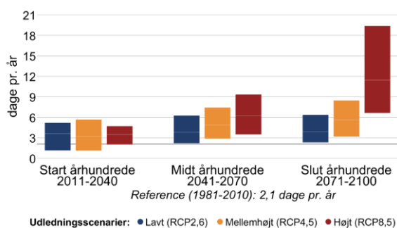
Figur 3 Ændring af gennemsnitstemperatur og antallet af hedebølgedage hen over året mellem 1981-2010 og fremtidsperioderne 2011-2040, 2041-2070 og 2071-2100 under forskellige udledningsscenarier i Stevns Kommune.
