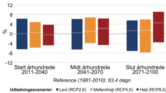
Figur 8 Procentvis ændring af tørre dage om sommeren (jun-aug) mellem 1981-2010 og fremtidsperioderne 2011-2040, 2041-2070 og 2071-2100 under forskellige udledningsscenarier i Stevns Kommune. Til venstre antallet af tørre dage med mindre end 1 mm nedbør, til højre længden af den længste sammenhængende tørre periode.
