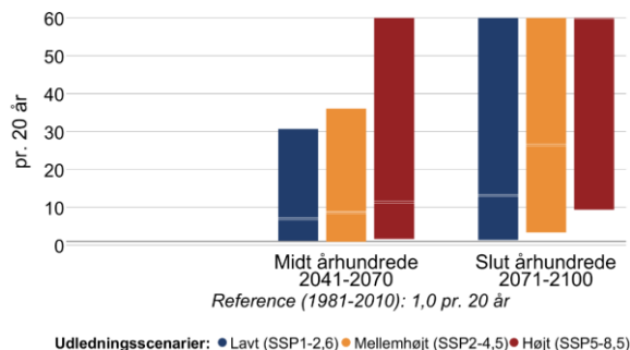
Figur 10 Ændring i middelvandstand (venstre) og hyppigheden af stormflod for Faxe Bugt i fremtidsperioderne 2041-2070 og 2071-2100 under forskellige udledningsscenarioer. Den grå linje viser referenceværdien for nutiden (1981-2010). En stormflod defineres her som en forhøjet vandstand, der statistisk set kun forekommer én gang hvert 20. år i perioden 1981-2010. Bemærk også at denne indikator kappes ved 60 stormfloder per 20 år.
