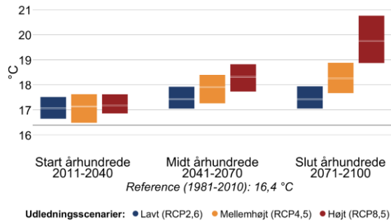
Figur 4 Gennemsnitstemperatur for sommer (jun-aug) og vinter (dec-feb) i fremtidsperioderne 2011-2040, 2041-2070 og 2071-2100 under forskellige udledningsscenarier i Stevns Kommune. Den grå linje viser referenceværdien for nutiden (1981-2010).
