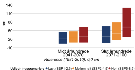
Figur 10 Ændring i middelvandstand (venstre) og hyppigheden af stormflod for Faxe Bugt i fremtidsperioderne 2041-2070 og 2071-2100 under forskellige udledningsscenarioer. Den grå linje viser referenceværdien for nutiden (1981-2010). En stormflod defineres her som en forhøjet vandstand, der statistisk set kun forekommer én gang hvert 20. år i perioden 1981-2010. Bemærk også at denne indikator kappes ved 60 stormfloder per 20 år.
