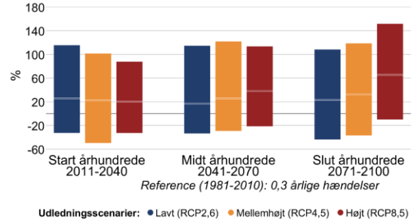
Figur 7 Procentvis ændring af ekstremnedbør hen over året mellem 1981-2010 og fremtidsperioderne 2011-2040, 2041-2070 og 2071-2100 under forskellige udledningsscenarier i Stevns Kommune. Til venstre 10-årshændelsen for døgnnedbør, til højre frekvensen af skybrud.
