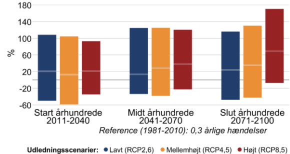
Figur 7 Procentvis ændring af ekstremnedbør hen over året mellem 1981-2010 og fremtidsperioderne 2011-2040, 2041-2070 og 2071-2100 under forskellige udledningsscenarier i Slagelse Kommune. Til venstre 10-årshændelsen for døgnnedbør, til højre frekvensen af skybrud.
