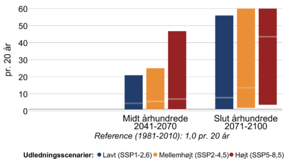
Figur 12 Ændring i middelvandstand (venstre) og hyppigheden af stormflod for Storebælt nordøst i fremtidsperioderne 2041-2070 og 2071-2100 under forskellige udledningsscenarier. Den grå linje viser referenceværdien for nutiden (1981-2010). En stormflod defineres her som en forhøjet vandstand, der statistisk set kun forekommer én gang hvert 20. år i perioden 1981-2010. Bemærk også at denne indikator kappes ved 60 stormfloder per 20 år.
