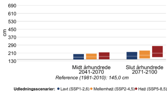
Figur 13 Højden af 20- (venstre) og 100-års (højre) stormflodhændelser for Storebælt nordøst i fremtidsperioderne 2041-2070 og 2071-2100 under forskellige udledningsscenarier. Den grå linje viser referenceværdien for nutiden (1981-2010).
