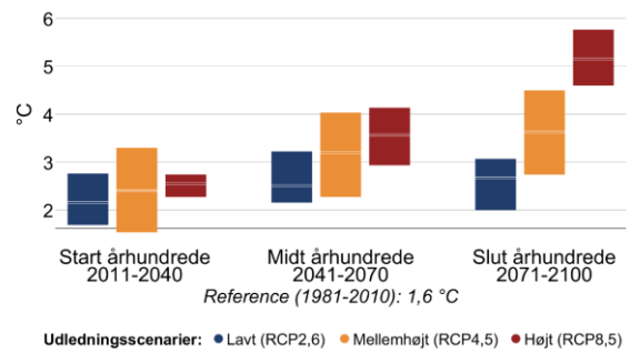
Figur 4 Gennemsnitstemperatur for sommer (jun-aug) og vinter (dec-feb) i fremtidsperioderne 2011-2040, 2041-2070 og 2071-2100 under forskellige udledningsscenarier i Slagelse Kommune. Den grå linje viser referenceværdien for nutiden (1981-2010).
