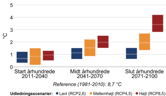
Figur 3 Ændring af gennemsnitstemperatur og antallet af hedebølgedage hen over året mellem 1981-2010 og fremtidsperioderne 2011-2040, 2041-2070 og 2071-2100 under forskellige udledningsscenarier i Slagelse Kommune.
