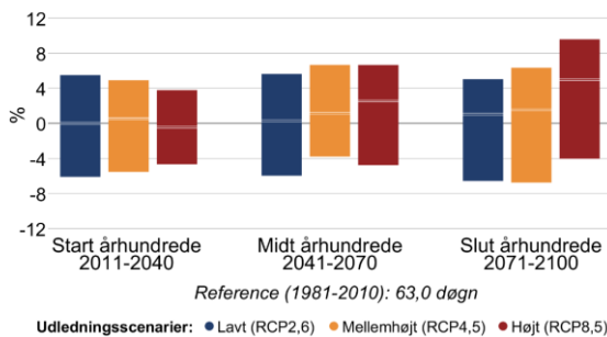
Figur 8 Procentvis ændring af tørre dage om sommeren (jun-aug) mellem 1981-2010 og fremtidsperioderne 2011-2040, 2041-2070 og 2071-2100 under forskellige udledningsscenarier i Slagelse Kommune. Til venstre antallet af tørre dage med mindre end 1 mm nedbør, til højre længden af den længste sammenhængende tørre periode.
