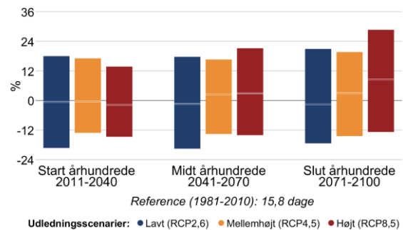
Figur 8 Procentvis ændring af tørre dage om sommeren (jun-aug) mellem 1981-2010 og fremtidsperioderne 2011-2040, 2041-2070 og 2071-2100 under forskellige udledningsscenarier i Slagelse Kommune. Til venstre antallet af tørre dage med mindre end 1 mm nedbør, til højre længden af den længste sammenhængende tørre periode.
