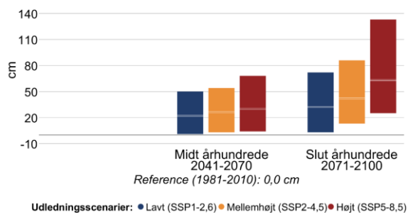
Figur 12 Ændring i middelvandstand (venstre) og hyppigheden af stormflod for Storebælt nordøst i fremtidsperioderne 2041-2070 og 2071-2100 under forskellige udledningsscenarier. Den grå linje viser referenceværdien for nutiden (1981-2010). En stormflod defineres her som en forhøjet vandstand, der statistisk set kun forekommer én gang hvert 20. år i perioden 1981-2010. Bemærk også at denne indikator kappes ved 60 stormfloder per 20 år.
