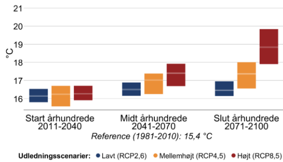
Figur 4 Gennemsnitstemperatur for sommer (jun-aug) og vinter (dec-feb) i fremtidsperioderne 2011-2040, 2041-2070 og 2071-2100 under forskellige udledningsscenarier i Skanderborg Kommune. Den grå linje viser referenceværdien for nutiden (1981-2010).
