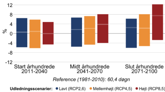
Figur 8 Procentvis ændring af tørre dage om sommeren (jun-aug) mellem 1981-2010 og fremtidsperioderne 2011-2040, 2041-2070 og 2071-2100 under forskellige udledningsscenarier i Skanderborg Kommune. Til venstre antallet af tørre dage med mindre end 1 mm nedbør, til højre længden af den længste sammenhængende tørre periode.
