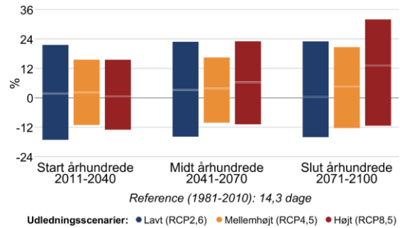
Figur 8 Procentvis ændring af tørre dage om sommeren (jun-aug) mellem 1981-2010 og fremtidsperioderne 2011-2040, 2041-2070 og 2071-2100 under forskellige udledningsscenarier i Skanderborg Kommune. Til venstre antallet af tørre dage med mindre end 1 mm nedbør, til højre længden af den længste sammenhængende tørre periode.
