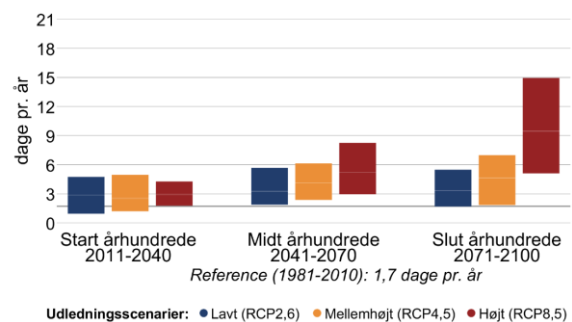
Figur 3 Ændring af gennemsnitstemperatur og antallet af hedebølgedage hen over året mellem 1981-2010 og fremtidsperioderne 2011-2040, 2041-2070 og 2071-2100 under forskellige udledningsscenarier i Skanderborg Kommune.
