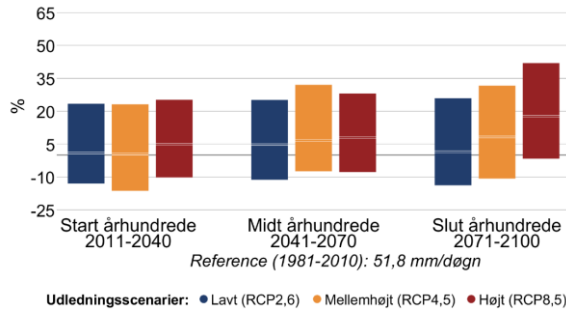
Figur 7 Procentvis ændring af ekstremnedbør hen over året mellem 1981-2010 og fremtidsperioderne 2011-2040, 2041-2070 og 2071-2100 under forskellige udledningsscenarier i Skanderborg Kommune. Til venstre 10-årshændelsen for døgnnedbør, til højre frekvensen af skybrud.
