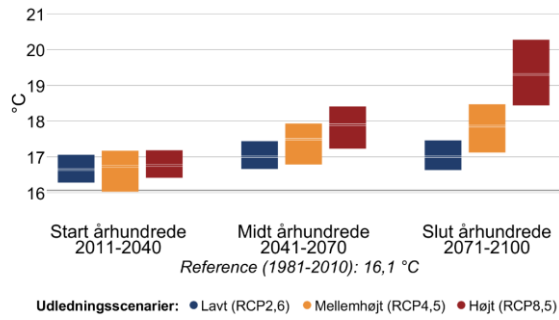
Figur 4 Gennemsnitstemperatur for sommer (jun-aug) og vinter (dec-feb) i fremtidsperioderne 2011-2040, 2041-2070 og 2071-2100 under forskellige udledningsscenarier i Samsø Kommune. Den grå linje viser referenceværdien for nutiden (1981-2010).
