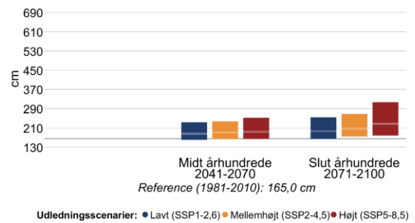
Figur 15 Højden af 20- (venstre) og 100-års (højre) stormflodhændelser for Sejerø Bugt i fremtidsperioderne 2041-2070 og 2071-2100 under forskellige udledningsscenarioer. Den grå linje viser referenceværdien for nutiden (1981-2010).
