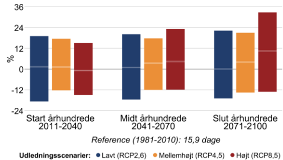
Figur 8 Procentvis ændring af tørre dage om sommeren (jun-aug) mellem 1981-2010 og fremtidsperioderne 2011-2040, 2041-2070 og 2071-2100 under forskellige udledningsscenarier i Samsø Kommune. Til venstre antallet af tørre dage med mindre end 1 mm nedbør, til højre længden af den længste sammenhængende tørre periode.
