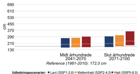
Figur 13 Højden af 20- (venstre) og 100-års (højre) stormflodhændelser for Storebælt nordvest og Odense Fjord i fremtidsperioderne 2041-2070 og 2071-2100 under forskellige udledningsscenarier. Den grå linje viser referenceværdien for nutiden (1981-2010).
