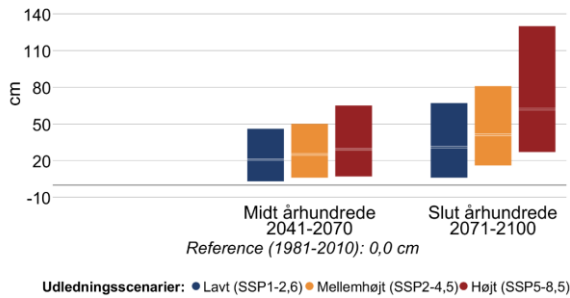
Figur 14 Ændring i middelvandstand (venstre) og hyppigheden af stormflod for Sejerø Bugt i fremtidsperioderne 2041-2070 og 2071-2100 under forskellige udledningsscenarioer. Den grå linje viser referenceværdien for nutiden (1981-2010). En stormflod defineres her som en forhøjet vandstand, der statistisk set kun forekommer én gang hvert 20. år i perioden 1981-2010. Bemærk også at denne indikator kappes ved 60 stormfloder per 20 år.
