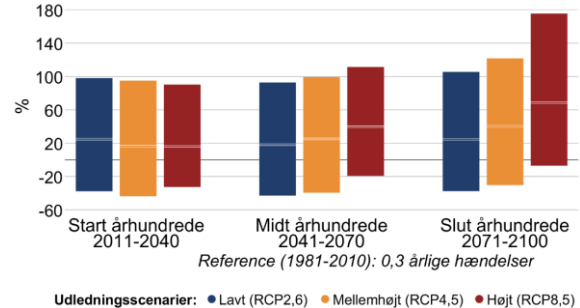
Figur 7 Procentvis ændring af ekstremnedbør hen over året mellem 1981-2010 og fremtidsperioderne 2011-2040, 2041-2070 og 2071-2100 under forskellige udledningsscenarier i Samsø Kommune. Til venstre 10-årshændelsen for døgnnedbør, til højre frekvensen af skybrud.
