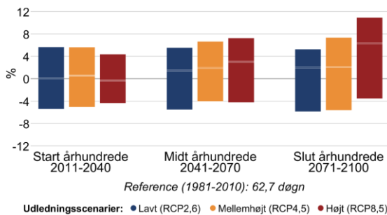
Figur 8 Procentvis ændring af tørre dage om sommeren (jun-aug) mellem 1981-2010 og fremtidsperioderne 2011-2040, 2041-2070 og 2071-2100 under forskellige udledningsscenarier i Samsø Kommune. Til venstre antallet af tørre dage med mindre end 1 mm nedbør, til højre længden af den længste sammenhængende tørre periode.
