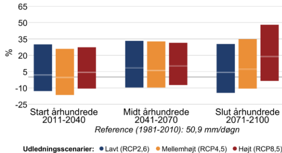
Figur 7 Procentvis ændring af ekstremnedbør hen over året mellem 1981-2010 og fremtidsperioderne 2011-2040, 2041-2070 og 2071-2100 under forskellige udledningsscenarier i Samsø Kommune. Til venstre 10-årshændelsen for døgnnedbør, til højre frekvensen af skybrud.
