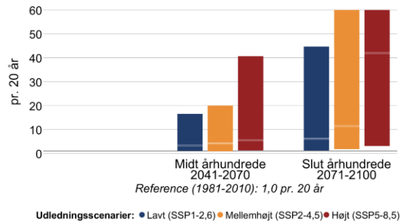
Figur 14 Ændring i middelvandstand (venstre) og hyppigheden af stormflod for Sejerø Bugt i fremtidsperioderne 2041-2070 og 2071-2100 under forskellige udledningsscenarioer. Den grå linje viser referenceværdien for nutiden (1981-2010). En stormflod defineres her som en forhøjet vandstand, der statistisk set kun forekommer én gang hvert 20. år i perioden 1981-2010. Bemærk også at denne indikator kappes ved 60 stormfloder per 20 år.
