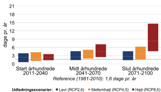
Figur 3 Ændring af gennemsnitstemperatur og antallet af hedebølgedage hen over året mellem 1981-2010 og fremtidsperioderne 2011-2040, 2041-2070 og 2071-2100 under forskellige udledningsscenarier i Samsø Kommune.
