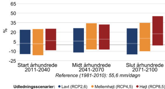
Figur 7 Procentvis ændring af ekstremnedbør hen over året mellem 1981-2010 og fremtidsperioderne 2011-2040, 2041-2070 og 2071-2100 under forskellige udledningsscenarier i Randers Kommune. Til venstre 10-årshændelsen for døgnnedbør, til højre frekvensen af skybrud.
