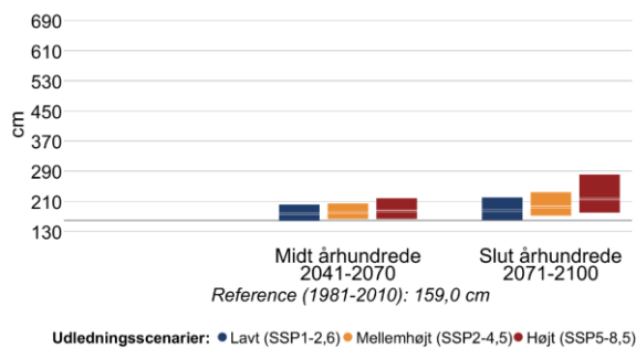
Figur 13 Højden af 20- (venstre) og 100-års (højre) stormflodhændelser for Randers Fjord og Mariager Fjord i fremtidsperioderne 2041-2070 og 2071-2100 under forskellige udledningsscenarier. Den grå linje viser referenceværdien for nutiden (1981-2010).
