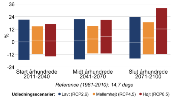
Figur 8 Procentvis ændring af tørre dage om sommeren (jun-aug) mellem 1981-2010 og fremtidsperioderne 2011-2040, 2041-2070 og 2071-2100 under forskellige udledningsscenarier i Randers Kommune. Til venstre antallet af tørre dage med mindre end 1 mm nedbør, til højre længden af den længste sammenhængende tørre periode.
