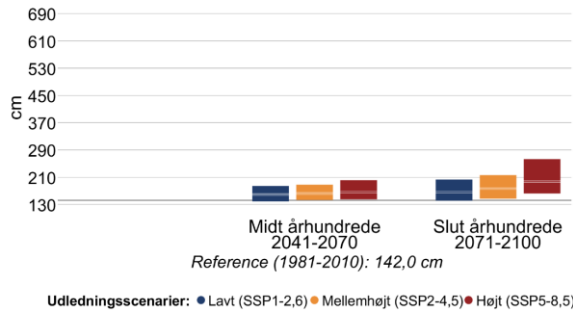
Figur 11 Højden af 20- (venstre) og 100-års (højre) stormflodhændelser for Ålborg Bugt i fremtidsperioderne 2041-2070 og 2071-2100 under forskellige udledningsscenarier. Den grå linje viser referenceværdien for nutiden (1981-2010).
