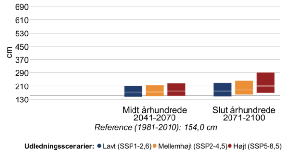
Figur 11 Højden af 20- (venstre) og 100-års (højre) stormflodhændelser for Ålborg Bugt i fremtidsperioderne 2041-2070 og 2071-2100 under forskellige udledningsscenarier. Den grå linje viser referenceværdien for nutiden (1981-2010).
