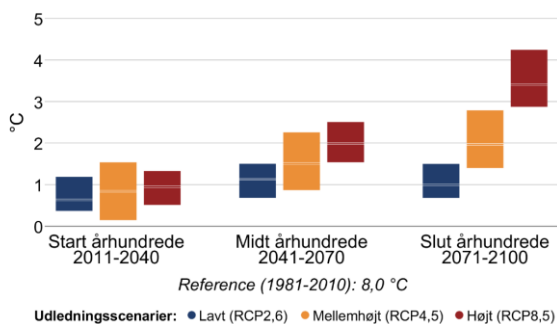
Figur 3 Ændring af gennemsnitstemperatur og antallet af hedebølgedage hen over året mellem 1981-2010 og fremtidsperioderne 2011-2040, 2041-2070 og 2071-2100 under forskellige udledningsscenarier i Randers Kommune.
