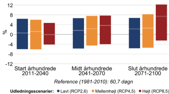
Figur 8 Procentvis ændring af tørre dage om sommeren (jun-aug) mellem 1981-2010 og fremtidsperioderne 2011-2040, 2041-2070 og 2071-2100 under forskellige udledningsscenarier i Randers Kommune. Til venstre antallet af tørre dage med mindre end 1 mm nedbør, til højre længden af den længste sammenhængende tørre periode.
