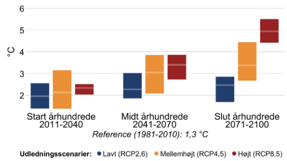
Figur 4 Gennemsnitstemperatur for sommer (jun-aug) og vinter (dec-feb) i fremtidsperioderne 2011-2040, 2041-2070 og 2071-2100 under forskellige udledningsscenarier i Randers Kommune. Den grå linje viser referenceværdien for nutiden (1981-2010).
