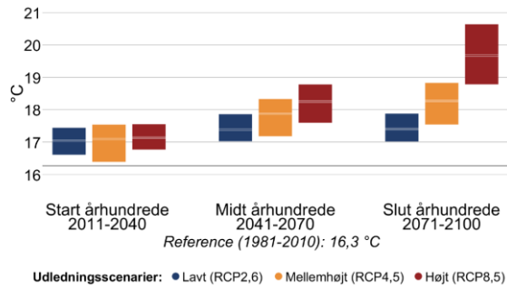
Figur 4 Gennemsnitstemperatur for sommer (jun-aug) og vinter (dec-feb) i fremtidsperioderne 2011-2040, 2041-2070 og 2071-2100 under forskellige udledningsscenarier i Odsherred Kommune. Den grå linje viser referenceværdien for nutiden (1981-2010).
