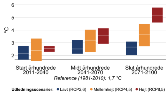
Figur 4 Gennemsnitstemperatur for sommer (jun-aug) og vinter (dec-feb) i fremtidsperioderne 2011-2040, 2041-2070 og 2071-2100 under forskellige udledningsscenarier i Odsherred Kommune. Den grå linje viser referenceværdien for nutiden (1981-2010).
