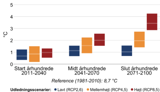
Figur 3 Ændring af gennemsnitstemperatur og antallet af hedebølgedage hen over året mellem 1981-2010 og fremtidsperioderne 2011-2040, 2041-2070 og 2071-2100 under forskellige udledningsscenarier i Odsherred Kommune.
