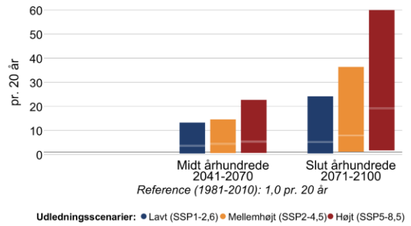
Figur 14 Ændring i middelvandstand (venstre) og hyppigheden af stormflod for Isefjord i fremtidsperioderne 2041-2070 og 2071-2100 under forskellige udledningsscenarier. Den grå linje viser referenceværdien for nutiden (1981-2010). En stormflod defineres her som en forhøjet vandstand, der statistisk set kun forekommer én gang hvert 20. år i perioden 1981-2010. Bemærk også at denne indikator kappes ved 60 stormfloder per 20 år.
