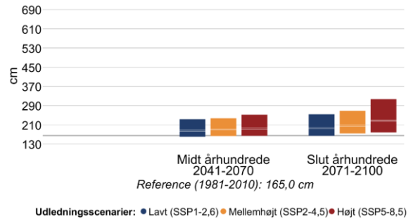
Figur 11 Højden af 20- (venstre) og 100-års (højre) stormflodhændelser for Sejerø Bugt i fremtidsperioderne 2041-2070 og 2071-2100 under forskellige udledningsscenarier. Den grå linje viser referenceværdien for nutiden (1981-2010).
