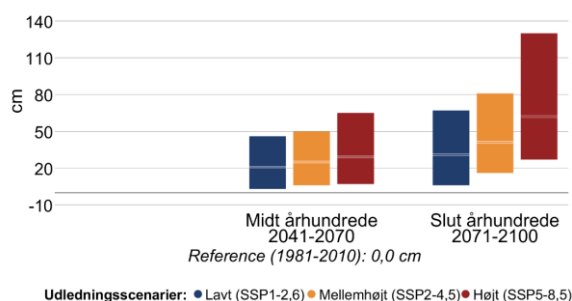
Figur 10 Ændring i middelvandstand (venstre) og hyppigheden af stormflod for Sejerø Bugt i fremtidsperioderne 2041-2070 og 2071-2100 under forskellige udledningsscenerier. Den grå linje viser referenceværdien for nutiden (1981-2010). En stormflod defineres her som en forhøjet vandstand, der statistisk set kun forekommer én gang hvert 20. år i perioden 1981-2010. Bemærk også at denne indikator kappes ved 60 stormfloder per 20 år.
