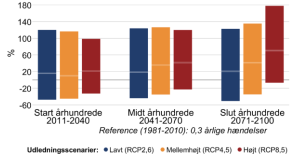
Figur 7 Procentvis ændring af ekstremnedbør hen over året mellem 1981-2010 og fremtidsperioderne 2011-2040, 2041-2070 og 2071-2100 under forskellige udledningsscenarier i Odsherred Kommune. Til venstre 10-årshændelsen for døgnnedbør, til højre frekvensen af skybrud.
