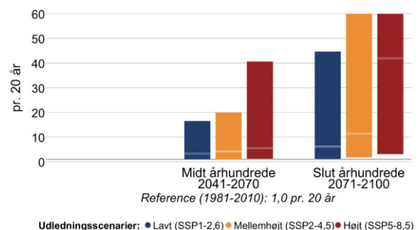
Figur 10 Ændring i middelvandstand (venstre) og hyppigheden af stormflod for Sejerø Bugt i fremtidsperioderne 2041-2070 og 2071-2100 under forskellige udledningsscenerier. Den grå linje viser referenceværdien for nutiden (1981-2010). En stormflod defineres her som en forhøjet vandstand, der statistisk set kun forekommer én gang hvert 20. år i perioden 1981-2010. Bemærk også at denne indikator kappes ved 60 stormfloder per 20 år.
