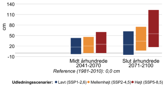
Figur 14 Ændring i middelvandstand (venstre) og hyppigheden af stormflod for Isefjord i fremtidsperioderne 2041-2070 og 2071-2100 under forskellige udledningsscenarier. Den grå linje viser referenceværdien for nutiden (1981-2010). En stormflod defineres her som en forhøjet vandstand, der statistisk set kun forekommer én gang hvert 20. år i perioden 1981-2010. Bemærk også at denne indikator kappes ved 60 stormfloder per 20 år.
