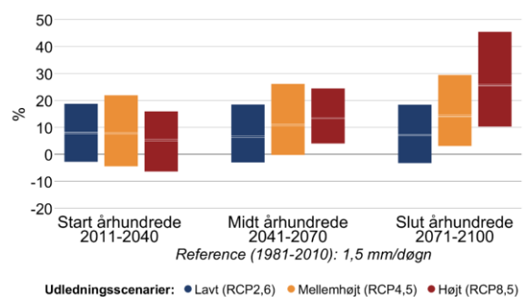
Figur 6 Procentvis ændring af middelnedbør mellem 1981-2010 og fremtidsperioderne 2011-2040, 2041-2070 og 2071-2100 under forskellige udledningsscenarier i Odsherred Kommune. Til venstre sommer (jun-aug), til højre vinter (dec-feb).
