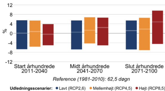
Figur 8 Procentvis ændring af tørre dage om sommeren (jun-aug) mellem 1981-2010 og fremtidsperioderne 2011-2040, 2041-2070 og 2071-2100 under forskellige udledningsscenarier i Odsherred Kommune. Til venstre antallet af tørre dage med mindre end 1 mm nedbør, til højre længden af den længste sammenhængende tørre periode.
