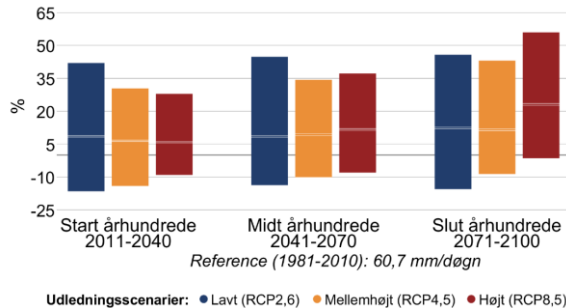
Figur 7 Procentvis ændring af ekstremnedbør hen over året mellem 1981-2010 og fremtidsperioderne 2011-2040, 2041-2070 og 2071-2100 under forskellige udledningsscenarier i Odsherred Kommune. Til venstre 10-årshændelsen for døgnnedbør, til højre frekvensen af skybrud.
