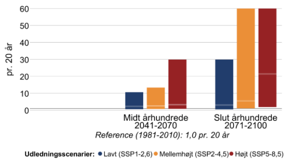
Figur 12 Ændring i middelvandstand (venstre) og hyppigheden af stormflod for Nordsjællands kyst i fremtidsperioderne 2041-2070 og 2071-2100 under forskellige udledningsscenarier. Den grå linje viser referenceværdien for nutiden (1981-2010). En stormflod defineres her som en forhøjet vandstand, der statistisk set kun forekommer én gang hvert 20. år i perioden 1981-2010. Bemærk også at denne indikator kappes ved 60 stormfloder per 20 år.
