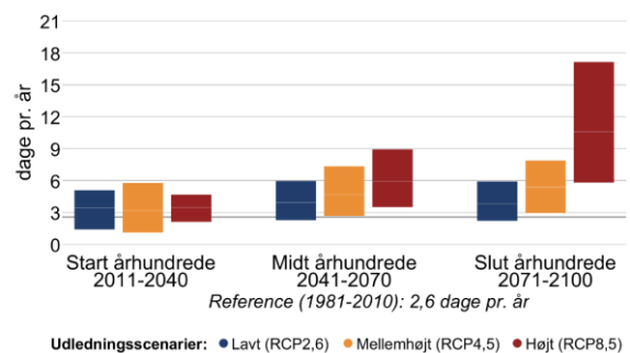
Figur 3 Ændring af gennemsnitstemperatur og antallet af hedebølgedage hen over året mellem 1981-2010 og fremtidsperioderne 2011-2040, 2041-2070 og 2071-2100 under forskellige udledningsscenarier i Odsherred Kommune.
