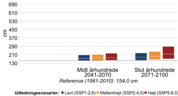
Figur 11 Højden af 20- (venstre) og 100-års (højre) stormflodhændelser for Sejerø Bugt i fremtidsperioderne 2041-2070 og 2071-2100 under forskellige udledningsscenarier. Den grå linje viser referenceværdien for nutiden (1981-2010).
