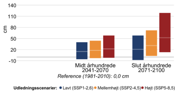
Figur 12 Ændring i middelvandstand (venstre) og hyppigheden af stormflod for Nordsjællands kyst i fremtidsperioderne 2041-2070 og 2071-2100 under forskellige udledningsscenarier. Den grå linje viser referenceværdien for nutiden (1981-2010). En stormflod defineres her som en forhøjet vandstand, der statistisk set kun forekommer én gang hvert 20. år i perioden 1981-2010. Bemærk også at denne indikator kappes ved 60 stormfloder per 20 år.
