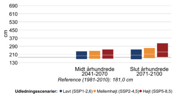
Figur 13 Højden af 20- (venstre) og 100-års (højre) stormflodhændelser for Nordsjællands kyst i fremtidsperioderne 2041-2070 og 2071-2100 under forskellige udledningsscenarier. Den grå linje viser referenceværdien for nutiden (1981-2010).
