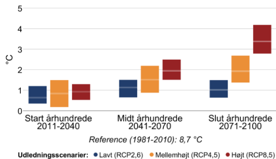
Figur 3 Ændring af gennemsnitstemperatur og antallet af hedebølgedage hen over året mellem 1981-2010 og fremtidsperioderne 2011-2040, 2041-2070 og 2071-2100 under forskellige udledningsscenarier i Odense Kommune.
