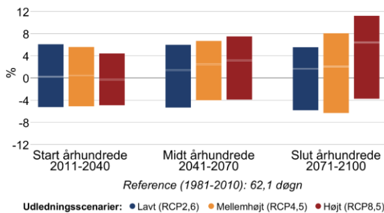
Figur 8 Procentvis ændring af tørre dage om sommeren (jun-aug) mellem 1981-2010 og fremtidsperioderne 2011-2040, 2041-2070 og 2071-2100 under forskellige udledningsscenarier i Odense Kommune. Til venstre antallet af tørre dage med mindre end 1 mm nedbør, til højre længden af den længste sammenhængende tørre periode.
