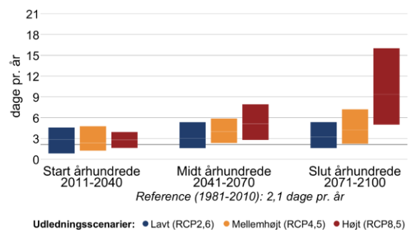
Figur 3 Ændring af gennemsnitstemperatur og antallet af hedebølgedage hen over året mellem 1981-2010 og fremtidsperioderne 2011-2040, 2041-2070 og 2071-2100 under forskellige udledningsscenarier i Odense Kommune.
