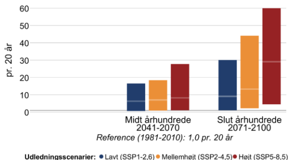
Figur 10 Ændring i middelvandstand (venstre) og hyppigheden af stormflod for Storebælt nordvest og Odense Fjord i fremtidsperioderne 2041-2070 og 2071-2100 under forskellige udledningsscenarier. Den grå linje viser referenceværdien for nutiden (1981-2010). En stormflod defineres her som en forhøjet vandstand, der statistisk set kun forekommer én gang hvert 20. år i perioden 1981-2010. Bemærk også at denne indikator kappes ved 60 stormfloder per 20 år.
