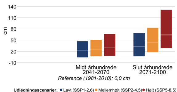
Figur 10 Ændring i middelvandstand (venstre) og hyppigheden af stormflod for Storebælt nordvest og Odense Fjord i fremtidsperioderne 2041-2070 og 2071-2100 under forskellige udledningsscenarier. Den grå linje viser referenceværdien for nutiden (1981-2010). En stormflod defineres her som en forhøjet vandstand, der statistisk set kun forekommer én gang hvert 20. år i perioden 1981-2010. Bemærk også at denne indikator kappes ved 60 stormfloder per 20 år.
