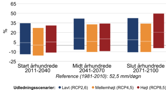
Figur 7 Procentvis ændring af ekstremnedbør hen over året mellem 1981-2010 og fremtidsperioderne 2011-2040, 2041-2070 og 2071-2100 under forskellige udledningsscenarier i Odense Kommune. Til venstre 10-årshændelsen for døgnnedbør, til højre frekvensen af skybrud.
