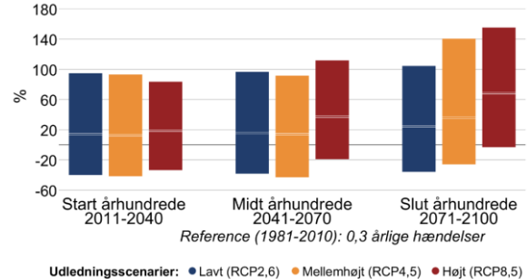
Figur 7 Procentvis ændring af ekstremnedbør hen over året mellem 1981-2010 og fremtidsperioderne 2011-2040, 2041-2070 og 2071-2100 under forskellige udledningsscenarier i Odense Kommune. Til venstre 10-årshændelsen for døgnnedbør, til højre frekvensen af skybrud.
