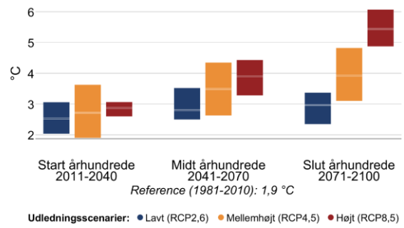
Figur 4 Gennemsnitstemperatur for sommer (jun-aug) og vinter (dec-feb) i fremtidsperioderne 2011-2040, 2041-2070 og 2071-2100 under forskellige udledningsscenarier i Odense Kommune. Den grå linje viser referenceværdien for nutiden (1981-2010).
