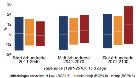
Figur 8 Procentvis ændring af tørre dage om sommeren (jun-aug) mellem 1981-2010 og fremtidsperioderne 2011-2040, 2041-2070 og 2071-2100 under forskellige udledningsscenarier i Odense Kommune. Til venstre antallet af tørre dage med mindre end 1 mm nedbør, til højre længden af den længste sammenhængende tørre periode.
