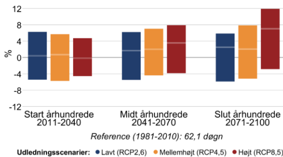
Figur 8 Procentvis ændring af tørre dage om sommeren (jun-aug) mellem 1981-2010 og fremtidsperioderne 2011-2040, 2041-2070 og 2071-2100 under forskellige udledningsscenarier i Odder Kommune. Til venstre antallet af tørre dage med mindre end 1 mm nedbør, til højre længden af den længste sammenhængende tørre periode.
