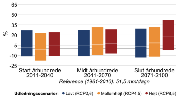
Figur 7 Procentvis ændring af ekstremnedbør hen over året mellem 1981-2010 og fremtidsperioderne 2011-2040, 2041-2070 og 2071-2100 under forskellige udledningsscenarier i Odder Kommune. Til venstre 10-årshændelsen for døgnnedbør, til højre frekvensen af skybrud.
