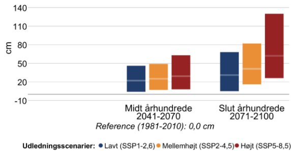
Figur 12 Ændring i middelvandstand (venstre) og hyppigheden af stormflod for Lillebælt nordlig i fremtidsperioderne 2041-2070 og 2071-2100 under forskellige udledningsscenarier. Den grå linje viser referenceværdien for nutiden (1981-2010). En stormflod defineres her som en forhøjet vandstand, der statistisk set kun forekommer én gang hvert 20. år i perioden 1981-2010. Bemærk også at denne indikator kappes ved 60 stormfloder per 20 år.
