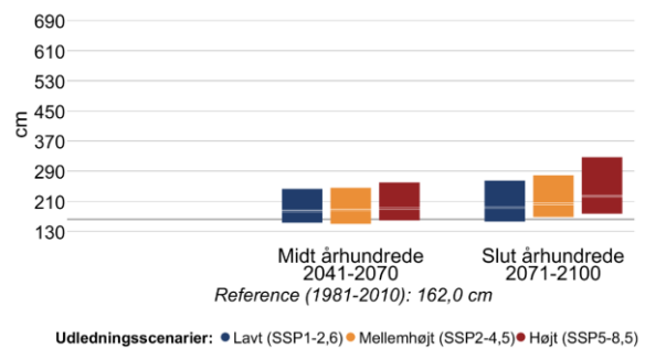
Figur 13 Højden af 20- (venstre) og 100-års (højre) stormflodhændelser for Lillebælt nordlig i fremtidsperioderne 2041-2070 og 2071-2100 under forskellige udledningsscenarier. Den grå linje viser referenceværdien for nutiden (1981-2010).
