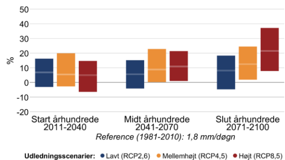
Figur 6 Procentvis ændring af middelnedbør mellem 1981-2010 og fremtidsperioderne 2011-2040, 2041-2070 og 2071-2100 under forskellige udledningsscenarier i Odder Kommune. Til venstre sommer (jun-aug), til højre vinter (dec-feb).
