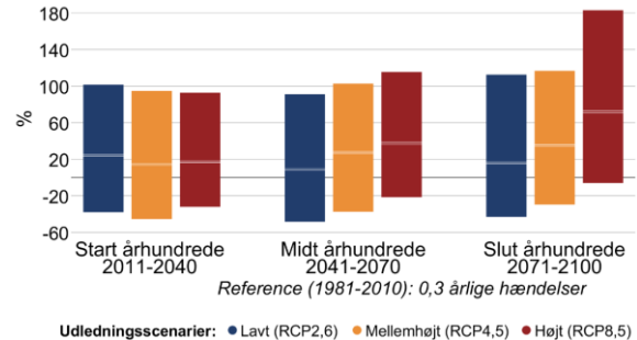
Figur 7 Procentvis ændring af ekstremnedbør hen over året mellem 1981-2010 og fremtidsperioderne 2011-2040, 2041-2070 og 2071-2100 under forskellige udledningsscenarier i Odder Kommune. Til venstre 10-årshændelsen for døgnnedbør, til højre frekvensen af skybrud.
