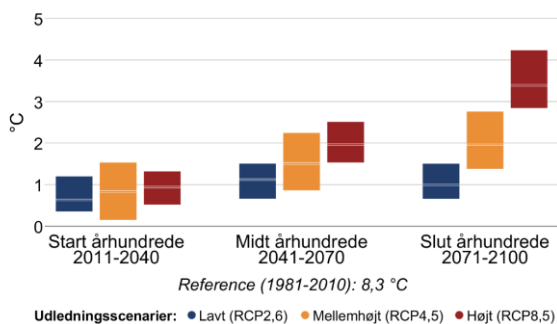
Figur 3 Ændring af gennemsnitstemperatur og antallet af hedebølgedage hen over året mellem 1981-2010 og fremtidsperioderne 2011-2040, 2041-2070 og 2071-2100 under forskellige udledningsscenarier i Odder Kommune.
