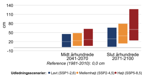
Figur 10 Ændring i middelvandstand (venstre) og hyppigheden af stormflod for Århus Bugt i fremtidsperioderne 2041-2070 og 2071-2100 under forskellige udledningsscenarioer. Den grå linje viser referenceværdien for nutiden (1981-2010). En stormflod defineres her som en forhøjet vandstand, der statistisk set kun forekommer én gang hvert 20. år i perioden 1981-2010. Bemærk også at denne indikator kappes ved 60 stormfloder per 20 år.
