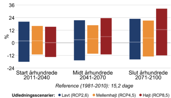
Figur 8 Procentvis ændring af tørre dage om sommeren (jun-aug) mellem 1981-2010 og fremtidsperioderne 2011-2040, 2041-2070 og 2071-2100 under forskellige udledningsscenarier i Odder Kommune. Til venstre antallet af tørre dage med mindre end 1 mm nedbør, til højre længden af den længste sammenhængende tørre periode.
