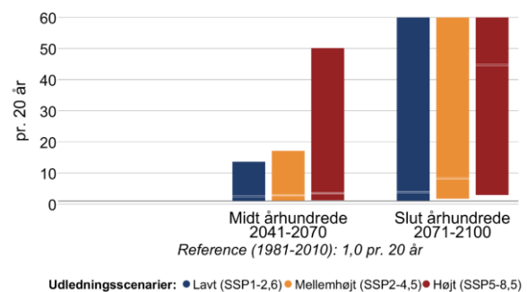
Figur 10 Ændring i middelvandstand (venstre) og hyppigheden af stormflod for Århus Bugt i fremtidsperioderne 2041-2070 og 2071-2100 under forskellige udledningsscenarioer. Den grå linje viser referenceværdien for nutiden (1981-2010). En stormflod defineres her som en forhøjet vandstand, der statistisk set kun forekommer én gang hvert 20. år i perioden 1981-2010. Bemærk også at denne indikator kappes ved 60 stormfloder per 20 år.
