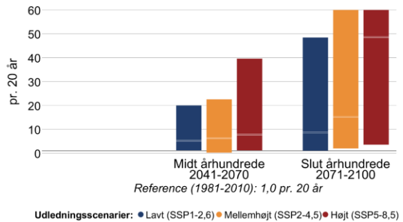
Figur 12 Ændring i middelvandstand (venstre) og hyppigheden af stormflod for Lillebælt nordlig i fremtidsperioderne 2041-2070 og 2071-2100 under forskellige udledningsscenarier. Den grå linje viser referenceværdien for nutiden (1981-2010). En stormflod defineres her som en forhøjet vandstand, der statistisk set kun forekommer én gang hvert 20. år i perioden 1981-2010. Bemærk også at denne indikator kappes ved 60 stormfloder per 20 år.
