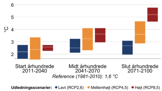
Figur 4 Gennemsnitstemperatur for sommer (jun-aug) og vinter (dec-feb) i fremtidsperioderne 2011-2040, 2041-2070 og 2071-2100 under forskellige udledningsscenarier i Odder Kommune. Den grå linje viser referenceværdien for nutiden (1981-2010).
