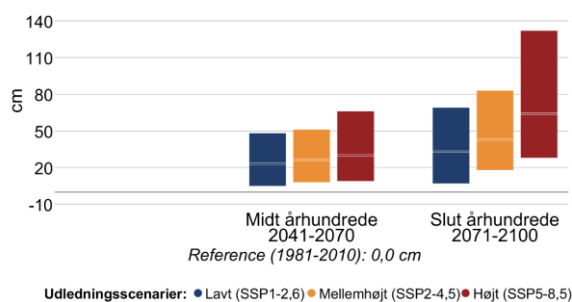
Figur 10 Ændring i middelvandstand (venstre) og hyppigheden af stormflod for Storebælt Sydvest i fremtidsperioderne 2041-2070 og 2071-2100 under forskellige udledningsscenarioer. Den grå linje viser referenceværdien for nutiden (1981-2010). En
