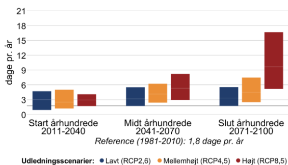
Figur 3 Ændring af gennemsnitstemperatur og antallet af hedebølgedage hen over året mellem 1981-2010 og fremtidsperioderne 2011-2040, 2041-2070 og 2071-2100 under forskellige udledningsscenarier i Nyborg Kommune.
