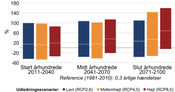
Figur 7 Procentvis ændring af ekstremnedbør hen over året mellem 1981-2010 og fremtidsperioderne 2011-2040, 2041-2070 og 2071-2100 under forskellige udledningsscenarier i Nyborg Kommune. Til venstre 10-årshændelsen for døgnet nedbør, til højre frekvensen af skybrud.
