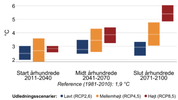
Figur 4 Gennemsnitstemperatur for sommer (jun-aug) og vinter (dec-feb) i fremtidsperioderne 2011-2040, 2041-2070 og 2071-2100 under forskellige udledningsscenarier i Nyborg Kommune. Den grå linje viser referenceværdien for nutiden (1981-2010).
