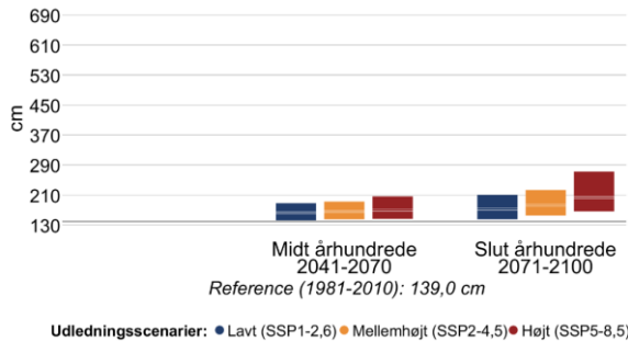
Figur 11 Højden af 20- (venstre) og 100-års (højre) stormflodhændelser for Storebælt Sydvest i fremtidsperioderne 2041-2070 og 2071-2100 under forskellige udledningsscenarier. Den grå linje viser referenceværdien for nutiden (1981-2010).
