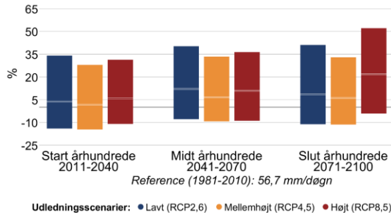
Figur 7 Procentvis ændring af ekstremnedbør hen over året mellem 1981-2010 og fremtidsperioderne 2011-2040, 2041-2070 og 2071-2100 under forskellige udledningsscenarier i Nyborg Kommune. Til venstre 10-årshændelsen for døgnet nedbør, til højre frekvensen af skybrud.
