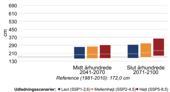
Figur 13 Højden af 20- (venstre) og 100-års (højre) stormflodhændelser for Storebælt nordvest og Odense Fjord i fremtidsperioderne 2041-2070 og 2071-2100 under forskellige udledningsscenarier. Den grå linje viser referenceværdien for nutiden (1981-2010).
