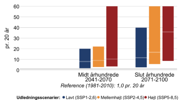
Figur 10 Ændring i middelvandstand (venstre) og hyppigheden af stormflod for Storebælt Sydvest i fremtidsperioderne 2041-2070 og 2071-2100 under forskellige udledningsscenarioer. Den grå linje viser referenceværdien for nutiden (1981-2010). En
