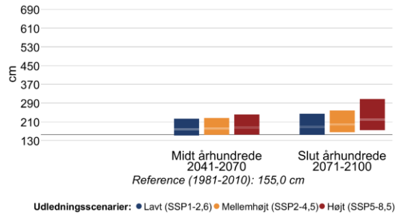
Figur 11 Højden af 20- (venstre) og 100-års (højre) stormflodhændelser for Storebælt Sydvest i fremtidsperioderne 2041-2070 og 2071-2100 under forskellige udledningsscenarier. Den grå linje viser referenceværdien for nutiden (1981-2010).
