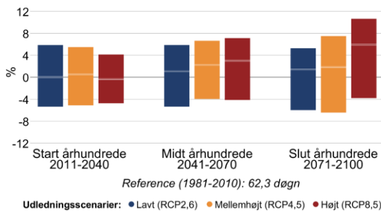
Figur 8 Procentvis ændring af tørre dage om sommeren (jun-aug) mellem 1981-2010 og fremtidsperioderne 2011-2040, 2041-2070 og 2071-2100 under forskellige udledningsscenarier i Nyborg Kommune. Til venstre antallet af tørre dage med mindre end 1 mm nedbør, til højre længden af den længste sammenhængende tørre periode.
