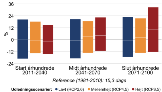
Figur 8 Procentvis ændring af tørre dage om sommeren (jun-aug) mellem 1981-2010 og fremtidsperioderne 2011-2040, 2041-2070 og 2071-2100 under forskellige udledningsscenarier i Nyborg Kommune. Til venstre antallet af tørre dage med mindre end 1 mm nedbør, til højre længden af den længste sammenhængende tørre periode.
