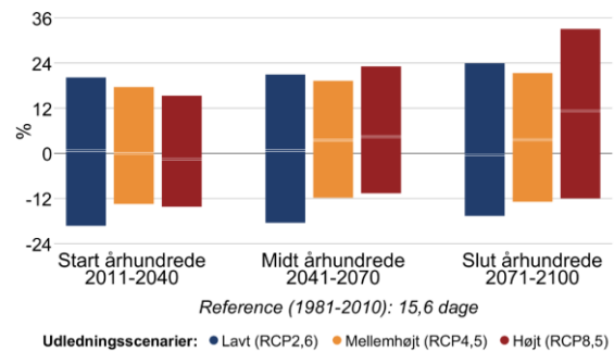
Figur 8 Procentvis ændring af tørre dage om sommeren (jun-aug) mellem 1981-2010 og fremtidsperioderne 2011-2040, 2041-2070 og 2071-2100 under forskellige udledningsscenarier i Nordfyns Kommune. Til venstre antallet af tørre dage med mindre end 1 mm nedbør, til højre længden af den længste sammenhængende tørre periode.
