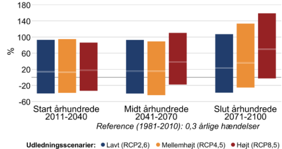
Figur 7 Procentvis ændring af ekstremnedbør hen over året mellem 1981-2010 og fremtidsperioderne 2011-2040, 2041-2070 og 2071-2100 under forskellige udledningsscenarier i Nordfyns Kommune. Til venstre 10-årshændelsen for døgnnedbør, til højre frekvensen af skybrud.
