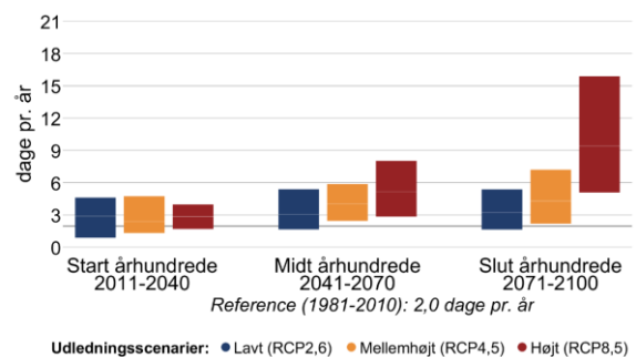
Figur 3 Ændring af gennemsnitstemperatur og antallet af hedebølgedage hen over året mellem 1981-2010 og fremtidsperioderne 2011-2040, 2041-2070 og 2071-2100 under forskellige udledningsscenarier i Nordfyns Kommune.
