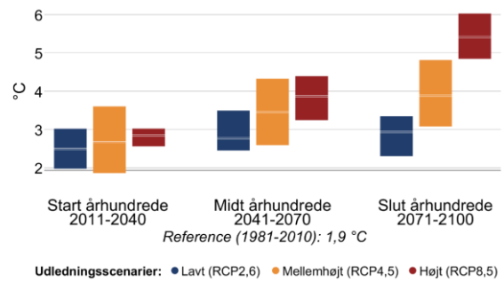
Figur 4 Gennemsnitstemperatur for sommer (jun-aug) og vinter (dec-feb) i fremtidsperioderne 2011-2040, 2041-2070 og 2071-2100 under forskellige udledningsscenarier i Nordfyns Kommune. Den grå linje viser referenceværdien for nutiden (1981-2010).
