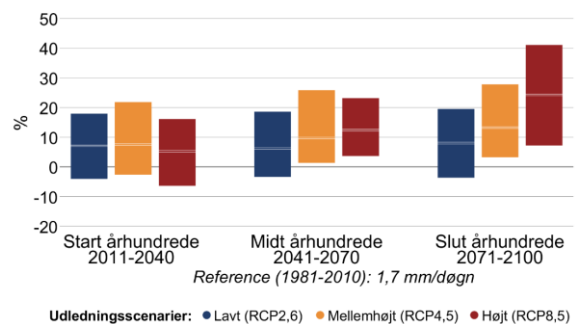
Figur 6 Procentvis ændring af middelnedbør mellem 1981-2010 og fremtidsperioderne 2011-2040, 2041-2070 og 2071-2100 under forskellige udledningsscenarier i Nordfyns Kommune. Til venstre sommer (jun-aug), til højre vinter (dec-feb).
