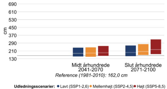
Figur 11 Højden af 20- (venstre) og 100-års (højre) stormflodhændelser for Lillebælt nordlig i fremtidsperioderne 2041-2070 og 2071-2100 under forskellige udledningsscenarioer. Den grå linje viser referenceværdien for nutiden (1981-2010).
