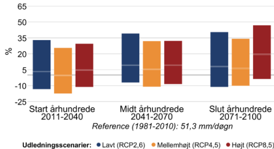
Figur 7 Procentvis ændring af ekstremnedbør hen over året mellem 1981-2010 og fremtidsperioderne 2011-2040, 2041-2070 og 2071-2100 under forskellige udledningsscenarier i Nordfyns Kommune. Til venstre 10-årshændelsen for døgnnedbør, til højre frekvensen af skybrud.
