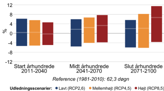
Figur 8 Procentvis ændring af tørre dage om sommeren (jun-aug) mellem 1981-2010 og fremtidsperioderne 2011-2040, 2041-2070 og 2071-2100 under forskellige udledningsscenarier i Nordfyns Kommune. Til venstre antallet af tørre dage med mindre end 1 mm nedbør, til højre længden af den længste sammenhængende tørre periode.
