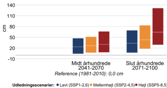
Figur 12 Ændring i middelvandstand (venstre) og hyppigheden af stormflod for Storebælt nordvest og Odense Fjord i fremtidsperioderne 2041-2070 og 2071-2100 under forskellige udledningsscenarioer. Den grå linje viser referenceværdien for nutiden (1981-2010). En stormflod defineres her som en forhøjet vandstand, der statistisk set kun forekommer én gang hvert 20. år i perioden 1981-2010. Bemærk også at denne indikator kappes ved 60 stormfloder per 20 år.
