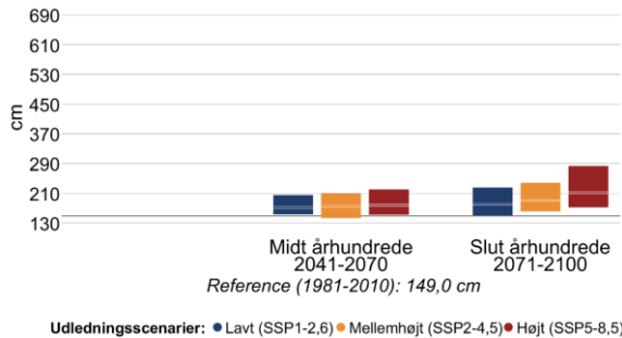
Figur 11 Højden af 20- (venstre) og 100-års (højre) stormflodhændelser for Lillebælt nordlig i fremtidsperioderne 2041-2070 og 2071-2100 under forskellige udledningsscenarioer. Den grå linje viser referenceværdien for nutiden (1981-2010).
