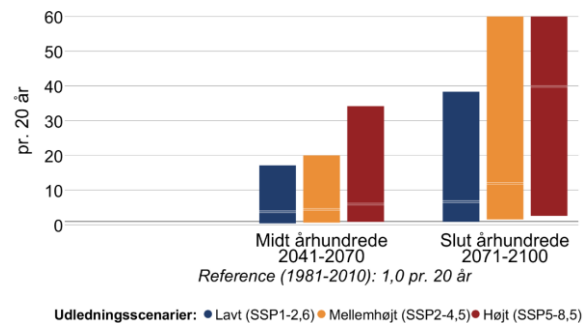
Figur 10 Ændring i middelvandstand (venstre) og hyppigheden af stormflod for Smålandsfarvandet i fremtidsperioderne 2041-2070 og 2071-2100 under forskellige udledningsscenarioer. Den grå linje viser referenceværdien for nutiden (1981-2010). En stormflod defineres her som en forhøjet vandstand, der statistisk set kun forekommer én gang hvert 20. år i perioden 1981-2010. Bemærk også at denne indikator kappes ved 60 stormfloder per 20 år.
