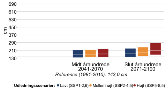
Figur 11 Højden af 20- (venstre) og 100-års (højre) stormflodhændelser for Smålandsfarvandet i fremtidsperioderne 2041-2070 og 2071-2100 under forskellige udledningsscenarier. Den grå linje viser referenceværdien for nutiden (1981-2010).
