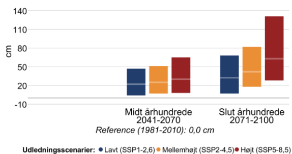
Figur 10 Ændring i middelvandstand (venstre) og hyppigheden af stormflod for Smålandsfarvandet i fremtidsperioderne 2041-2070 og 2071-2100 under forskellige udledningsscenarioer. Den grå linje viser referenceværdien for nutiden (1981-2010). En stormflod defineres her som en forhøjet vandstand, der statistisk set kun forekommer én gang hvert 20. år i perioden 1981-2010. Bemærk også at denne indikator kappes ved 60 stormfloder per 20 år.
