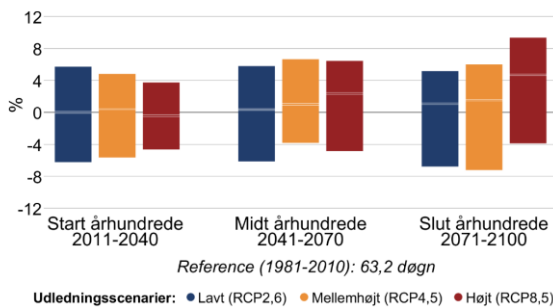
Figur 8 Procentvis ændring af tørre dage om sommeren (jun-aug) mellem 1981-2010 og fremtidsperioderne 2011-2040, 2041-2070 og 2071-2100 under forskellige udledningsscenarier i Næstved Kommune. Til venstre antallet af tørre dage med mindre end 1 mm nedbør, til højre længden af den længste sammenhængende tørre periode.
