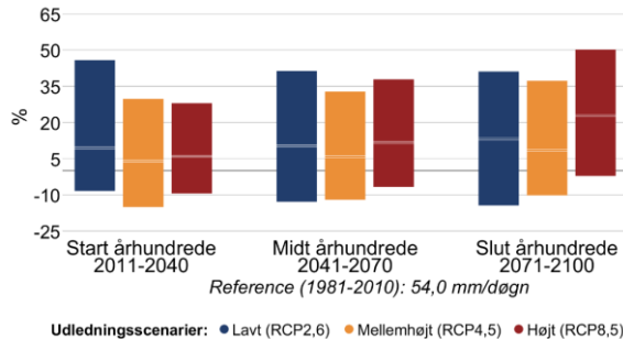
Figur 7 Procentvis ændring af ekstremnedbør hen over året mellem 1981-2010 og fremtidsperioderne 2011-2040, 2041-2070 og 2071-2100 under forskellige udledningsscenarier i Næstved Kommune. Til venstre 10-årshændelsen for døgnet nedbør, til højre frekvensen af skybrud.
