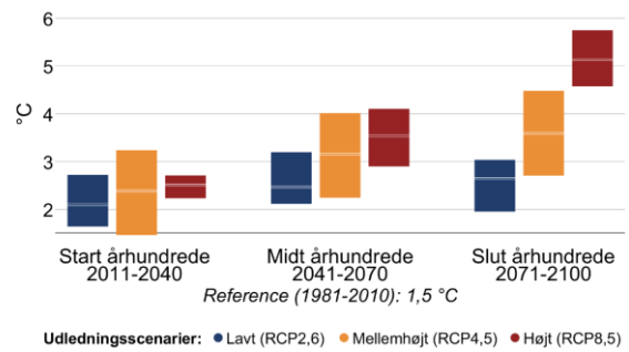
Figur 4 Gennemsnitstemperatur for sommer (jun-aug) og vinter (dec-feb) i fremtidsperioderne 2011-2040, 2041-2070 og 2071-2100 under forskellige udledningsscenarier i Næstved Kommune. Den grå linje viser referenceværdien for nutiden (1981-2010).
