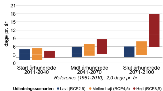
Figur 3 Ændring af gennemsnitstemperatur og antallet af hedebløddage hen over året mellem 1981-2010 og fremtidsperioderne 2011-2040, 2041-2070 og 2071-2100 under forskellige udledningsscenarier i Næstved Kommune.
