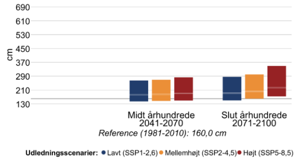
Figur 11 Højden af 20- (venstre) og 100-års (højre) stormflodhændelser for Smålandsfarvandet i fremtidsperioderne 2041-2070 og 2071-2100 under forskellige udledningsscenarier. Den grå linje viser referenceværdien for nutiden (1981-2010).
