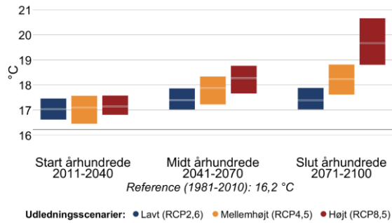
Figur 4 Gennemsnitstemperatur for sommer (jun-aug) og vinter (dec-feb) i fremtidsperioderne 2011-2040, 2041-2070 og 2071-2100 under forskellige udledningsscenarier i Næstved Kommune. Den grå linje viser referenceværdien for nutiden (1981-2010).
