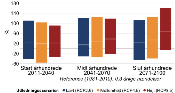
Figur 7 Procentvis ændring af ekstremnedbør hen over året mellem 1981-2010 og fremtidsperioderne 2011-2040, 2041-2070 og 2071-2100 under forskellige udledningsscenarier i Næstved Kommune. Til venstre 10-årshændelsen for døgnet nedbør, til højre frekvensen af skybrud.
