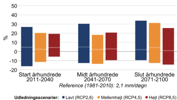
Figur 6 Procentvis ændring af middelnedbør mellem 1981-2010 og fremtidsperioderne 2011-2040, 2041-2070 og 2071-2100 under forskellige udledningsscenarier i Næstved Kommune. Til venstre sommer (jun-aug), til højre vinter (dec-feb).
