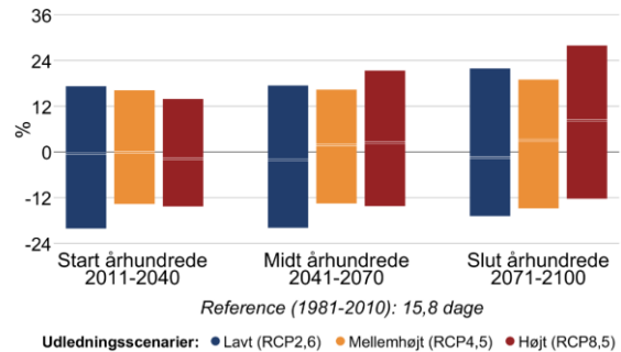
Figur 8 Procentvis ændring af tørre dage om sommeren (jun-aug) mellem 1981-2010 og fremtidsperioderne 2011-2040, 2041-2070 og 2071-2100 under forskellige udledningsscenarier i Næstved Kommune. Til venstre antallet af tørre dage med mindre end 1 mm nedbør, til højre længden af den længste sammenhængende tørre periode.
