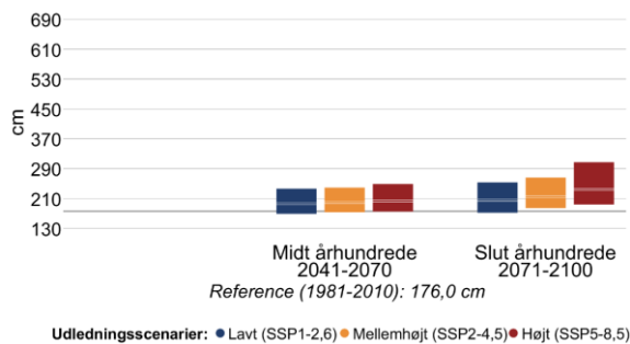
Figur 15 Højden af 20- (venstre) og 100-års (højre) stormflodhændelser for Limfjorden ved Thisted i fremtidsperioderne 2041-2070 og 2071-2100 under forskellige udledningsscenarier. Den grå linje viser referenceværdien for nutiden (1981-2010).
