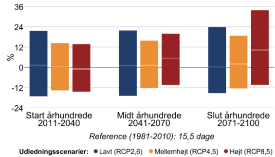
Figur 8 Procentvis ændring af tørre dage om sommeren (jun-aug) mellem 1981-2010 og fremtidsperioderne 2011-2040, 2041-2070 og 2071-2100 under forskellige udledningsscenarier i Morsø Kommune. Til venstre antallet af tørre dage med mindre end 1 mm nedbør, til højre længden af den længste sammenhængende tørre periode.
