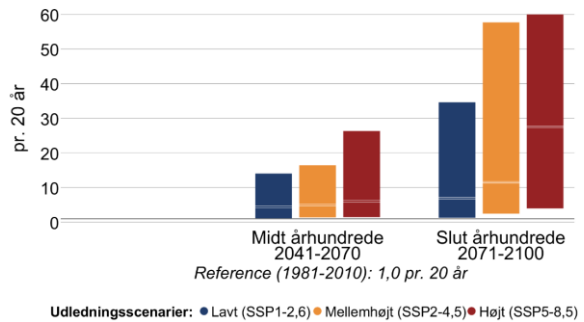
Figur 12 Ændring i middelvandstand (venstre) og hyppigheden af stormflod for Limfjorden ved Lemvig i fremtidsperioderne 2041-2070 og 2071-2100 under forskellige udledningsscenarier. Den grå linje viser referenceværdien for nutiden (1981-2010). En stormflod defineres her som en forhøjet vandstand, der statistisk set kun forekommer én gang hvert 20. år i perioden 1981-2010. Bemærk også at denne indikator kappes ved 60 stormfloder per 20 år.
