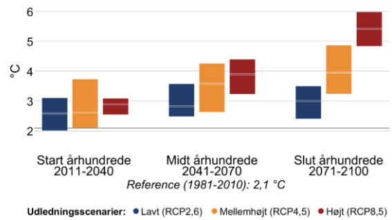
Figur 4 Gennemsnitstemperatur for sommer (jun-aug) og vinter (dec-feb) i fremtidsperioderne 2011-2040, 2041-2070 og 2071-2100 under forskellige udledningsscenarier i Morsø Kommune. Den grå linje viser referenceværdien for nutiden (1981-2010).
