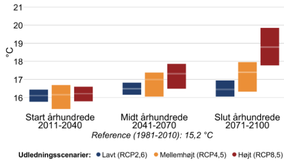
Figur 4 Gennemsnitstemperatur for sommer (jun-aug) og vinter (dec-feb) i fremtidsperioderne 2011-2040, 2041-2070 og 2071-2100 under forskellige udledningsscenarier i Morsø Kommune. Den grå linje viser referenceværdien for nutiden (1981-2010).
