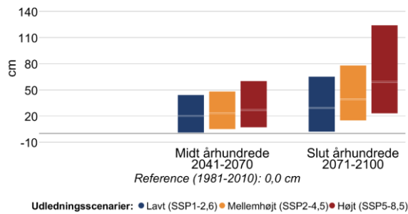
Figur 14 Ændring i middelvandstand (venstre) og hyppigheden af stormflod for Limfjorden ved Thisted i fremtidsperioderne 2041-2070 og 2071-2100 under forskellige udledningsscenarier. Den grå linje viser referenceværdien for nutiden (1981-2010). En stormflod defineres her som en forhøjet vandstand, der statistisk set kun forekommer én gang hvert 20. år i perioden 1981-2010. Bemærk også at denne indikator kappes ved 60 stormfloder per 20 år.
