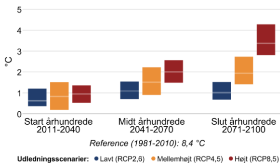
Figur 3 Ændring af gennemsnitstemperatur og antallet af hedebløgedage hen over året mellem 1981-2010 og fremtidsperioderne 2011-2040, 2041-2070 og 2071-2100 under forskellige udledningsscenarier i Morsø Kommune.
