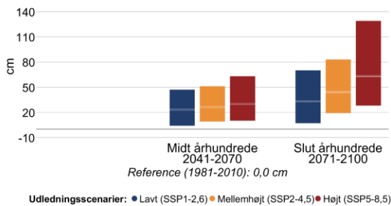
Figur 12 Ændring i middelvandstand (venstre) og hyppigheden af stormflod for Limfjorden ved Lemvig i fremtidsperioderne 2041-2070 og 2071-2100 under forskellige udledningsscenarier. Den grå linje viser referenceværdien for nutiden (1981-2010). En stormflod defineres her som en forhøjet vandstand, der statistisk set kun forekommer én gang hvert 20. år i perioden 1981-2010. Bemærk også at denne indikator kappes ved 60 stormfloder per 20 år.
