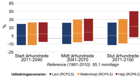
Figur 7 Procentvis ændring af ekstremnedbør hen over året mellem 1981-2010 og fremtidsperioderne 2011-2040, 2041-2070 og 2071-2100 under forskellige udledningsscenarier i Morsø Kommune. Til venstre 10-årshændelsen for døgnnedbør, til højre frekvensen af skybrud.
