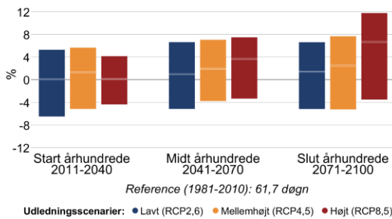
Figur 8 Procentvis ændring af tørre dage om sommeren (jun-aug) mellem 1981-2010 og fremtidsperioderne 2011-2040, 2041-2070 og 2071-2100 under forskellige udledningsscenarier i Morsø Kommune. Til venstre antallet af tørre dage med mindre end 1 mm nedbør, til højre længden af den længste sammenhængende tørre periode.
