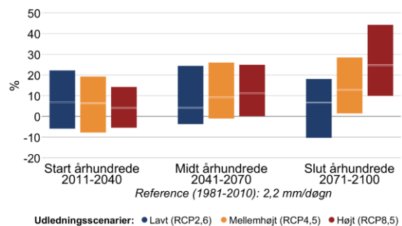
Figur 6 Procentvis ændring af middelnedbør mellem 1981-2010 og fremtidsperioderne 2011-2040, 2041-2070 og 2071-2100 under forskellige udledningsscenarier i Morsø Kommune. Til venstre sommer (jun-aug), til højre vinter (dec-feb).
