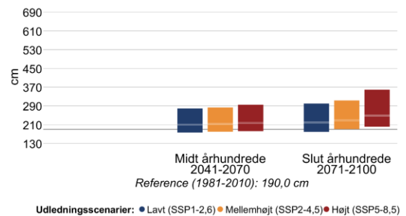
Figur 15 Højden af 20- (venstre) og 100-års (højre) stormflodhændelser for Limfjorden ved Thisted i fremtidsperioderne 2041-2070 og 2071-2100 under forskellige udledningsscenarier. Den grå linje viser referenceværdien for nutiden (1981-2010).
