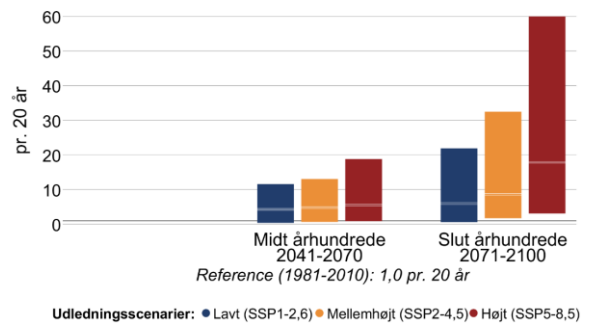
Figur 14 Ændring i middelvandstand (venstre) og hyppigheden af stormflod for Limfjorden ved Thisted i fremtidsperioderne 2041-2070 og 2071-2100 under forskellige udledningsscenarier. Den grå linje viser referenceværdien for nutiden (1981-2010). En stormflod defineres her som en forhøjet vandstand, der statistisk set kun forekommer én gang hvert 20. år i perioden 1981-2010. Bemærk også at denne indikator kappes ved 60 stormfloder per 20 år.
