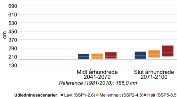
Figur 13 Højden af 20- (venstre) og 100-års (højre) stormflodhændelser for Limfjorden ved Lemvig i fremtidsperioderne 2041-2070 og 2071-2100 under forskellige udledningsscenarier. Den grå linje viser referenceværdien for nutiden (1981-2010).
