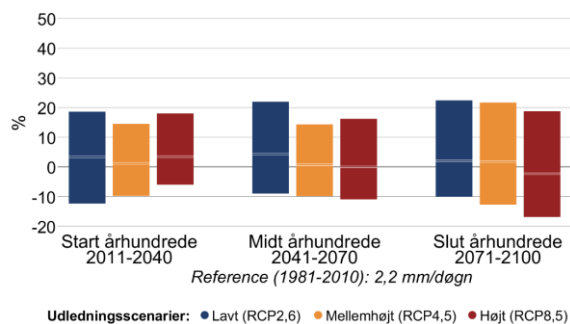
Figur 6 Procentvis ændring af middelnedbør mellem 1981-2010 og fremtidsperioderne 2011-2040, 2041-2070 og 2071-2100 under forskellige udledningsscenarier i Middelfart Kommune. Til venstre sommer (jun-aug), til højre vinter (dec-feb).
