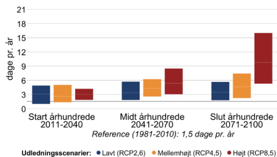
Figur 3 Ændring af gennemsnitstemperatur og antallet af hedebølgedage hen over året mellem 1981-2010 og fremtidsperioderne 2011-2040, 2041-2070 og 2071-2100 under forskellige udledningsscenarier i Middelfart Kommune.
