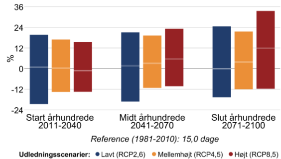
Figur 8 Procentvis ændring af tørre dage om sommeren (jun-aug) mellem 1981-2010 og fremtidsperioderne 2011-2040, 2041-2070 og 2071-2100 under forskellige udledningsscenarier i Middelfart Kommune. Til venstre antallet af tørre dage med mindre end 1 mm nedbør, til højre længden af den længste sammenhængende tørre periode.
