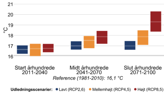
Figur 4 Gennemsnitstemperatur for sommer (jun-aug) og vinter (dec-feb) i fremtidsperioderne 2011-2040, 2041-2070 og 2071-2100 under forskellige udledningsscenarier i Middelfart Kommune. Den grå linje viser referenceværdien for nutiden (1981-2010).
