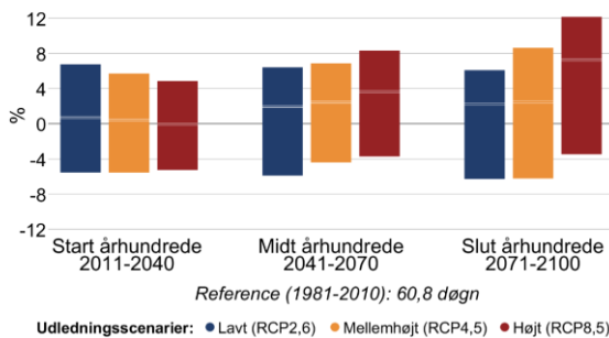
Figur 8 Procentvis ændring af tørre dage om sommeren (jun-aug) mellem 1981-2010 og fremtidsperioderne 2011-2040, 2041-2070 og 2071-2100 under forskellige udledningsscenarier i Middelfart Kommune. Til venstre antallet af tørre dage med mindre end 1 mm nedbør, til højre længden af den længste sammenhængende tørre periode.
