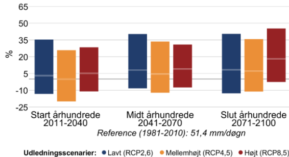
Figur 7 Procentvis ændring af ekstremnedbør hen over året mellem 1981-2010 og fremtidsperioderne 2011-2040, 2041-2070 og 2071-2100 under forskellige udledningsscenarier i Middelfart Kommune. Til venstre 10-årshændelsen for døgnnedbør, til højre frekvensen af skybrud.
