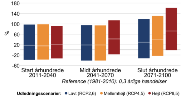
Figur 7 Procentvis ændring af ekstremnedbør hen over året mellem 1981-2010 og fremtidsperioderne 2011-2040, 2041-2070 og 2071-2100 under forskellige udledningsscenarier i Middelfart Kommune. Til venstre 10-årshændelsen for døgnnedbør, til højre frekvensen af skybrud.
