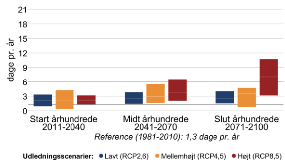
Figur 3 Ændring af gennemsnitstemperatur og antallet af hedebølgedage hen over året mellem 1981-2010 og fremtidsperioderne 2011-2040, 2041-2070 og 2071-2100 under forskellige udledningsscenarier i Lemvig Kommune.
