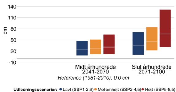
Figur 10 Ændring i middelvandstand (venstre) og hyppigheden af stormflod for Vestkyst central i fremtidsperioderne 2041-2070 og 2071-2100 under forskellige udledningsscenarioer. Den grå linje viser referenceværdien for nutiden (1981-2010). En
