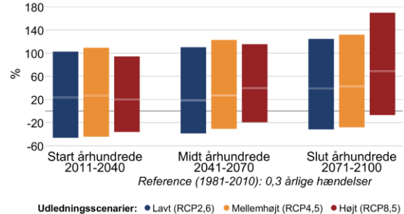
Figur 7 Procentvis ændring af ekstremnedbør hen over året mellem 1981-2010 og fremtidsperioderne 2011-2040, 2041-2070 og 2071-2100 under forskellige udledningsscenarier i Lemvig Kommune. Til venstre 10-årshændelsen for døgnnedbør, til højre frekvensen af skybrud.
