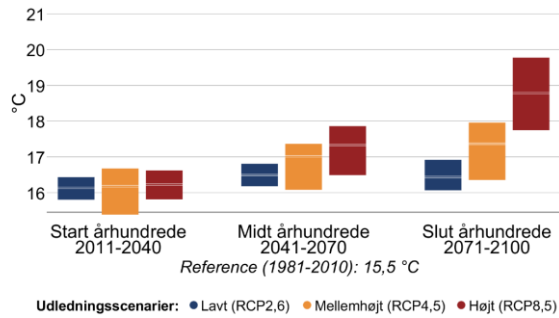
Figur 4 Gennemsnitstemperatur for sommer (jun-aug) og vinter (dec-feb) i fremtidsperioderne 2011-2040, 2041-2070 og 2071-2100 under forskellige udledningsscenarier i Lemvig Kommune. Den grå linje viser referenceværdien for nutiden (1981-2010).
