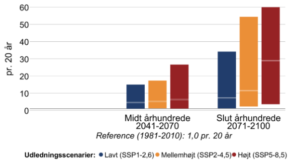
Figur 12 Ændring i middelvandstand (venstre) og hyppigheden af stormflod for Vestkysten ud for Limfjorden i fremtidsperioderne 2041-2070 og 2071-2100 under forskellige udledningsscenarioer. Den grå linje viser referenceværdien for nutiden (1981-2010). En stormflod defineres her som en forhøjet vandstand, der statistisk set kun forekommer én gang hvert 20. år i perioden 1981-2010. Bemærk også at denne indikator kappes ved 60 stormfloder per 20 år.
