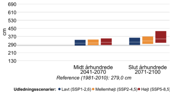
Figur 11 Højden af 20- (venstre) og 100-års (højre) stormflodhændelser for Vestkyst central i fremtidsperioderne 2041-2070 og 2071-2100 under forskellige udledningsscenarioer. Den grå linje viser referenceværdien for nutiden (1981-2010).
