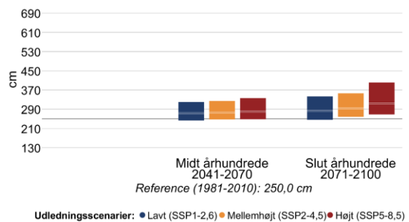
Figur 13 Højden af 20- (venstre) og 100-års (højre) stormflodhændelser for Vestkysten ud for Limfjorden i fremtidsperioderne 2041-2070 og 2071-2100 under forskellige udledningsscenarioer. Den grå linje viser referenceværdien for nutiden (1981-2010).
