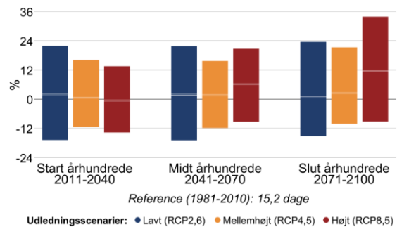
Figur 8 Procentvis ændring af tørre dage om sommeren (jun-aug) mellem 1981-2010 og fremtidsperioderne 2011-2040, 2041-2070 og 2071-2100 under forskellige udledningsscenarier i Lemvig Kommune. Til venstre antallet af tørre dage med mindre end 1 mm nedbør, til højre længden af den længste sammenhængende tørre periode.
