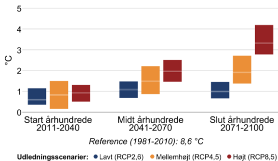
Figur 3 Ændring af gennemsnitstemperatur og antallet af hedebølgedage hen over året mellem 1981-2010 og fremtidsperioderne 2011-2040, 2041-2070 og 2071-2100 under forskellige udledningsscenarier i Lemvig Kommune.
