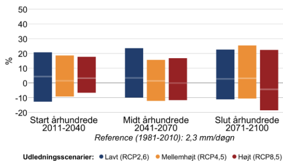
Figur 6 Procentvis ændring af middelnedbør mellem 1981-2010 og fremtidsperioderne 2011-2040, 2041-2070 og 2071-2100 under forskellige udledningsscenarier i Lemvig Kommune. Til venstre sommer (jun-aug), til højre vinter (dec-feb).
