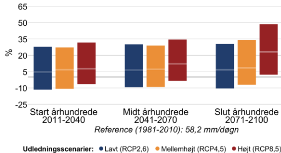
Figur 7 Procentvis ændring af ekstremnedbør hen over året mellem 1981-2010 og fremtidsperioderne 2011-2040, 2041-2070 og 2071-2100 under forskellige udledningsscenarier i Lemvig Kommune. Til venstre 10-årshændelsen for døgnnedbør, til højre frekvensen af skybrud.
