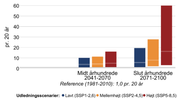
Figur 10 Ændring i middelvandstand (venstre) og hyppigheden af stormflod for Vestkyst central i fremtidsperioderne 2041-2070 og 2071-2100 under forskellige udledningsscenarioer. Den grå linje viser referenceværdien for nutiden (1981-2010). En
