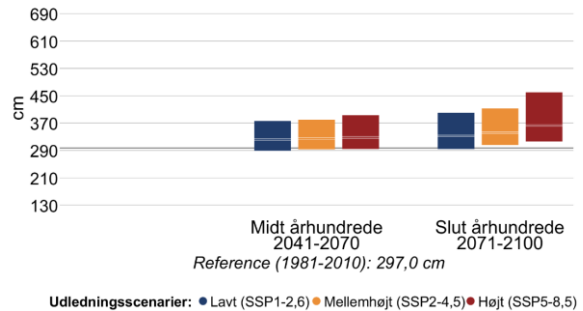
Figur 11 Højden af 20- (venstre) og 100-års (højre) stormflodhændelser for Vestkyst central i fremtidsperioderne 2041-2070 og 2071-2100 under forskellige udledningsscenarioer. Den grå linje viser referenceværdien for nutiden (1981-2010).
