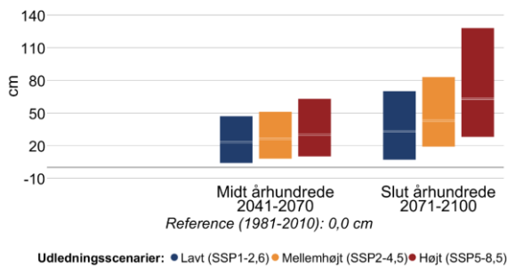
Figur 12 Ændring i middelvandstand (venstre) og hyppigheden af stormflod for Vestkysten ud for Limfjorden i fremtidsperioderne 2041-2070 og 2071-2100 under forskellige udledningsscenarioer. Den grå linje viser referenceværdien for nutiden (1981-2010). En stormflod defineres her som en forhøjet vandstand, der statistisk set kun forekommer én gang hvert 20. år i perioden 1981-2010. Bemærk også at denne indikator kappes ved 60 stormfloder per 20 år.
