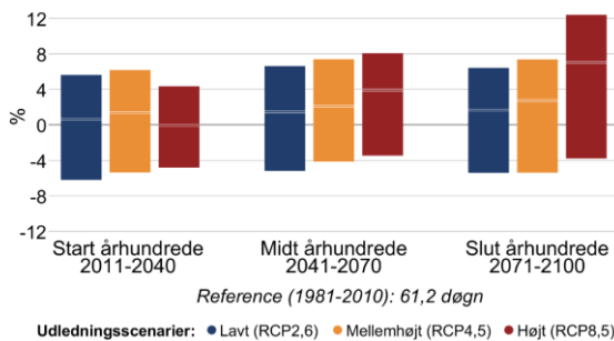
Figur 8 Procentvis ændring af tørre dage om sommeren (jun-aug) mellem 1981-2010 og fremtidsperioderne 2011-2040, 2041-2070 og 2071-2100 under forskellige udledningsscenarier i Lemvig Kommune. Til venstre antallet af tørre dage med mindre end 1 mm nedbør, til højre længden af den længste sammenhængende tørre periode.
