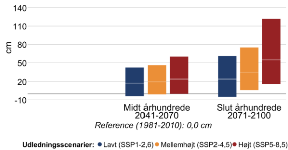
Figur 12 Ændring i middelvandstand (venstre) og hyppigheden af stormflod for Roskilde Fjord i fremtidsperioderne 2041-2070 og 2071-2100 under forskellige udledningsscenarier. Den grå linje viser referenceværdien for nutiden (1981-2010). En stormflod defineres her som en forhøjet vandstand, der statistisk set kun forekommer én gang hvert 20. år i perioden 1981-2010. Bemærk også at denne indikator kappes ved 60 stormfloder per 20 år.
