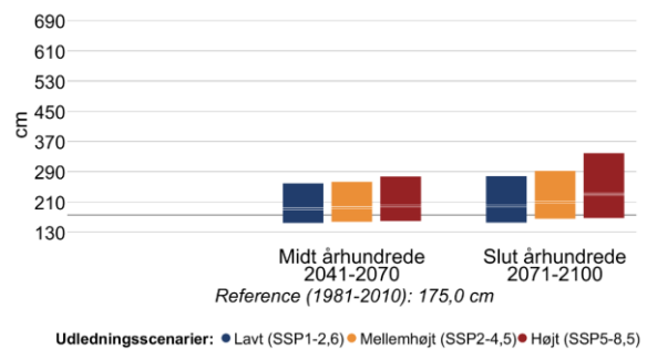
Figur 13 Højden af 20- (venstre) og 100-års (højre) stormflodhændelser for Roskilde Fjord i fremtidsperioderne 2041-2070 og 2071-2100 under forskellige udledningsscenarier. Den grå linje viser referenceværdien for nutiden (1981-2010).
