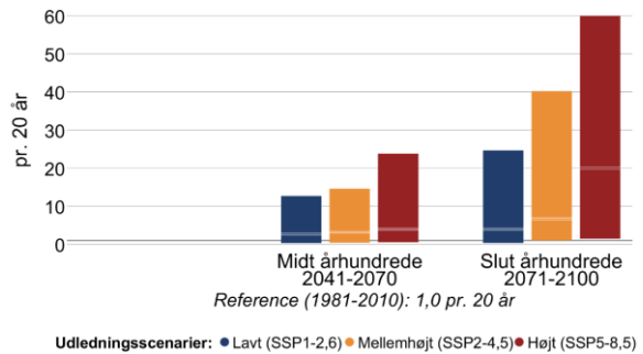
Figur 12 Ændring i middelvandstand (venstre) og hyppigheden af stormflod for Roskilde Fjord i fremtidsperioderne 2041-2070 og 2071-2100 under forskellige udledningsscenarier. Den grå linje viser referenceværdien for nutiden (1981-2010). En stormflod defineres her som en forhøjet vandstand, der statistisk set kun forekommer én gang hvert 20. år i perioden 1981-2010. Bemærk også at denne indikator kappes ved 60 stormfloder per 20 år.
