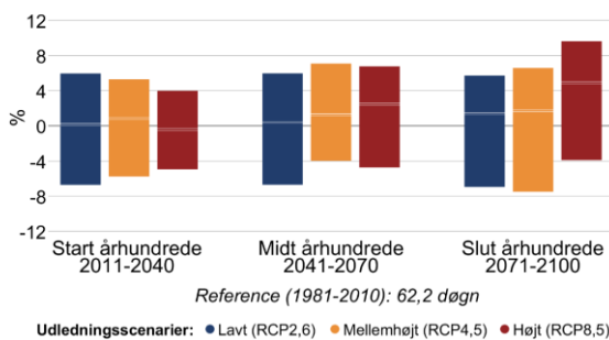
Figur 8 Procentvis ændring af tørre dage om sommeren (jun-aug) mellem 1981-2010 og fremtidsperioderne 2011-2040, 2041-2070 og 2071-2100 under forskellige udledningsscenarier i Lejre Kommune. Til venstre antallet af tørre dage med mindre end 1 mm nedbør, til højre længden af den længste sammenhængende tørre periode.
