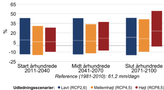
Figur 7 Procentvis ændring af ekstremnedbør hen over året mellem 1981-2010 og fremtidsperioderne 2011-2040, 2041-2070 og 2071-2100 under forskellige udledningsscenarier i Lejre Kommune. Til venstre 10-årshændelsen for døgnnedbør, til højre frekvensen af skybrud.
