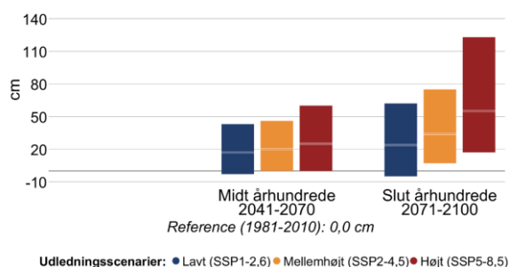
Figur 10 Ændring i middelvandstand (venstre) og hyppigheden af stormflod for Isefjord i fremtidsperioderne 2041-2070 og 2071-2100 under forskellige udledningsscenarioer. Den grå linje viser referenceværdien for nutiden (1981-2010). En stormflod defineres her som en forhøjet vandstand, der statistisk set kun forekommer én gang hvert 20. år i perioden 1981-2010. Bemærk også at denne indikator kappes ved 60 stormfloder per 20 år.
