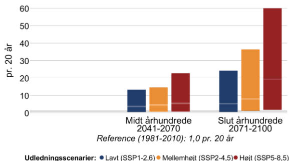
Figur 10 Ændring i middelvandstand (venstre) og hyppigheden af stormflod for Isefjord i fremtidsperioderne 2041-2070 og 2071-2100 under forskellige udledningsscenarioer. Den grå linje viser referenceværdien for nutiden (1981-2010). En stormflod defineres her som en forhøjet vandstand, der statistisk set kun forekommer én gang hvert 20. år i perioden 1981-2010. Bemærk også at denne indikator kappes ved 60 stormfloder per 20 år.
