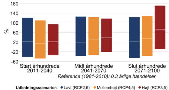
Figur 7 Procentvis ændring af ekstremnedbør hen over året mellem 1981-2010 og fremtidsperioderne 2011-2040, 2041-2070 og 2071-2100 under forskellige udledningsscenarier i Lejre Kommune. Til venstre 10-årshændelsen for døgnnedbør, til højre frekvensen af skybrud.
