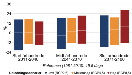
Figur 8 Procentvis ændring af tørre dage om sommeren (jun-aug) mellem 1981-2010 og fremtidsperioderne 2011-2040, 2041-2070 og 2071-2100 under forskellige udledningsscenarier i Lejre Kommune. Til venstre antallet af tørre dage med mindre end 1 mm nedbør, til højre længden af den længste sammenhængende tørre periode.
