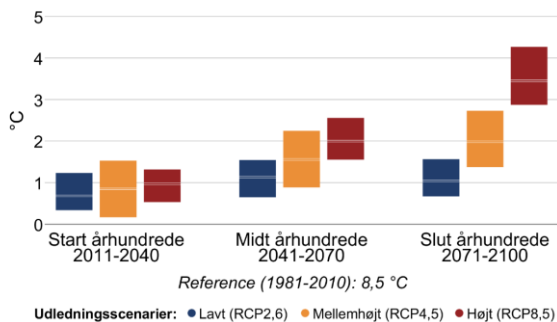
Figur 3 Ændring af gennemsnitstemperatur og antallet af hedebløgedage hen over året mellem 1981-2010 og fremtidsperioderne 2011-2040, 2041-2070 og 2071-2100 under forskellige udledningsscenarier i Lejre Kommune.
