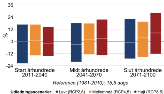
Figur 8 Procentvis ændring af tørre dage om sommeren (jun-aug) mellem 1981-2010 og fremtidsperioderne 2011-2040, 2041-2070 og 2071-2100 under forskellige udledningsscenarier i Køge Kommune. Til venstre antallet af tørre dage med mindre end 1 mm nedbør, til højre længden af den længste sammenhængende tørre periode.
