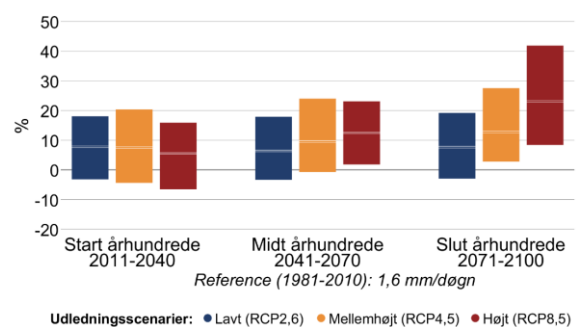
Figur 6 Procentvis ændring af middelnedbør mellem 1981-2010 og fremtidsperioderne 2011-2040, 2041-2070 og 2071-2100 under forskellige udledningsscenarier i Køge Kommune. Til venstre sommer (jun-aug), til højre vinter (dec-feb).
