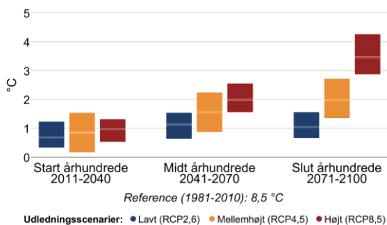
Figur 3 Ændring af gennemsnitstemperatur og antallet af hedebølgedage hen over året mellem 1981-2010 og fremtidsperioderne 2011-2040, 2041-2070 og 2071-2100 under forskellige udledningsscenarier i Køge Kommune.
