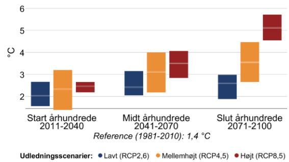
Figur 4 Gennemsnitstemperatur for sommer (jun-aug) og vinter (dec-feb) i fremtidsperioderne 2011-2040, 2041-2070 og 2071-2100 under forskellige udledningsscenarier i Køge Kommune. Den grå linje viser referenceværdien for nutiden (1981-2010).
