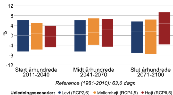
Figur 8 Procentvis ændring af tørre dage om sommeren (jun-aug) mellem 1981-2010 og fremtidsperioderne 2011-2040, 2041-2070 og 2071-2100 under forskellige udledningsscenarier i Køge Kommune. Til venstre antallet af tørre dage med mindre end 1 mm nedbør, til højre længden af den længste sammenhængende tørre periode.
