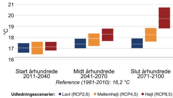
Figur 4 Gennemsnitstemperatur for sommer (jun-aug) og vinter (dec-feb) i fremtidsperioderne 2011-2040, 2041-2070 og 2071-2100 under forskellige udledningsscenarier i Køge Kommune. Den grå linje viser referenceværdien for nutiden (1981-2010).
