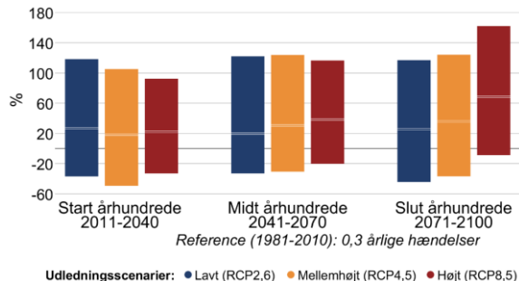
Figur 7 Procentvis ændring af ekstremnedbør hen over året mellem 1981-2010 og fremtidsperioderne 2011-2040, 2041-2070 og 2071-2100 under forskellige udledningsscenarier i Køge Kommune. Til venstre 10-årshændelsen for døgnet nedbør, til højre frekvensen af skybrud.
