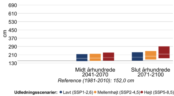
Figur 11 Højden af 20- (venstre) og 100-års (højre) stormflodhændelser for Storebælt nordvest og Odense Fjord i fremtidsperioderne 2041-2070 og 2071-2100 under forskellige udledningsscenarier. Den grå linje viser referenceværdien for nutiden (1981-2010).
