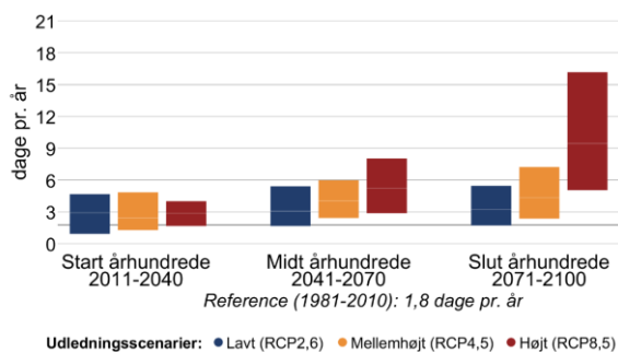
Figur 3 Ændring af gennemsnitstemperatur og antallet af hedebølgedage hen over året mellem 1981-2010 og fremtidsperioderne 2011-2040, 2041-2070 og 2071-2100 under forskellige udledningsscenarier i Kerteminde Kommune.
