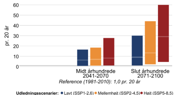
Figur 10 Ændring i middelvandstand (venstre) og hyppigheden af stormflod for Storebælt nordvest og Odense Fjord i fremtidsperioderne 2041-2070 og 2071-2100 under forskellige udledningsscenarioer. Den grå linje viser referenceværdien for nutiden (1981-2010). En stormflod defineres her som en forhøjet vandstand, der statistisk set kun forekommer én gang hvert 20. år i perioden 1981-2010. Bemærk også at denne indikator kappes ved 60 stormfloder per 20 år.
