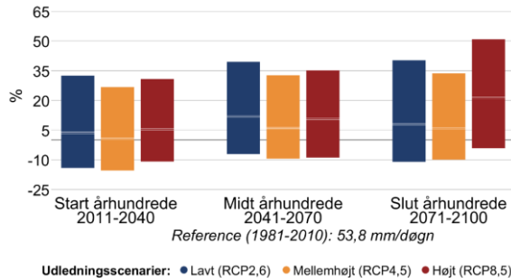
Figur 7 Procentvis ændring af ekstremnedbør hen over året mellem 1981-2010 og fremtidsperioderne 2011-2040, 2041-2070 og 2071-2100 under forskellige udledningsscenarier i Kerteminde Kommune. Til venstre 10-årshændelsen for døgnnedbør, til højre frekvensen af skybrud.
