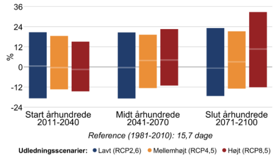
Figur 8 Procentvis ændring af tørre dage om sommeren (jun-aug) mellem 1981-2010 og fremtidsperioderne 2011-2040, 2041-2070 og 2071-2100 under forskellige udledningsscenarier i Kerteminde Kommune. Til venstre antallet af tørre dage med mindre end 1 mm nedbør, til højre længden af den længste sammenhængende tørre periode.
