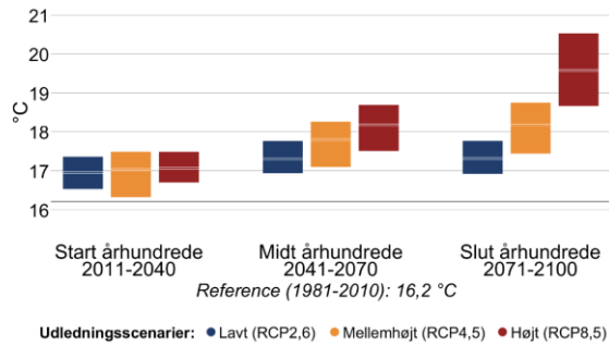
Figur 4 Gennemsnitstemperatur for sommer (jun-aug) og vinter (dec-feb) i fremtidsperioderne 2011-2040, 2041-2070 og 2071-2100 under forskellige udledningsscenarier i Kerteminde Kommune. Den grå linje viser referenceværdien for nutiden (1981-2010).
