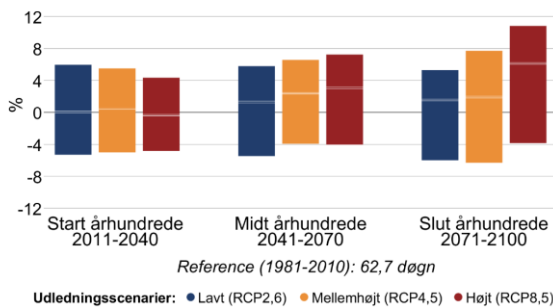
Figur 8 Procentvis ændring af tørre dage om sommeren (jun-aug) mellem 1981-2010 og fremtidsperioderne 2011-2040, 2041-2070 og 2071-2100 under forskellige udledningsscenarier i Kerteminde Kommune. Til venstre antallet af tørre dage med mindre end 1 mm nedbør, til højre længden af den længste sammenhængende tørre periode.
