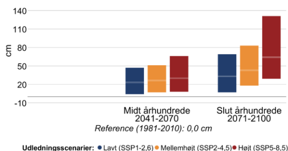
Figur 10 Ændring i middelvandstand (venstre) og hyppigheden af stormflod for Storebælt nordvest og Odense Fjord i fremtidsperioderne 2041-2070 og 2071-2100 under forskellige udledningsscenarioer. Den grå linje viser referenceværdien for nutiden (1981-2010). En stormflod defineres her som en forhøjet vandstand, der statistisk set kun forekommer én gang hvert 20. år i perioden 1981-2010. Bemærk også at denne indikator kappes ved 60 stormfloder per 20 år.
