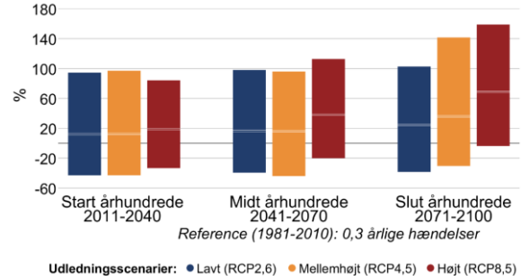
Figur 7 Procentvis ændring af ekstremnedbør hen over året mellem 1981-2010 og fremtidsperioderne 2011-2040, 2041-2070 og 2071-2100 under forskellige udledningsscenarier i Kerteminde Kommune. Til venstre 10-årshændelsen for døgnnedbør, til højre frekvensen af skybrud.
