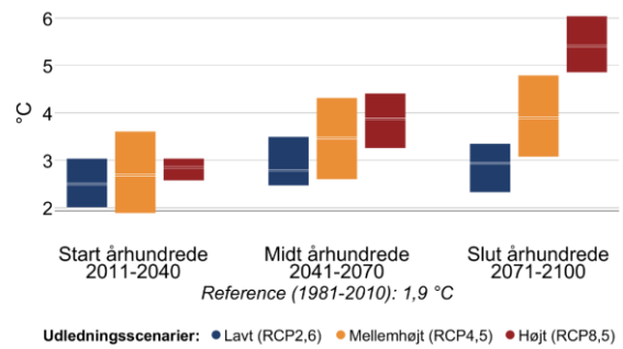
Figur 4 Gennemsnitstemperatur for sommer (jun-aug) og vinter (dec-feb) i fremtidsperioderne 2011-2040, 2041-2070 og 2071-2100 under forskellige udledningsscenarier i Kerteminde Kommune. Den grå linje viser referenceværdien for nutiden (1981-2010).
