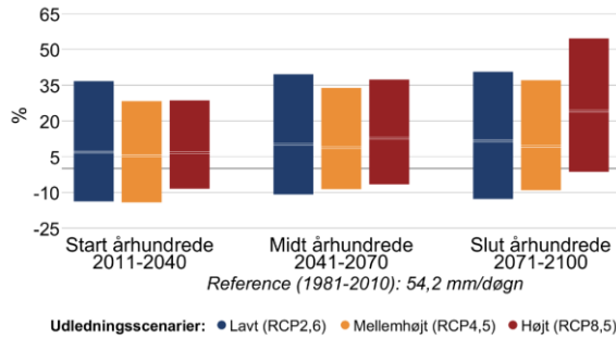
Figur 7 Procentvis ændring af ekstremnedbør hen over året mellem 1981-2010 og fremtidsperioderne 2011-2040, 2041-2070 og 2071-2100 under forskellige udledningsscenarier i Kalundborg Kommune. Til venstre 10-årshændelsen for døgnnedbør, til højre frekvensen af skybrud.
