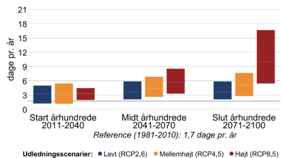
Figur 3 Ændring af gennemsnitstemperatur og antallet af hedebølgedage hen over året mellem 1981-2010 og fremtidsperioderne 2011-2040, 2041-2070 og 2071-2100 under forskellige udledningsscenarier i Kalundborg Kommune.
