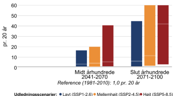
Figur 12 Ændring i middelvandstand (venstre) og hyppigheden af stormflod for Sejrø Bugt i fremtidsperioderne 2041-2070 og 2071-2100 under forskellige udledningsscenarier. Den grå linje viser referenceværdien for nutiden (1981-2010). En stormflod defineres her som en forhøjet vandstand, der statistisk set kun forekommer én gang hvert 20. år i perioden 1981-2010. Bemærk også at denne indikator kappes ved 60 stormfloder per 20 år.
