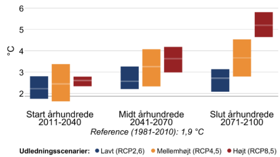
Figur 4 Gennemsnitstemperatur for sommer (jun-aug) og vinter (dec-feb) i fremtidsperioderne 2011-2040, 2041-2070 og 2071-2100 under forskellige udledningsscenarier i Kalundborg Kommune. Den grå linje viser referenceværdien for nutiden (1981-2010).
