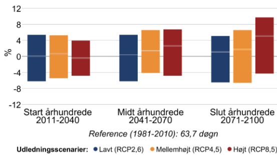
Figur 8 Procentvis ændring af tørre dage om sommeren (jun-aug) mellem 1981-2010 og fremtidsperioderne 2011-2040, 2041-2070 og 2071-2100 under forskellige udledningsscenarier i Kalundborg Kommune. Til venstre antallet af tørre dage med mindre end 1 mm nedbør, til højre længden af den længste sammenhængende tørre periode.
