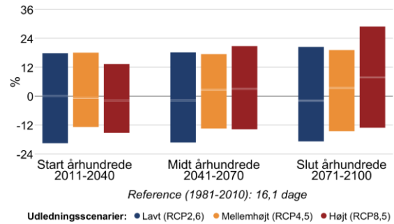
Figur 8 Procentvis ændring af tørre dage om sommeren (jun-aug) mellem 1981-2010 og fremtidsperioderne 2011-2040, 2041-2070 og 2071-2100 under forskellige udledningsscenarier i Kalundborg Kommune. Til venstre antallet af tørre dage med mindre end 1 mm nedbør, til højre længden af den længste sammenhængende tørre periode.
