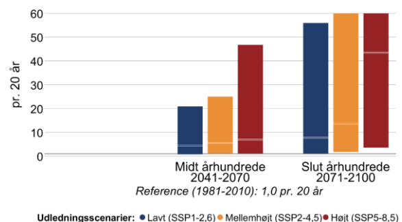
Figur 10 Ændring i middelvandstand (venstre) og hyppigheden af stormflod for Storebælt nordøst i fremtidsperioderne 2041-2070 og 2071-2100 under forskellige udledningsscenarioer. Den grå linje viser referenceværdien for nutiden (1981-2010). En stormflod defineres her som en forhøjet vandstand, der statistisk set kun forekommer én gang hvert 20. år i perioden 1981-2010. Bemærk også at denne indikator kappes ved 60 stormfloder per 20 år.
