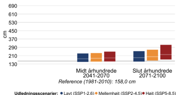
Figur 11 Højden af 20- (venstre) og 100-års (højre) stormflodhændelser for Storebælt nordøst i fremtidsperioderne 2041-2070 og 2071-2100 under forskellige udledningsscenarier. Den grå linje viser referenceværdien for nutiden (1981-2010).
