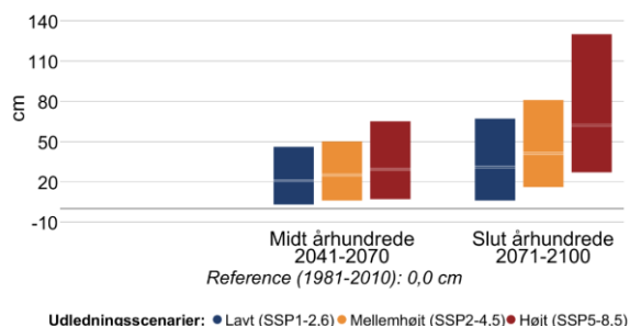
Figur 12 Ændring i middelvandstand (venstre) og hyppigheden af stormflod for Sejrø Bugt i fremtidsperioderne 2041-2070 og 2071-2100 under forskellige udledningsscenarier. Den grå linje viser referenceværdien for nutiden (1981-2010). En stormflod defineres her som en forhøjet vandstand, der statistisk set kun forekommer én gang hvert 20. år i perioden 1981-2010. Bemærk også at denne indikator kappes ved 60 stormfloder per 20 år.
