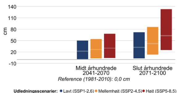
Figur 10 Ændring i middelvandstand (venstre) og hyppigheden af stormflod for Storebælt nordøst i fremtidsperioderne 2041-2070 og 2071-2100 under forskellige udledningsscenarioer. Den grå linje viser referenceværdien for nutiden (1981-2010). En stormflod defineres her som en forhøjet vandstand, der statistisk set kun forekommer én gang hvert 20. år i perioden 1981-2010. Bemærk også at denne indikator kappes ved 60 stormfloder per 20 år.
