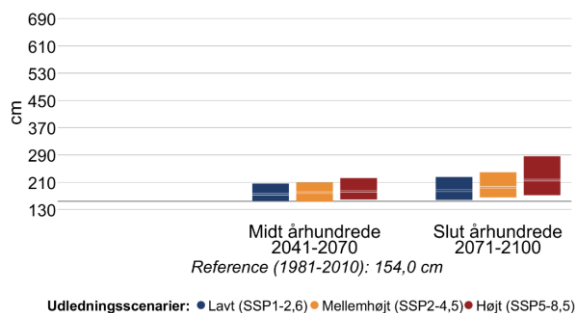
Figur 13 Højden af 20- (venstre) og 100-års (højre) stormflodhændelser for Sejrø Bugt i fremtidsperioderne 2041-2070 og 2071-2100 under forskellige udledningsscenarier. Den grå linje viser referenceværdien for nutiden (1981-2010).
