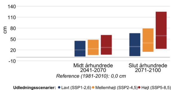
Figur 10 Ændring i middelvandstand (venstre) og hyppigheden af stormflod for Skagerrakkyst sydlige i fremtidsperioderne 2041-2070 og 2071-2100 under forskellige udledningsscenarioer. Den grå linje viser referenceværdien for nutiden (1981-2010).
