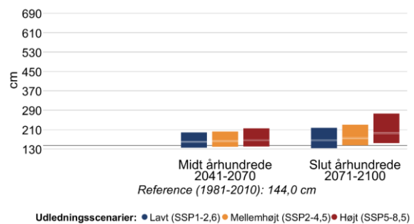
Figur 13 Højden af 20- (venstre) og 100-års (højre) stormflodhændelser for Skagerrakkyst nordlig i fremtidsperioderne 2041-2070 og 2071-2100 under forskellige udledningsscenarier. Den grå linje viser referenceværdien for nutiden (1981-2010).
