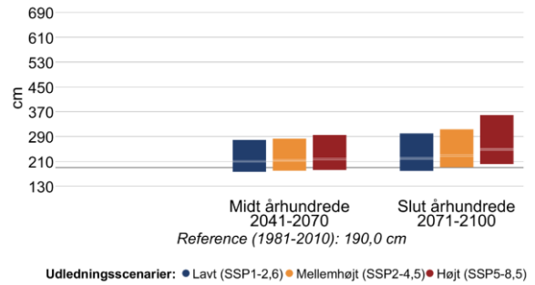
Figur 17 Højden af 20- (venstre) og 100-års (højre) stormflodhændelser for Limfjorden ved Thisted i fremtidsperioderne 2041-2070 og 2071-2100 under forskellige udledningsscenarier. Den grå linje viser referenceværdien for nutiden (1981-2010).
