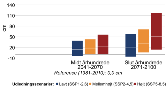
Figur 12 Ændring i middelvandstand (venstre) og hyppigheden af stormflod for Skagerrakkyst nordlig i fremtidsperioderne 2041-2070 og 2071-2100 under forskellige udledningsscenarier. Den grå linje viser referenceværdien for nutiden (1981-2010). En stormflod defineres her som en forhøjet vandstand, der statistisk set kun forekommer én gang hvert 20. år i perioden 1981-2010. Bemærk også at denne indikator kappes ved 60 stormfloder per 20 år.
