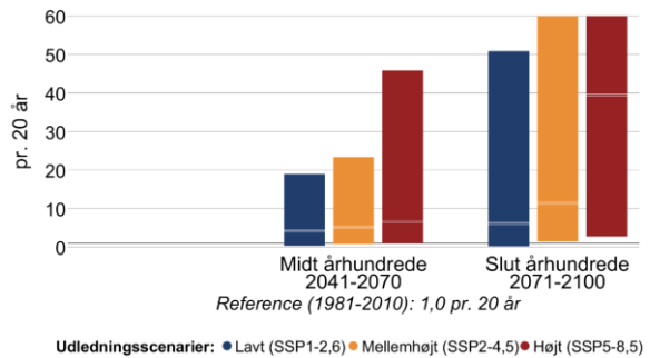
Figur 12 Ændring i middelvandstand (venstre) og hyppigheden af stormflod for Skagerrakkyst nordlig i fremtidsperioderne 2041-2070 og 2071-2100 under forskellige udledningsscenarier. Den grå linje viser referenceværdien for nutiden (1981-2010). En stormflod defineres her som en forhøjet vandstand, der statistisk set kun forekommer én gang hvert 20. år i perioden 1981-2010. Bemærk også at denne indikator kappes ved 60 stormfloder per 20 år.
