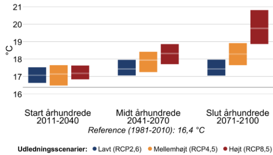
Figur 4 Gennemsnitstemperatur for sommer (jun-aug) og vinter (dec-feb) i fremtidsperioderne 2011-2040, 2041-2070 og 2071-2100 under forskellige udledningsscenarier i Ishøj Kommune. Den grå linje viser referenceværdien for nutiden (1981-2010).
