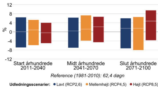
Figur 8 Procentvis ændring af tørre dage om sommeren (jun-aug) mellem 1981-2010 og fremtidsperioderne 2011-2040, 2041-2070 og 2071-2100 under forskellige udledningsscenarier i Ishøj Kommune. Til venstre antallet af tørre dage med mindre end 1 mm nedbør, til højre længden af den længste sammenhængende tørre periode.
