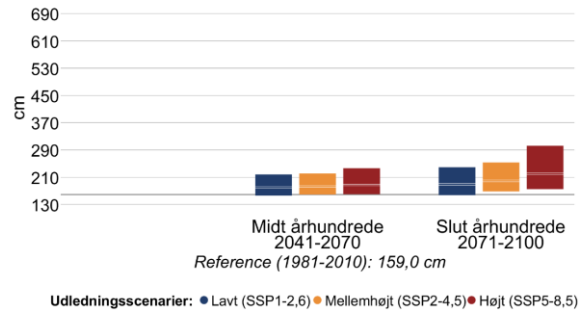
Figur 11 Højden af 20- (venstre) og 100-års (højre) stormflodhændelser for Køge Bugt i fremtidsperioderne 2041-2070 og 2071-2100 under forskellige udledningsscenarier. Den grå linje viser referenceværdien for nutiden (1981-2010).
