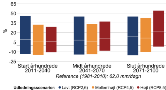
Figur 7 Procentvis ændring af ekstremnedbør hen over året mellem 1981-2010 og fremtidsperioderne 2011-2040, 2041-2070 og 2071-2100 under forskellige udledningsscenarier i Ishøj Kommune. Til venstre 10-årshændelsen for døgnnedbør, til højre frekvensen af skybrud.
