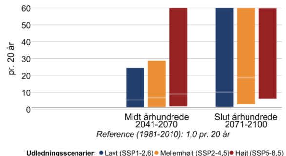
Figur 10 Ændring i middelvandstand (venstre) og hyppigheden af stormflod for Køge Bugt i fremtidsperioderne 2041-2070 og 2071-2100 under forskellige udledningsscenarioer. Den grå linje viser referenceværdien for nutiden (1981-2010). En stormflod defineres her som en forhøjet vandstand, der statistisk set kun forekommer én gang hvert 20. år i perioden 1981-2010. Bemærk også at denne indikator kappes ved 60 stormfloder per 20 år.
