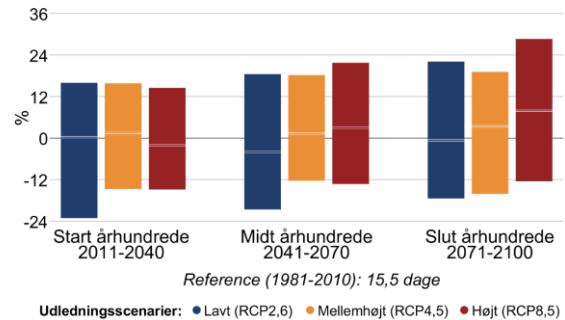
Figur 8 Procentvis ændring af tørre dage om sommeren (jun-aug) mellem 1981-2010 og fremtidsperioderne 2011-2040, 2041-2070 og 2071-2100 under forskellige udledningsscenarier i Ishøj Kommune. Til venstre antallet af tørre dage med mindre end 1 mm nedbør, til højre længden af den længste sammenhængende tørre periode.
