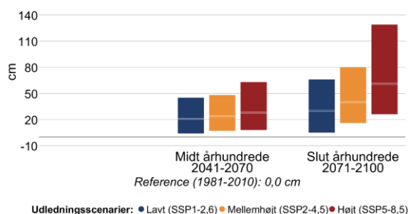
Figur 10 Ændring i middelvandstand (venstre) og hyppigheden af stormflod for Køge Bugt i fremtidsperioderne 2041-2070 og 2071-2100 under forskellige udledningsscenarioer. Den grå linje viser referenceværdien for nutiden (1981-2010). En stormflod defineres her som en forhøjet vandstand, der statistisk set kun forekommer én gang hvert 20. år i perioden 1981-2010. Bemærk også at denne indikator kappes ved 60 stormfloder per 20 år.
