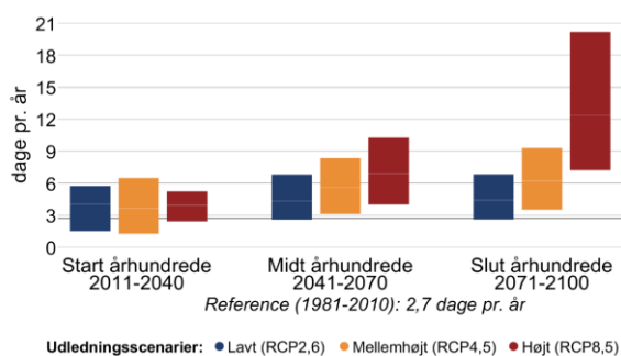
Figur 3 Ændring af gennemsnitstemperatur og antallet af hedebløddage hen over året mellem 1981-2010 og fremtidsperioderne 2011-2040, 2041-2070 og 2071-2100 under forskellige udledningsscenarier i Ishøj Kommune.
