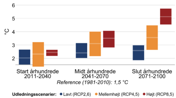
Figur 4 Gennemsnitstemperatur for sommer (jun-aug) og vinter (dec-feb) i fremtidsperioderne 2011-2040, 2041-2070 og 2071-2100 under forskellige udledningsscenarier i Ishøj Kommune. Den grå linje viser referenceværdien for nutiden (1981-2010).
