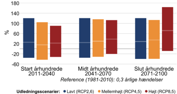
Figur 7 Procentvis ændring af ekstremnedbør hen over året mellem 1981-2010 og fremtidsperioderne 2011-2040, 2041-2070 og 2071-2100 under forskellige udledningsscenarier i Ishøj Kommune. Til venstre 10-årshændelsen for døgnnedbør, til højre frekvensen af skybrud.
