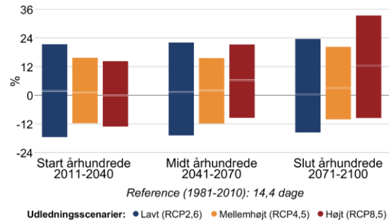
Figur 8 Procentvis ændring af tørre dage om sommeren (jun-aug) mellem 1981-2010 og fremtidsperioderne 2011-2040, 2041-2070 og 2071-2100 under forskellige udledningsscenarier i Holstebro Kommune. Til venstre antallet af tørre dage med mindre end 1 mm nedbør, til højre længden af den længste sammenhængende tørre periode.
