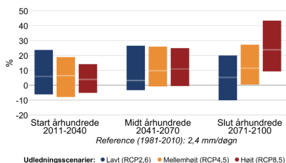
Figur 6 Procentvis ændring af middelnedbør mellem 1981-2010 og fremtidsperioderne 2011-2040, 2041-2070 og 2071-2100 under forskellige udledningsscenarier i Holstebro Kommune. Til venstre sommer (jun-aug), til højre vinter (dec-feb).
