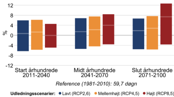
Figur 8 Procentvis ændring af tørre dage om sommeren (jun-aug) mellem 1981-2010 og fremtidsperioderne 2011-2040, 2041-2070 og 2071-2100 under forskellige udledningsscenarier i Holstebro Kommune. Til venstre antallet af tørre dage med mindre end 1 mm nedbør, til højre længden af den længste sammenhængende tørre periode.
