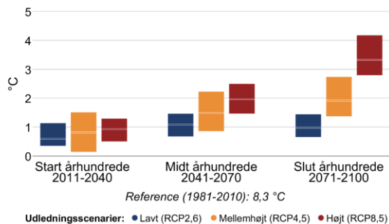
Figur 3 Ændring af gennemsnitstemperatur og antallet af hedebølgedage hen over året mellem 1981-2010 og fremtidsperioderne 2011-2040, 2041-2070 og 2071-2100 under forskellige udledningsscenarier i Holstebro Kommune.
