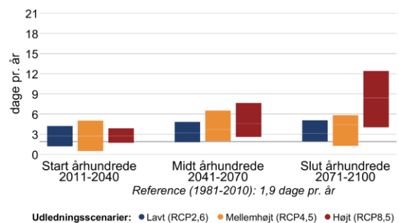
Figur 3 Ændring af gennemsnitstemperatur og antallet af hedebølgedage hen over året mellem 1981-2010 og fremtidsperioderne 2011-2040, 2041-2070 og 2071-2100 under forskellige udledningsscenarier i Holstebro Kommune.
