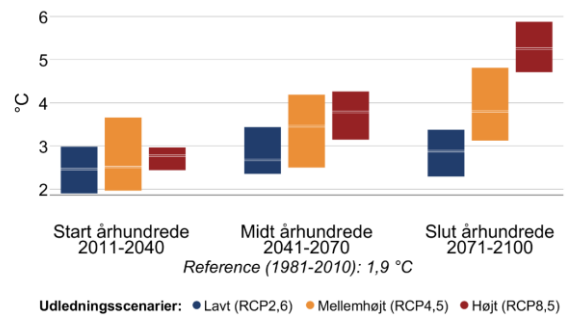
Figur 4 Gennemsnitstemperatur for sommer (jun-aug) og vinter (dec-feb) i fremtidsperioderne 2011-2040, 2041-2070 og 2071-2100 under forskellige udledningsscenarier i Holstebro Kommune. Den grå linje viser referenceværdien for nutiden (1981-2010).
