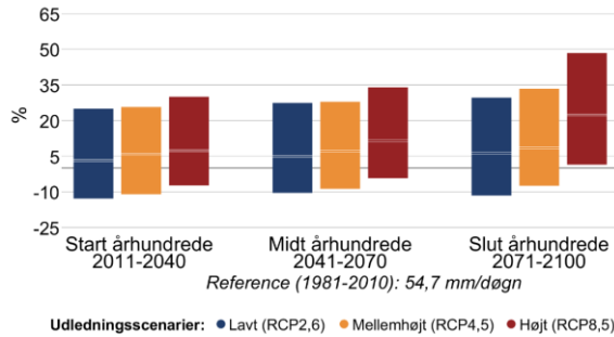
Figur 7 Procentvis ændring af ekstremnedbør hen over året mellem 1981-2010 og fremtidsperioderne 2011-2040, 2041-2070 og 2071-2100 under forskellige udledningsscenarier i Holstebro Kommune. Til venstre 10-årshændelsen for døgnnedbør, til højre frekvensen af skybrud.
