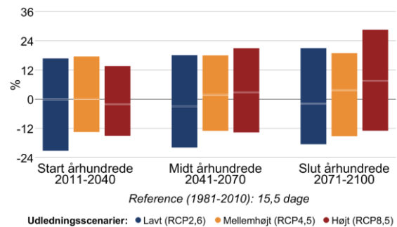
Figur 8 Procentvis ændring af tørre dage om sommeren (jun-aug) mellem 1981-2010 og fremtidsperioderne 2011-2040, 2041-2070 og 2071-2100 under forskellige udledningsscenarier i Holbæk Kommune. Til venstre antallet af tørre dage med mindre end 1 mm nedbør, til højre længden af den længste sammenhængende tørre periode.
