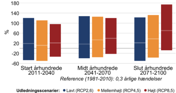
Figur 7 Procentvis ændring af ekstremnedbør hen over året mellem 1981-2010 og fremtidsperioderne 2011-2040, 2041-2070 og 2071-2100 under forskellige udledningsscenarier i Holbæk Kommune. Til venstre 10-årshændelsen for døgnnedbør, til højre frekvensen af skybrud.
