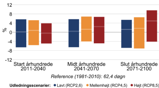
Figur 8 Procentvis ændring af tørre dage om sommeren (jun-aug) mellem 1981-2010 og fremtidsperioderne 2011-2040, 2041-2070 og 2071-2100 under forskellige udledningsscenarier i Holbæk Kommune. Til venstre antallet af tørre dage med mindre end 1 mm nedbør, til højre længden af den længste sammenhængende tørre periode.
