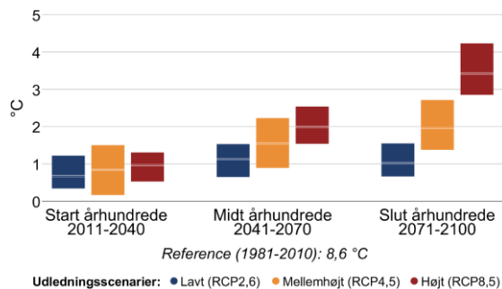
Figur 3 Ændring af gennemsnitstemperatur og antallet af hedebløddage hen over året mellem 1981-2010 og fremtidsperioderne 2011-2040, 2041-2070 og 2071-2100 under forskellige udledningsscenarier i Holbæk Kommune.
