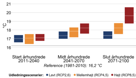
Figur 4 Gennemsnitstemperatur for sommer (jun-aug) og vinter (dec-feb) i fremtidsperioderne 2011-2040, 2041-2070 og 2071-2100 under forskellige udledningsscenarier i Holbæk Kommune. Den grå linje viser referenceværdien for nutiden (1981-2010).
