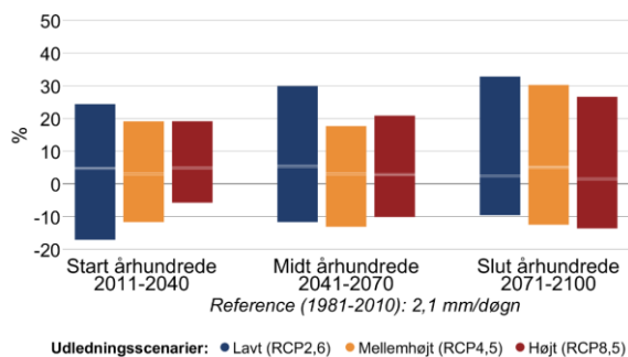
Figur 6 Procentvis ændring af middelnedbør mellem 1981-2010 og fremtidsperioderne 2011-2040, 2041-2070 og 2071-2100 under forskellige udledningsscenarier i Holbæk Kommune. Til venstre sommer (jun-aug), til højre vinter (dec-feb).
