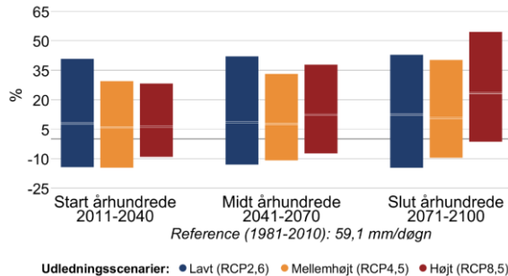
Figur 7 Procentvis ændring af ekstremnedbør hen over året mellem 1981-2010 og fremtidsperioderne 2011-2040, 2041-2070 og 2071-2100 under forskellige udledningsscenarier i Holbæk Kommune. Til venstre 10-årshændelsen for døgnnedbør, til højre frekvensen af skybrud.
