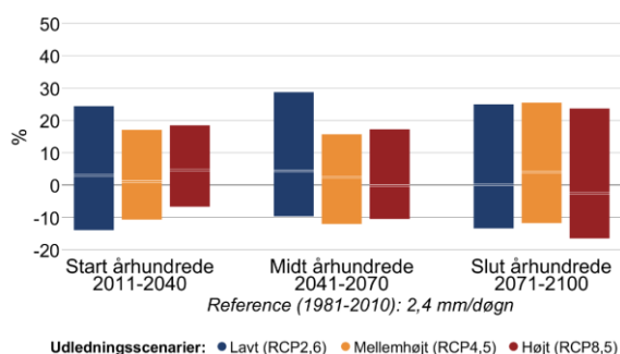
Figur 6 Procentvis ændring af middelnedbør mellem 1981-2010 og fremtidsperioderne 2011-2040, 2041-2070 og 2071-2100 under forskellige udledningsscenarier i Hjørring Kommune. Til venstre sommer (jun-aug), til højre vinter (dec-feb).
