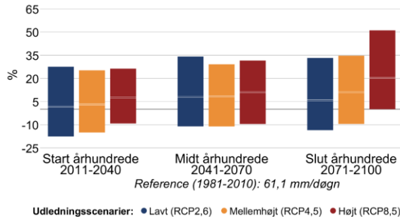
Figur 7 Procentvis ændring af ekstremnedbør hen over året mellem 1981-2010 og fremtidsperioderne 2011-2040, 2041-2070 og 2071-2100 under forskellige udledningsscenarier i Hjørring Kommune. Til venstre 10-årshændelsen for døgnnedbør, til højre frekvensen af skybrud.
