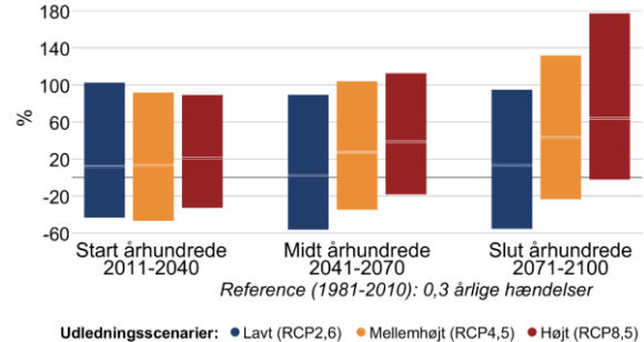
Figur 7 Procentvis ændring af ekstremnedbør hen over året mellem 1981-2010 og fremtidsperioderne 2011-2040, 2041-2070 og 2071-2100 under forskellige udledningsscenarier i Hjørring Kommune. Til venstre 10-årshændelsen for døgnnedbør, til højre frekvensen af skybrud.
