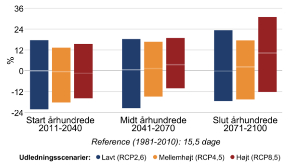
Figur 8 Procentvis ændring af tørre dage om sommeren (jun-aug) mellem 1981-2010 og fremtidsperioderne 2011-2040, 2041-2070 og 2071-2100 under forskellige udledningsscenarier i Hjørring Kommune. Til venstre antallet af tørre dage med mindre end 1 mm nedbør, til højre længden af den længste sammenhængende tørre periode.
