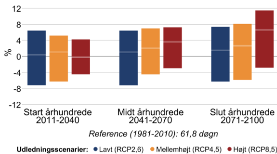
Figur 8 Procentvis ændring af tørre dage om sommeren (jun-aug) mellem 1981-2010 og fremtidsperioderne 2011-2040, 2041-2070 og 2071-2100 under forskellige udledningsscenarier i Hjørring Kommune. Til venstre antallet af tørre dage med mindre end 1 mm nedbør, til højre længden af den længste sammenhængende tørre periode.
