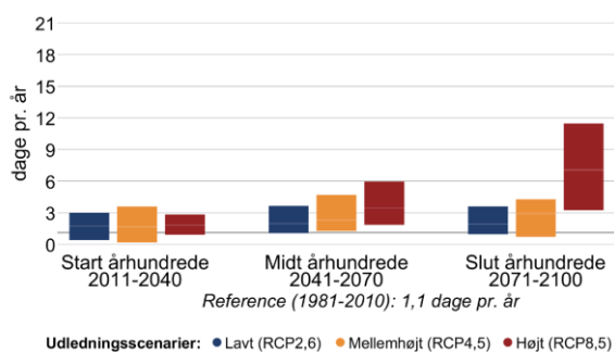
Figur 3 Ændring af gennemsnitstemperatur og antallet af hedebølgedage hen over året mellem 1981-2010 og fremtidsperioderne 2011-2040, 2041-2070 og 2071-2100 under forskellige udledningsscenarier i Hjørring Kommune.
