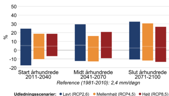
Figur 6 Procentvis ændring af middelnedbør mellem 1981-2010 og fremtidsperioderne 2011-2040, 2041-2070 og 2071-2100 under forskellige udledningsscenarier i Hillerød Kommune. Til venstre sommer (jun-aug), til højre vinter (dec-feb).
