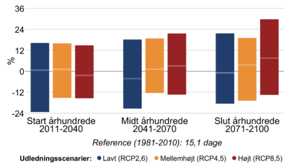
Figur 8 Procentvis ændring af tørre dage om sommeren (jun-aug) mellem 1981-2010 og fremtidsperioderne 2011-2040, 2041-2070 og 2071-2100 under forskellige udledningsscenarier i Hillerød Kommune. Til venstre antallet af tørre dage med mindre end 1 mm nedbør, til højre længden af den længste sammenhængende tørre periode.
