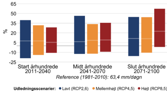
Figur 7 Procentvis ændring af ekstremnedbør hen over året mellem 1981-2010 og fremtidsperioderne 2011-2040, 2041-2070 og 2071-2100 under forskellige udledningsscenarier i Hillerød Kommune. Til venstre 10-årshændelsen for døgnnedbør, til højre frekvensen af skybrud.
