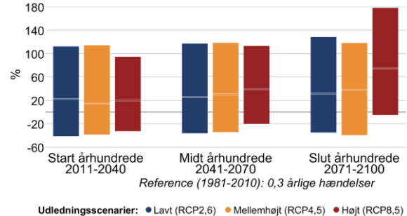
Figur 7 Procentvis ændring af ekstremnedbør hen over året mellem 1981-2010 og fremtidsperioderne 2011-2040, 2041-2070 og 2071-2100 under forskellige udledningsscenarier i Hillerød Kommune. Til venstre 10-årshændelsen for døgnnedbør, til højre frekvensen af skybrud.
