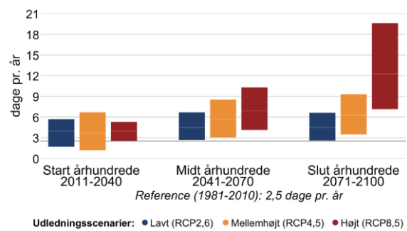
Figur 3 Ændring af gennemsnitstemperatur og antallet af hedebløgedage hen over året mellem 1981-2010 og fremtidsperioderne 2011-2040, 2041-2070 og 2071-2100 under forskellige udledningsscenarier i Hillerød Kommune.
