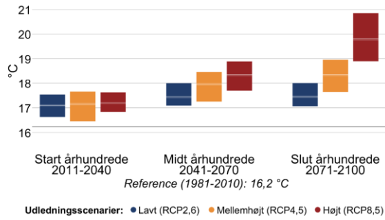
Figur 4 Gennemsnitstemperatur for sommer (jun-aug) og vinter (dec-feb) i fremtidsperioderne 2011-2040, 2041-2070 og 2071-2100 under forskellige udledningsscenarier i Hillerød Kommune. Den grå linje viser referenceværdien for nutiden (1981-2010).
