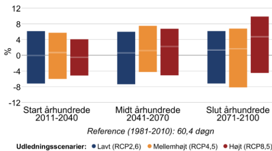
Figur 8 Procentvis ændring af tørre dage om sommeren (jun-aug) mellem 1981-2010 og fremtidsperioderne 2011-2040, 2041-2070 og 2071-2100 under forskellige udledningsscenarier i Hillerød Kommune. Til venstre antallet af tørre dage med mindre end 1 mm nedbør, til højre længden af den længste sammenhængende tørre periode.
