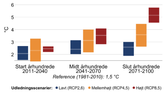
Figur 4 Gennemsnitstemperatur for sommer (jun-aug) og vinter (dec-feb) i fremtidsperioderne 2011-2040, 2041-2070 og 2071-2100 under forskellige udledningsscenarier i Halsnæs Kommune. Den grå linje viser referenceværdien for nutiden (1981-2010).
