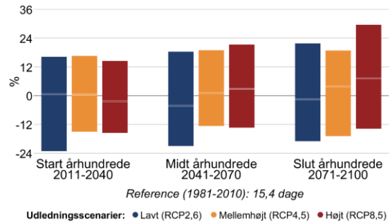
Figur 8 Procentvis ændring af tørre dage om sommeren (jun-aug) mellem 1981-2010 og fremtidsperioderne 2011-2040, 2041-2070 og 2071-2100 under forskellige udledningsscenarier i Halsnæs Kommune. Til venstre antallet af tørre dage med mindre end 1 mm nedbør, til højre længden af den længste sammenhængende tørre periode.
