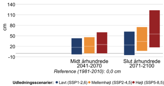
Figur 12 Ændring i middelvandstand (venstre) og hyppigheden af stormflod for Isefjord i fremtidsperioderne 2041-2070 og 2071-2100 under forskellige udledningsscenarier. Den grå linje viser referenceværdien for nutiden (1981-2010). En stormflod defineres her som en forhøjet vandstand, der statistisk set kun forekommer én gang hvert 20. år i perioden 1981-2010. Bemærk også at denne indikator kappes ved 60 stormfloder per 20 år.
