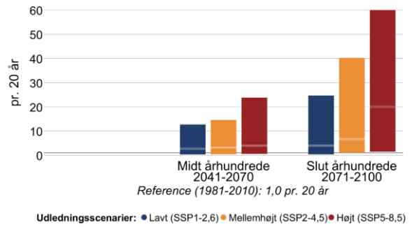
Figur 14 Ændring i middelvandstand (venstre) og hyppigheden af stormflod for Roskilde Fjord i fremtidsperioderne 2041-2070 og 2071-2100 under forskellige udledningsscenarier. Den grå linje viser referenceværdien for nutiden (1981-2010). En stormflod defineres her som en forhøjet vandstand, der statistisk set kun forekommer én gang hvert 20. år i perioden 1981-2010. Bemærk også at denne indikator kappes ved 60 stormfloder per 20 år.
