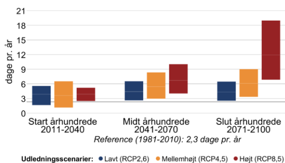
Figur 3 Ændring af gennemsnitstemperatur og antallet af hedebølgedage hen over året mellem 1981-2010 og fremtidsperioderne 2011-2040, 2041-2070 og 2071-2100 under forskellige udledningsscenarier i Halsnæs Kommune.
