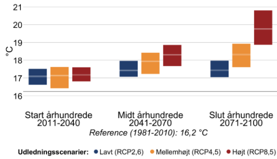
Figur 4 Gennemsnitstemperatur for sommer (jun-aug) og vinter (dec-feb) i fremtidsperioderne 2011-2040, 2041-2070 og 2071-2100 under forskellige udledningsscenarier i Halsnæs Kommune. Den grå linje viser referenceværdien for nutiden (1981-2010).
