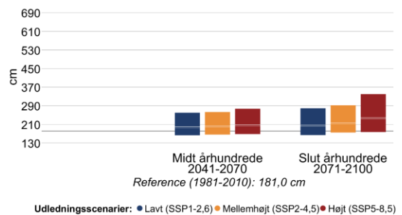
Figur 13 Højden af 20- (venstre) og 100-års (højre) stormflodhændelser for Isefjord i fremtidsperioderne 2041-2070 og 2071-2100 under forskellige udledningsscenarier. Den grå linje viser referenceværdien for nutiden (1981-2010).
