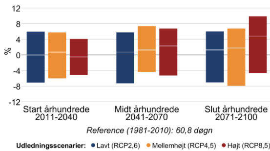
Figur 8 Procentvis ændring af tørre dage om sommeren (jun-aug) mellem 1981-2010 og fremtidsperioderne 2011-2040, 2041-2070 og 2071-2100 under forskellige udledningsscenarier i Halsnæs Kommune. Til venstre antallet af tørre dage med mindre end 1 mm nedbør, til højre længden af den længste sammenhængende tørre periode.
