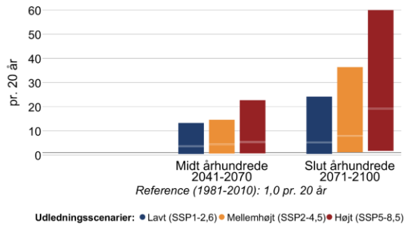
Figur 12 Ændring i middelvandstand (venstre) og hyppigheden af stormflod for Isefjord i fremtidsperioderne 2041-2070 og 2071-2100 under forskellige udledningsscenarier. Den grå linje viser referenceværdien for nutiden (1981-2010). En stormflod defineres her som en forhøjet vandstand, der statistisk set kun forekommer én gang hvert 20. år i perioden 1981-2010. Bemærk også at denne indikator kappes ved 60 stormfloder per 20 år.
