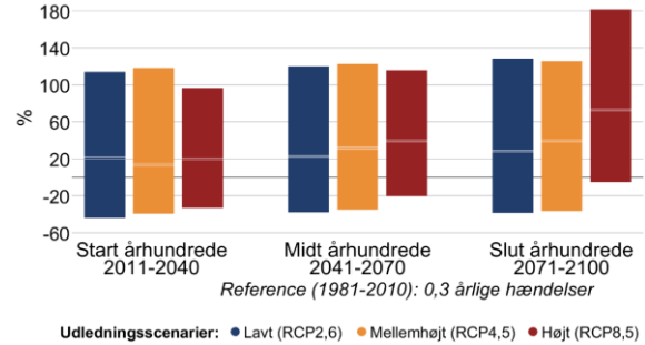
Figur 7 Procentvis ændring af ekstremnedbør hen over året mellem 1981-2010 og fremtidsperioderne 2011-2040, 2041-2070 og 2071-2100 under forskellige udledningsscenarier i Halsnæs Kommune. Til venstre 10-årshændelsen for døgnnedbør, til højre frekvensen af skybrud.
