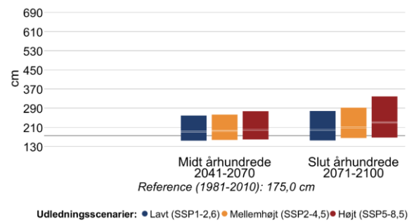
Figur 15 Højden af 20- (venstre) og 100-års (højre) stormflodhændelser for Roskilde Fjord i fremtidsperioderne 2041-2070 og 2071-2100 under forskellige udledningsscenarier. Den grå linje viser referenceværdien for nutiden (1981-2010).
