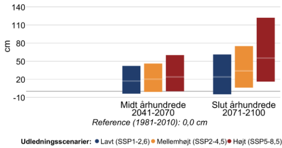
Figur 14 Ændring i middelvandstand (venstre) og hyppigheden af stormflod for Roskilde Fjord i fremtidsperioderne 2041-2070 og 2071-2100 under forskellige udledningsscenarier. Den grå linje viser referenceværdien for nutiden (1981-2010). En stormflod defineres her som en forhøjet vandstand, der statistisk set kun forekommer én gang hvert 20. år i perioden 1981-2010. Bemærk også at denne indikator kappes ved 60 stormfloder per 20 år.
