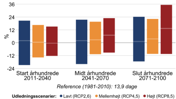
Figur 8 Procentvis ændring af tørre dage om sommeren (jun-aug) mellem 1981-2010 og fremtidsperioderne 2011-2040, 2041-2070 og 2071-2100 under forskellige udledningsscenarier i Haderslev Kommune. Til venstre antallet af tørre dage med mindre end 1 mm nedbør, til højre længden af den længste sammenhængende tørre periode.
