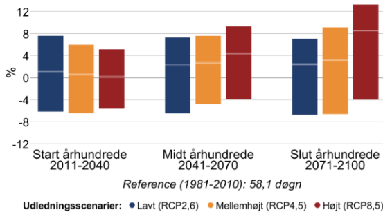
Figur 8 Procentvis ændring af tørre dage om sommeren (jun-aug) mellem 1981-2010 og fremtidsperioderne 2011-2040, 2041-2070 og 2071-2100 under forskellige udledningsscenarier i Haderslev Kommune. Til venstre antallet af tørre dage med mindre end 1 mm nedbør, til højre længden af den længste sammenhængende tørre periode.
