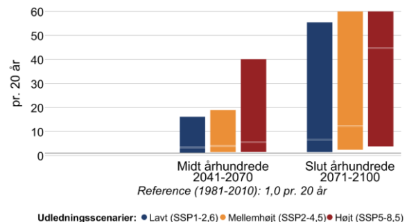
Figur 10 Ændring i middelvandstand (venstre) og hyppigheden af stormflod for Lillebælt sydlig i fremtidsperioderne 2041-2070 og 2071-2100 under forskellige udledningsscenarier. Den grå linje viser referenceværdien for nutiden (1981-2010). En stormflod defineres her som en forhøjet vandstand, der statistisk set kun forekommer én gang hvert 20. år i perioden 1981-2010. Bemærk også at denne indikator kappes ved 60 stormfloder per 20 år.
