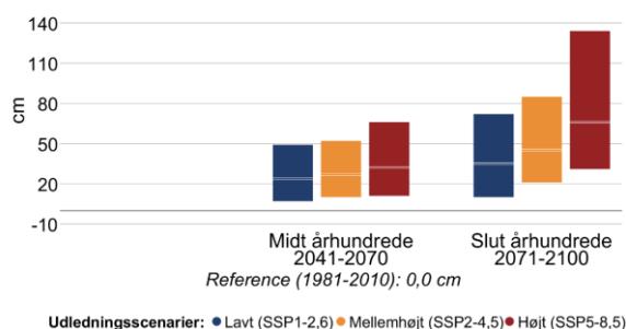
Figur 10 Ændring i middelvandstand (venstre) og hyppigheden af stormflod for Lillebælt sydlig i fremtidsperioderne 2041-2070 og 2071-2100 under forskellige udledningsscenarier. Den grå linje viser referenceværdien for nutiden (1981-2010). En stormflod defineres her som en forhøjet vandstand, der statistisk set kun forekommer én gang hvert 20. år i perioden 1981-2010. Bemærk også at denne indikator kappes ved 60 stormfloder per 20 år.
