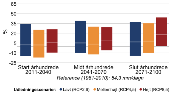
Figur 7 Procentvis ændring af ekstremnedbør hen over året mellem 1981-2010 og fremtidsperioderne 2011-2040, 2041-2070 og 2071-2100 under forskellige udledningsscenarier i Haderslev Kommune. Til venstre 10-årshændelsen for døgnnedbør, til højre frekvensen af skybrud.
