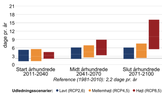
Figur 3 Ændring af gennemsnitstemperatur og antallet af hedebølgedage hen over året mellem 1981-2010 og fremtidsperioderne 2011-2040, 2041-2070 og 2071-2100 under forskellige udledningsscenarier i Haderslev Kommune.
