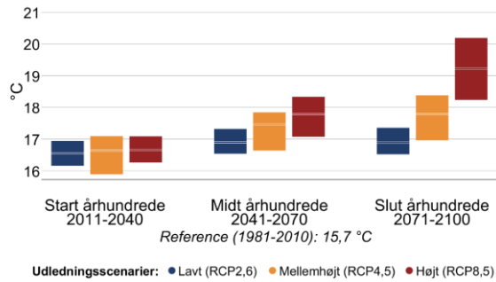
Figur 4 Gennemsnitstemperatur for sommer (jun-aug) og vinter (dec-feb) i fremtidsperioderne 2011-2040, 2041-2070 og 2071-2100 under forskellige udledningsscenarier i Haderslev Kommune. Den grå linje viser referenceværdien for nutiden (1981-2010).
