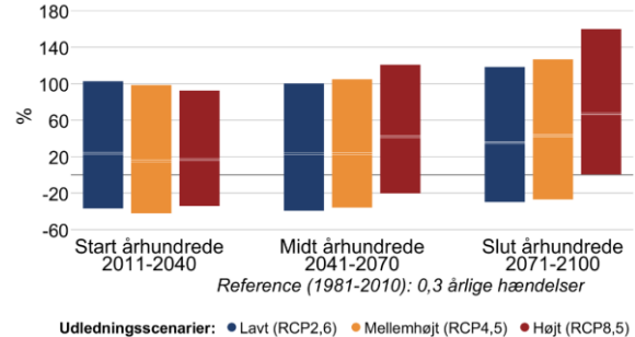
Figur 7 Procentvis ændring af ekstremnedbør hen over året mellem 1981-2010 og fremtidsperioderne 2011-2040, 2041-2070 og 2071-2100 under forskellige udledningsscenarier i Haderslev Kommune. Til venstre 10-årshændelsen for døgnnedbør, til højre frekvensen af skybrud.
