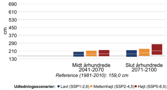
Figur 11 Højden af 20- (venstre) og 100-års (højre) stormflodhændelser for Nordsjællands kyst i fremtidsperioderne 2041-2070 og 2071-2100 under forskellige udledningsscenarier. Den grå linje viser referenceværdien for nutiden (1981-2010).
