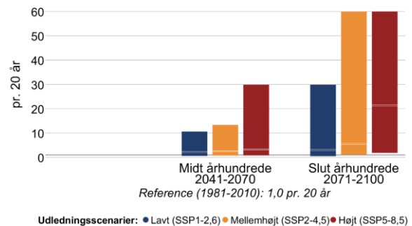
Figur 10 Ændring i middelvandstand (venstre) og hyppigheden af stormflod for Nordsjællands kyst i fremtidsperioderne 2041-2070 og 2071-2100 under forskellige udledningsscenarier. Den grå linje viser referenceværdien for nutiden (1981-2010). En stormflod defineres her som en forhøjet vandstand, der statistisk set kun forekommer én gang hvert 20. år i perioden 1981-2010. Bemærk også at denne indikator kappes ved 60 stormfloder per 20 år.
