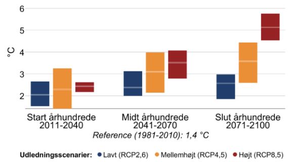
Figur 4 Gennemsnitstemperatur for sommer (jun-aug) og vinter (dec-feb) i fremtidsperioderne 2011-2040, 2041-2070 og 2071-2100 under forskellige udledningsscenarier i Gribskov Kommune. Den grå linje viser referenceværdien for nutiden (1981-2010).
