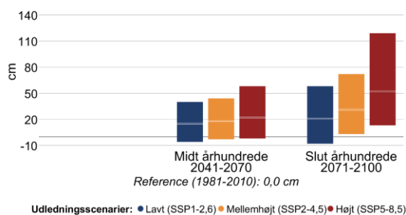
Figur 10 Ændring i middelvandstand (venstre) og hyppigheden af stormflod for Nordsjællands kyst i fremtidsperioderne 2041-2070 og 2071-2100 under forskellige udledningsscenarier. Den grå linje viser referenceværdien for nutiden (1981-2010). En stormflod defineres her som en forhøjet vandstand, der statistisk set kun forekommer én gang hvert 20. år i perioden 1981-2010. Bemærk også at denne indikator kappes ved 60 stormfloder per 20 år.
