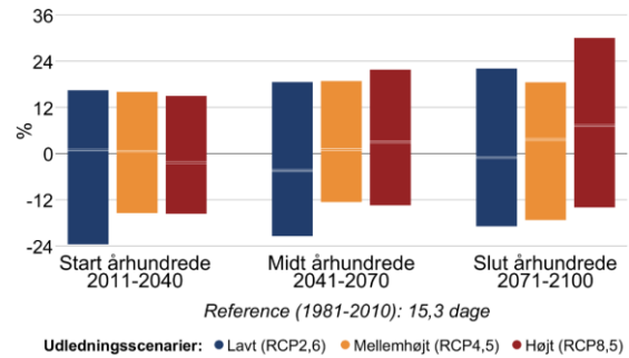
Figur 8 Procentvis ændring af tørre dage om sommeren (jun-aug) mellem 1981-2010 og fremtidsperioderne 2011-2040, 2041-2070 og 2071-2100 under forskellige udledningsscenarier i Gribskov Kommune. Til venstre antallet af tørre dage med mindre end 1 mm nedbør, til højre længden af den længste sammenhængende tørre periode.
