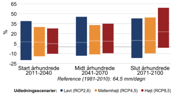
Figur 7 Procentvis ændring af ekstremnedbør hen over året mellem 1981-2010 og fremtidsperioderne 2011-2040, 2041-2070 og 2071-2100 under forskellige udledningsscenarier i Gribskov Kommune. Til venstre 10-årshændelsen for døgnnedbør, til højre frekvensen af skybrud.
