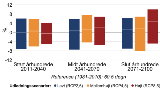
Figur 8 Procentvis ændring af tørre dage om sommeren (jun-aug) mellem 1981-2010 og fremtidsperioderne 2011-2040, 2041-2070 og 2071-2100 under forskellige udledningsscenarier i Gribskov Kommune. Til venstre antallet af tørre dage med mindre end 1 mm nedbør, til højre længden af den længste sammenhængende tørre periode.
