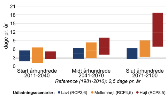
Figur 3 Ændring af gennemsnitstemperatur og antallet af hedebløgedage hen over året mellem 1981-2010 og fremtidsperioderne 2011-2040, 2041-2070 og 2071-2100 under forskellige udledningsscenarier i Gribskov Kommune.
