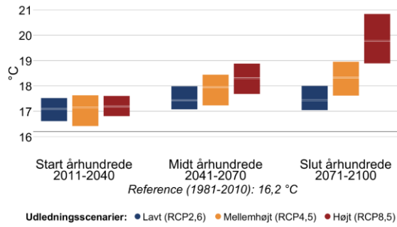
Figur 4 Gennemsnitstemperatur for sommer (jun-aug) og vinter (dec-feb) i fremtidsperioderne 2011-2040, 2041-2070 og 2071-2100 under forskellige udledningsscenarier i Gribskov Kommune. Den grå linje viser referenceværdien for nutiden (1981-2010).
