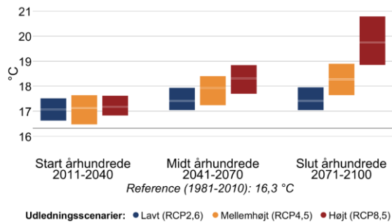
Figur 4 Gennemsnitstemperatur for sommer (jun-aug) og vinter (dec-feb) i fremtidsperioderne 2011-2040, 2041-2070 og 2071-2100 under forskellige udledningsscenarier i Greve Kommune. Den grå linje viser referenceværdien for nutiden (1981-2010).
