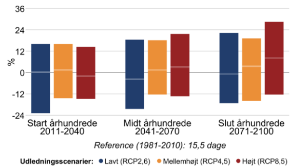
Figur 8 Procentvis ændring af tørre dage om sommeren (jun-aug) mellem 1981-2010 og fremtidsperioderne 2011-2040, 2041-2070 og 2071-2100 under forskellige udledningsscenarier i Greve Kommune. Til venstre antallet af tørre dage med mindre end 1 mm nedbør, til højre længden af den længste sammenhængende tørre periode.
