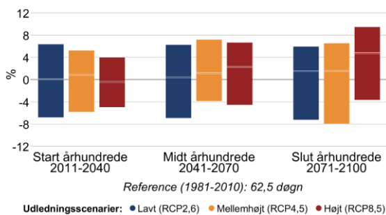
Figur 8 Procentvis ændring af tørre dage om sommeren (jun-aug) mellem 1981-2010 og fremtidsperioderne 2011-2040, 2041-2070 og 2071-2100 under forskellige udledningsscenarier i Greve Kommune. Til venstre antallet af tørre dage med mindre end 1 mm nedbør, til højre længden af den længste sammenhængende tørre periode.
