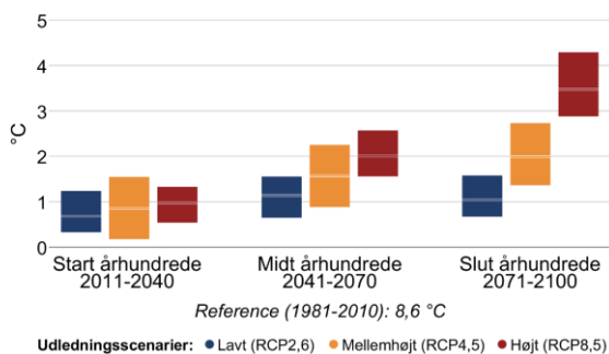
Figur 3 Ændring af gennemsnitstemperatur og antallet af hedebløgedage hen over året mellem 1981-2010 og fremtidsperioderne 2011-2040, 2041-2070 og 2071-2100 under forskellige udledningsscenarier i Greve Kommune.
