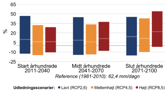
Figur 7 Procentvis ændring af ekstremnedbør hen over året mellem 1981-2010 og fremtidsperioderne 2011-2040, 2041-2070 og 2071-2100 under forskellige udledningsscenarier i Greve Kommune. Til venstre 10-årshændelsen for døgnnedbør, til højre frekvensen af skybrud.
