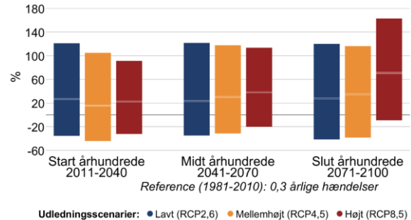
Figur 7 Procentvis ændring af ekstremnedbør hen over året mellem 1981-2010 og fremtidsperioderne 2011-2040, 2041-2070 og 2071-2100 under forskellige udledningsscenarier i Greve Kommune. Til venstre 10-årshændelsen for døgnnedbør, til højre frekvensen af skybrud.
