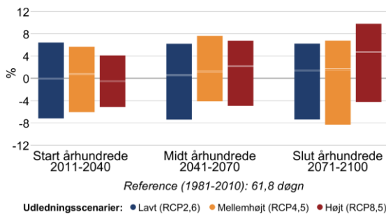
Figur 8 Procentvis ændring af tørre dage om sommeren (jun-aug) mellem 1981-2010 og fremtidsperioderne 2011-2040, 2041-2070 og 2071-2100 under forskellige udledningsscenarier i Gentofte Kommune. Til venstre antallet af tørre dage med mindre end 1 mm nedbør, til højre længden af den længste sammenhængende tørre periode.
