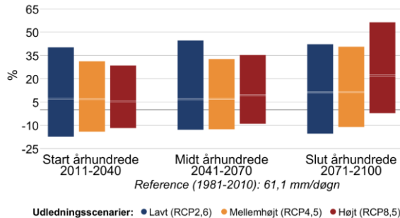
Figur 7 Procentvis ændring af ekstremnedbør hen over året mellem 1981-2010 og fremtidsperioderne 2011-2040, 2041-2070 og 2071-2100 under forskellige udledningsscenarier i Gentofte Kommune. Til venstre 10-årshændelsen for døgnnedbør, til højre frekvensen af skybrud.
