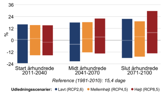
Figur 8 Procentvis ændring af tørre dage om sommeren (jun-aug) mellem 1981-2010 og fremtidsperioderne 2011-2040, 2041-2070 og 2071-2100 under forskellige udledningsscenarier i Gentofte Kommune. Til venstre antallet af tørre dage med mindre end 1 mm nedbør, til højre længden af den længste sammenhængende tørre periode.
