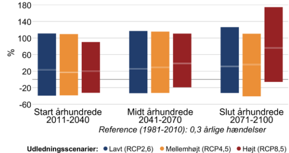
Figur 7 Procentvis ændring af ekstremnedbør hen over året mellem 1981-2010 og fremtidsperioderne 2011-2040, 2041-2070 og 2071-2100 under forskellige udledningsscenarier i Gentofte Kommune. Til venstre 10-årshændelsen for døgnnedbør, til højre frekvensen af skybrud.
