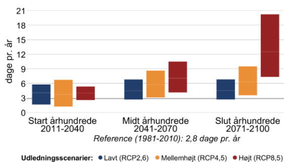
Figur 3 Ændring af gennemsnitstemperatur og antallet af hedebløgedage hen over året mellem 1981-2010 og fremtidsperioderne 2011-2040, 2041-2070 og 2071-2100 under forskellige udledningsscenarier i Gentofte Kommune.
