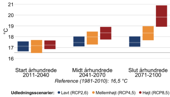
Figur 4 Gennemsnitstemperatur for sommer (jun-aug) og vinter (dec-feb) i fremtidsperioderne 2011-2040, 2041-2070 og 2071-2100 under forskellige udledningsscenarier i Gentofte Kommune. Den grå linje viser referenceværdien for nutiden (1981-2010).
