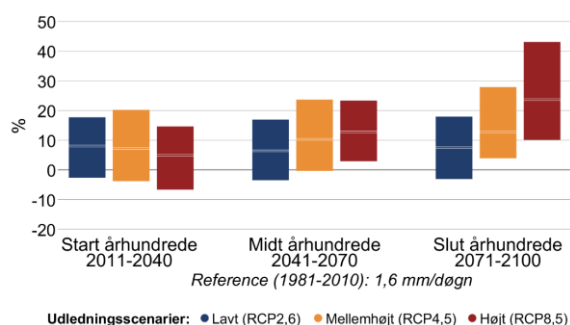
Figur 6 Procentvis ændring af middelnedbør mellem 1981-2010 og fremtidsperioderne 2011-2040, 2041-2070 og 2071-2100 under forskellige udledningsscenarier i Gentofte Kommune. Til venstre sommer (jun-aug), til højre vinter (dec-feb).
