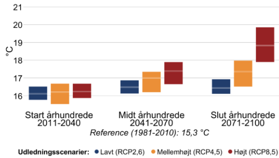
Figur 4 Gennemsnitstemperatur for sommer (jun-aug) og vinter (dec-feb) i fremtidsperioderne 2011-2040, 2041-2070 og 2071-2100 under forskellige udledningsscenarier i Favrskov Kommune. Den grå linje viser referenceværdien for nutiden (1981-2010).
