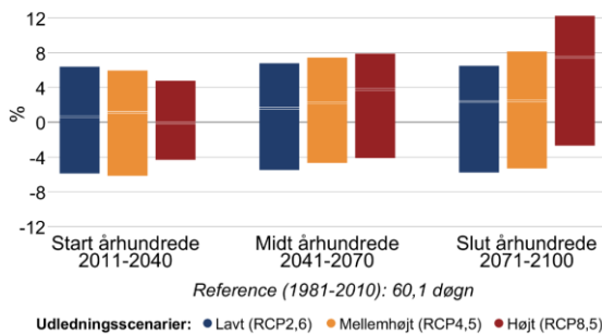
Figur 8 Procentvis ændring af tørre dage om sommeren (jun-aug) mellem 1981-2010 og fremtidsperioderne 2011-2040, 2041-2070 og 2071-2100 under forskellige udledningsscenarier i Favrskov Kommune. Til venstre antallet af tørre dage med mindre end 1 mm nedbør, til højre længden af den længste sammenhængende tørre periode.
