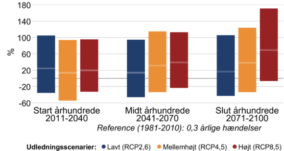
Figur 7 Procentvis ændring af ekstremnedbør hen over året mellem 1981-2010 og fremtidsperioderne 2011-2040, 2041-2070 og 2071-2100 under forskellige udledningsscenarier i Favrskov Kommune. Til venstre 10-årshændelsen for døgnnedbør, til højre frekvensen af skybrud.
