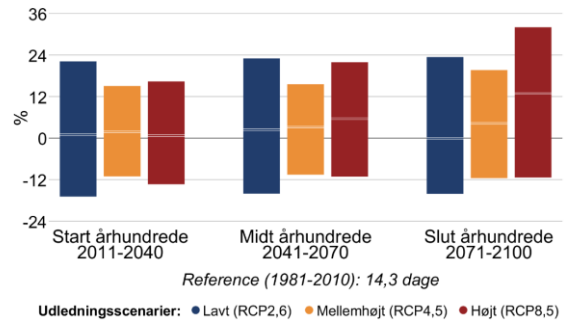
Figur 8 Procentvis ændring af tørre dage om sommeren (jun-aug) mellem 1981-2010 og fremtidsperioderne 2011-2040, 2041-2070 og 2071-2100 under forskellige udledningsscenarier i Favrskov Kommune. Til venstre antallet af tørre dage med mindre end 1 mm nedbør, til højre længden af den længste sammenhængende tørre periode.
