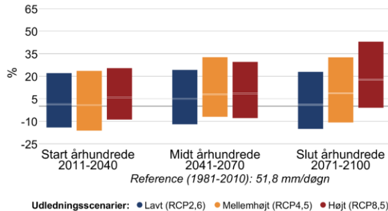
Figur 7 Procentvis ændring af ekstremnedbør hen over året mellem 1981-2010 og fremtidsperioderne 2011-2040, 2041-2070 og 2071-2100 under forskellige udledningsscenarier i Favrskov Kommune. Til venstre 10-årshændelsen for døgnnedbør, til højre frekvensen af skybrud.
