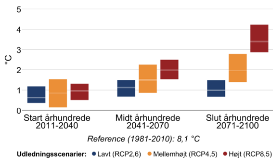
Figur 3 Ændring af gennemsnitstemperatur og antallet af hedebølgedage hen over året mellem 1981-2010 og fremtidsperioderne 2011-2040, 2041-2070 og 2071-2100 under forskellige udledningsscenarier i Favrskov Kommune.
