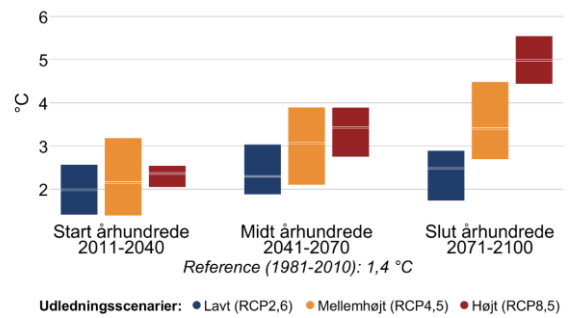
Figur 4 Gennemsnitstemperatur for sommer (jun-aug) og vinter (dec-feb) i fremtidsperioderne 2011-2040, 2041-2070 og 2071-2100 under forskellige udledningsscenarier i Favrskov Kommune. Den grå linje viser referenceværdien for nutiden (1981-2010).
