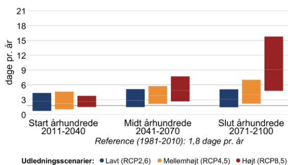
Figur 3 Ændring af gennemsnitstemperatur og antallet af hedebølgedage hen over året mellem 1981-2010 og fremtidsperioderne 2011-2040, 2041-2070 og 2071-2100 under forskellige udledningsscenarier i Faaborg-Midtfyn Kommune.
