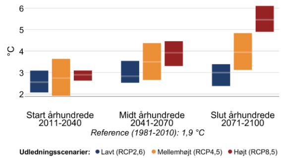
Figur 4 Gennemsnitstemperatur for sommer (jun-aug) og vinter (dec-feb) i fremtidsperioderne 2011-2040, 2041-2070 og 2071-2100 under forskellige udledningsscenarier i Faaborg-Midtfyn Kommune. Den grå linje viser referenceværdien for nutiden (1981-2010).
