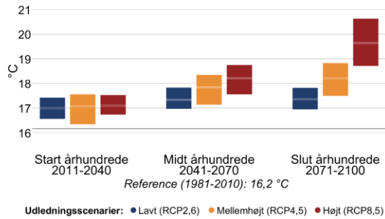
Figur 4 Gennemsnitstemperatur for sommer (jun-aug) og vinter (dec-feb) i fremtidsperioderne 2011-2040, 2041-2070 og 2071-2100 under forskellige udledningsscenarier i Faaborg-Midtfyn Kommune. Den grå linje viser referenceværdien for nutiden (1981-2010).
