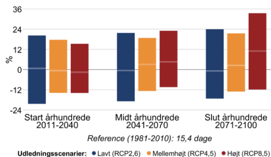
Figur 8 Procentvis ændring af tørre dage om sommeren (jun-aug) mellem 1981-2010 og fremtidsperioderne 2011-2040, 2041-2070 og 2071-2100 under forskellige udledningsscenarier i Faaborg-Midtfyn Kommune. Til venstre antallet af tørre dage med mindre end 1 mm nedbør, til højre længden af den længste sammenhængende tørre periode.
