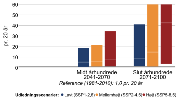
Figur 12 Ændring i middelvandstand (venstre) og hyppigheden af stormflod for Sydfynske Øhav i fremtidsperioderne 2041-2070 og 2071-2100 under forskellige udledningsscenarier. Den grå linje viser referenceværdien for nutiden (1981-2010). En stormflod defineres her som en forhøjet vandstand, der statistisk set kun forekommer én gang hvert 20. år i perioden 1981-2010. Bemærk også at denne indikator kappes ved 60 stormfloder per 20 år.
