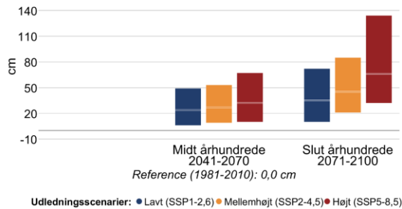
Figur 12 Ændring i middelvandstand (venstre) og hyppigheden af stormflod for Sydfynske Øhav i fremtidsperioderne 2041-2070 og 2071-2100 under forskellige udledningsscenarier. Den grå linje viser referenceværdien for nutiden (1981-2010). En stormflod defineres her som en forhøjet vandstand, der statistisk set kun forekommer én gang hvert 20. år i perioden 1981-2010. Bemærk også at denne indikator kappes ved 60 stormfloder per 20 år.
