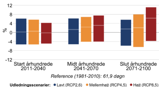
Figur 8 Procentvis ændring af tørre dage om sommeren (jun-aug) mellem 1981-2010 og fremtidsperioderne 2011-2040, 2041-2070 og 2071-2100 under forskellige udledningsscenarier i Faaborg-Midtfyn Kommune. Til venstre antallet af tørre dage med mindre end 1 mm nedbør, til højre længden af den længste sammenhængende tørre periode.
