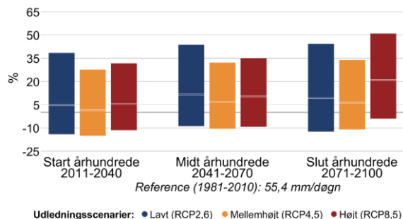
Figur 7 Procentvis ændring af ekstremnedbør hen over året mellem 1981-2010 og fremtidsperioderne 2011-2040, 2041-2070 og 2071-2100 under forskellige udledningsscenarier i Faaborg-Midtfyn Kommune. Til venstre 10-årshændelsen for døgnnedbør, til højre frekvensen af skybrud.
