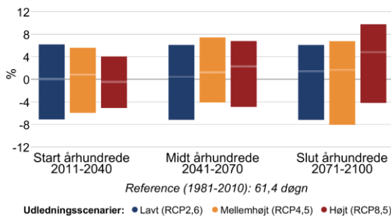
Figur 8 Procentvis ændring af tørre dage om sommeren (jun-aug) mellem 1981-2010 og fremtidsperioderne 2011-2040, 2041-2070 og 2071-2100 under forskellige udledningsscenarier i Egedal Kommune. Til venstre antallet af tørre dage med mindre end 1 mm nedbør, til højre længden af den længste sammenhængende tørre periode.
