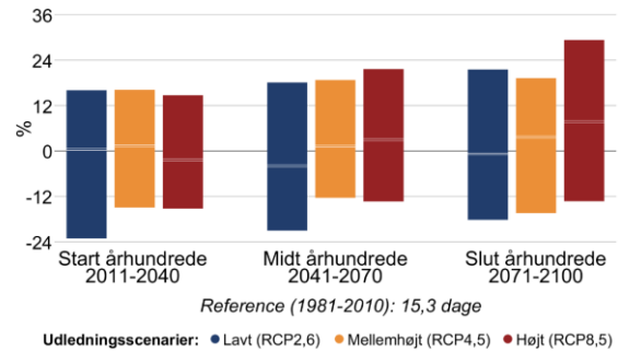
Figur 8 Procentvis ændring af tørre dage om sommeren (jun-aug) mellem 1981-2010 og fremtidsperioderne 2011-2040, 2041-2070 og 2071-2100 under forskellige udledningsscenarier i Egedal Kommune. Til venstre antallet af tørre dage med mindre end 1 mm nedbør, til højre længden af den længste sammenhængende tørre periode.
