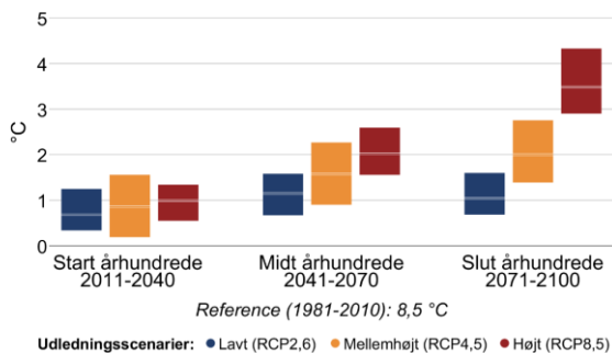
Figur 3 Ændring af gennemsnitstemperatur og antallet af hedebløgedage hen over året mellem 1981-2010 og fremtidsperioderne 2011-2040, 2041-2070 og 2071-2100 under forskellige udledningsscenarier i Egedal Kommune.
