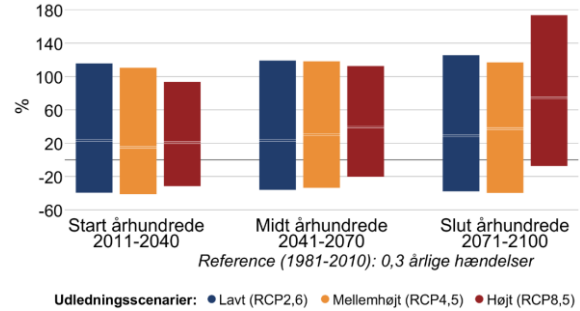
Figur 7 Procentvis ændring af ekstremnedbør hen over året mellem 1981-2010 og fremtidsperioderne 2011-2040, 2041-2070 og 2071-2100 under forskellige udledningsscenarier i Egedal Kommune. Til venstre 10-årshændelsen for døgnnedbør, til højre frekvensen af skybrud.
