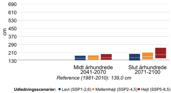
Figur 11 Højden af 20- (venstre) og 100-års (højre) stormflodhændelser for Kattegatkyst nordlige i fremtidsperioderne 2041-2070 og 2071-2100 under forskellige udledningsscenarier. Den grå linje viser referenceværdien for nutiden (1981-2010).
