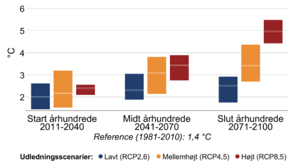
Figur 4 Gennemsnitstemperatur for sommer (jun-aug) og vinter (dec-feb) i fremtidsperioderne 2011-2040, 2041-2070 og 2071-2100 under forskellige udledningsscenarier i Brønderslev Kommune. Den grå linje viser referenceværdien for nutiden (1981-2010).
