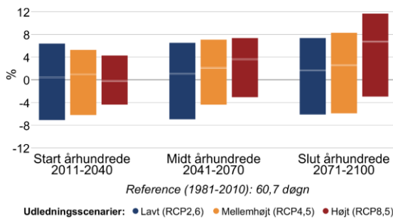
Figur 8 Procentvis ændring af tørre dage om sommeren (jun-aug) mellem 1981-2010 og fremtidsperioderne 2011-2040, 2041-2070 og 2071-2100 under forskellige udledningsscenarier i Brønderslev Kommune. Til venstre antallet af tørre dage med mindre end 1 mm nedbør, til højre længden af den længste sammenhængende tørre periode.
