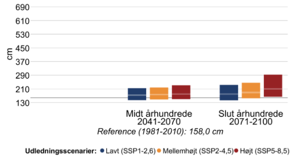
Figur 11 Højden af 20- (venstre) og 100-års (højre) stormflodhændelser for Kattegatkyst nordlige i fremtidsperioderne 2041-2070 og 2071-2100 under forskellige udledningsscenarier. Den grå linje viser referenceværdien for nutiden (1981-2010).
