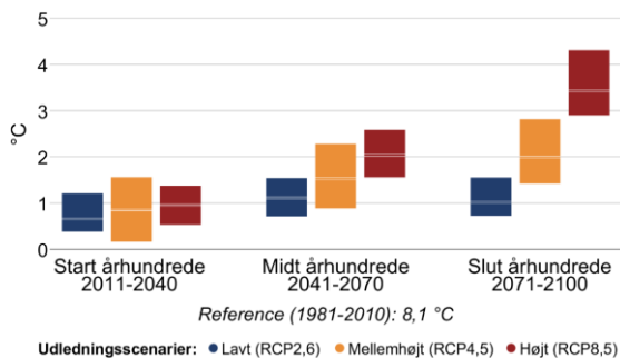
Figur 3 Ændring af gennemsnitstemperatur og antallet af hedebølgedage hen over året mellem 1981-2010 og fremtidsperioderne 2011-2040, 2041-2070 og 2071-2100 under forskellige udledningsscenarier i Brønderslev Kommune.
