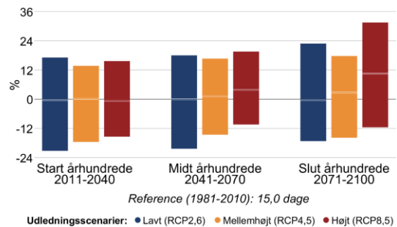
Figur 8 Procentvis ændring af tørre dage om sommeren (jun-aug) mellem 1981-2010 og fremtidsperioderne 2011-2040, 2041-2070 og 2071-2100 under forskellige udledningsscenarier i Brønderslev Kommune. Til venstre antallet af tørre dage med mindre end 1 mm nedbør, til højre længden af den længste sammenhængende tørre periode.
