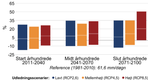
Figur 7 Procentvis ændring af ekstremnedbør hen over året mellem 1981-2010 og fremtidsperioderne 2011-2040, 2041-2070 og 2071-2100 under forskellige udledningsscenarier i Brønderslev Kommune. Til venstre 10-årshændelsen for døgnnedbør, til højre frekvensen af skybrud.
