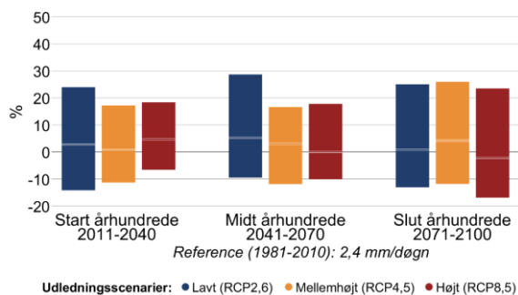
Figur 6 Procentvis ændring af middelnedbør mellem 1981-2010 og fremtidsperioderne 2011-2040, 2041-2070 og 2071-2100 under forskellige udledningsscenerier i Brønderslev Kommune. Til venstre sommer (jun-aug), til højre vinter (dec-feb).
