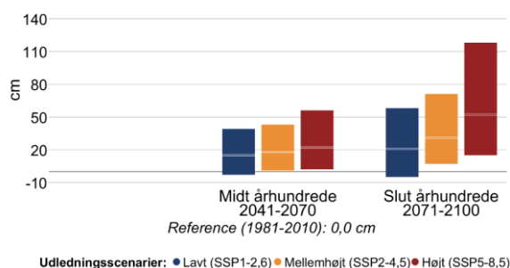
Figur 10 Ændring i middelvandstand (venstre) og hyppigheden af stormflod for Kattegatkyst nordlige i fremtidsperioderne 2041-2070 og 2071-2100 under forskellige udledningsscenarioer. Den grå linje viser referenceværdien for nutiden (1981-2010). En stormflod defineres her som en forhøjet vandstand, der statistisk set kun forekommer én gang hvert 20. år i perioden 1981-2010. Bemærk også at denne indikator kappes ved 60 stormfloder per 20 år.
