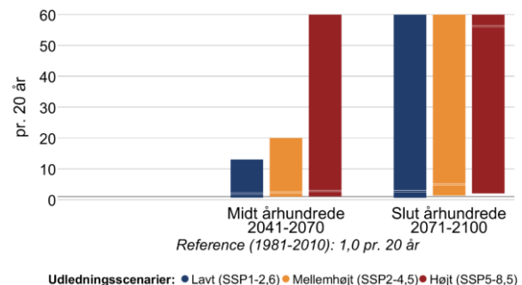
Figur 10 Ændring i middelvandstand (venstre) og hyppigheden af stormflod for Kattegatkyst nordlige i fremtidsperioderne 2041-2070 og 2071-2100 under forskellige udledningsscenarioer. Den grå linje viser referenceværdien for nutiden (1981-2010). En stormflod defineres her som en forhøjet vandstand, der statistisk set kun forekommer én gang hvert 20. år i perioden 1981-2010. Bemærk også at denne indikator kappes ved 60 stormfloder per 20 år.
