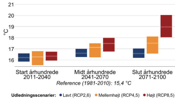
Figur 4 Gennemsnitstemperatur for sommer (jun-aug) og vinter (dec-feb) i fremtidsperioderne 2011-2040, 2041-2070 og 2071-2100 under forskellige udledningsscenarier i Brønderslev Kommune. Den grå linje viser referenceværdien for nutiden (1981-2010).
