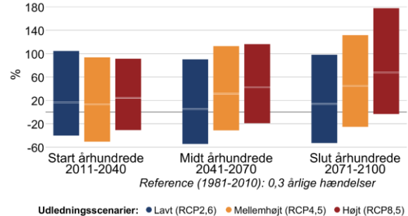
Figur 7 Procentvis ændring af ekstremnedbør hen over året mellem 1981-2010 og fremtidsperioderne 2011-2040, 2041-2070 og 2071-2100 under forskellige udledningsscenarier i Brønderslev Kommune. Til venstre 10-årshændelsen for døgnnedbør, til højre frekvensen af skybrud.
