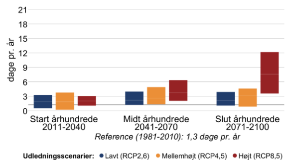
Figur 3 Ændring af gennemsnitstemperatur og antallet af hedebølgedage hen over året mellem 1981-2010 og fremtidsperioderne 2011-2040, 2041-2070 og 2071-2100 under forskellige udledningsscenarier i Brønderslev Kommune.
