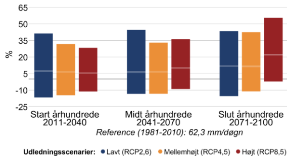
Figur 7 Procentvis ændring af ekstremnedbør hen over året mellem 1981-2010 og fremtidsperioderne 2011-2040, 2041-2070 og 2071-2100 under forskellige udledningsscenarier i Ballerup Kommune. Til venstre 10-årshændelsen for døgnnedbør, til højre frekvensen af skybrud.
