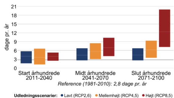
Figur 3 Ændring af gennemsnitstemperatur og antallet af hedebløgedage hen over året mellem 1981-2010 og fremtidsperioderne 2011-2040, 2041-2070 og 2071-2100 under forskellige udledningsscenarier i Ballerup Kommune.
