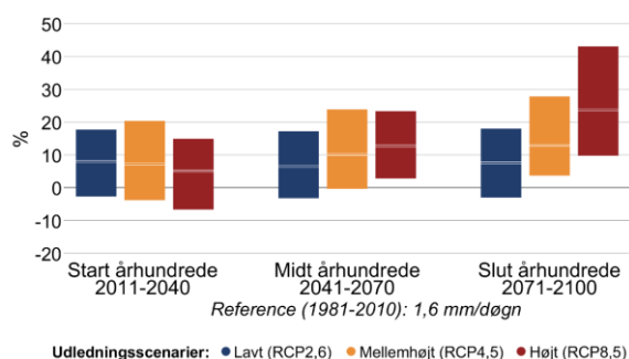
Figur 6 Procentvis ændring af middelnedbør mellem 1981-2010 og fremtidsperioderne 2011-2040, 2041-2070 og 2071-2100 under forskellige udledningsscenarier i Ballerup Kommune. Til venstre sommer (jun-aug), til højre vinter (dec-feb).
