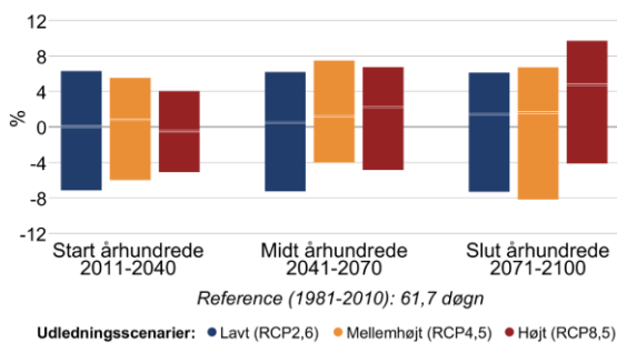
Figur 8 Procentvis ændring af tørre dage om sommeren (jun-aug) mellem 1981-2010 og fremtidsperioderne 2011-2040, 2041-2070 og 2071-2100 under forskellige udledningsscenarier i Ballerup Kommune. Til venstre antallet af tørre dage med mindre end 1 mm nedbør, til højre længden af den længste sammenhængende tørre periode.
