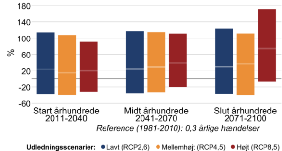
Figur 7 Procentvis ændring af ekstremnedbør hen over året mellem 1981-2010 og fremtidsperioderne 2011-2040, 2041-2070 og 2071-2100 under forskellige udledningsscenarier i Ballerup Kommune. Til venstre 10-årshændelsen for døgnnedbør, til højre frekvensen af skybrud.
