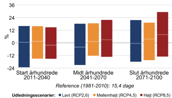
Figur 8 Procentvis ændring af tørre dage om sommeren (jun-aug) mellem 1981-2010 og fremtidsperioderne 2011-2040, 2041-2070 og 2071-2100 under forskellige udledningsscenarier i Ballerup Kommune. Til venstre antallet af tørre dage med mindre end 1 mm nedbør, til højre længden af den længste sammenhængende tørre periode.
