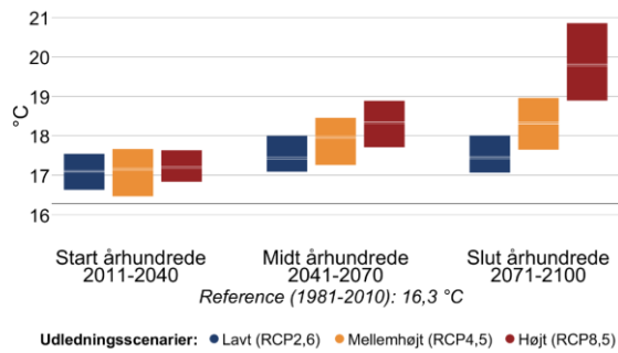
Figur 4 Gennemsnitstemperatur for sommer (jun-aug) og vinter (dec-feb) i fremtidsperioderne 2011-2040, 2041-2070 og 2071-2100 under forskellige udledningsscenarier i Allerød Kommune. Den grå linje viser referenceværdien for nutiden (1981-2010).
