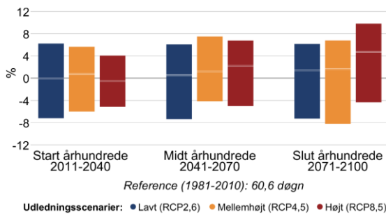
Figur 8 Procentvis ændring af tørre dage om sommeren (jun-aug) mellem 1981-2010 og fremtidsperioderne 2011-2040, 2041-2070 og 2071-2100 under forskellige udledningsscenarier i Allerød Kommune. Til venstre antallet af tørre dage med mindre end 1 mm nedbør, til højre længden af den længste sammenhængende tørre periode.
