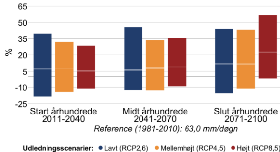
Figur 7 Procentvis ændring af ekstremnedbør hen over året mellem 1981-2010 og fremtidsperioderne 2011-2040, 2041-2070 og 2071-2100 under forskellige udledningsscenarier i Allerød Kommune. Til venstre 10-årshændelsen for døgnet nedbør, til højre frekvensen af skybrud.
