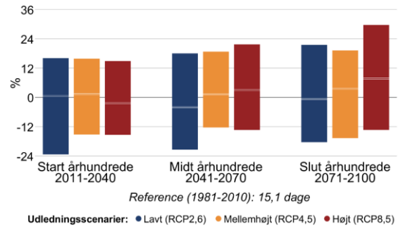
Figur 8 Procentvis ændring af tørre dage om sommeren (jun-aug) mellem 1981-2010 og fremtidsperioderne 2011-2040, 2041-2070 og 2071-2100 under forskellige udledningsscenarier i Allerød Kommune. Til venstre antallet af tørre dage med mindre end 1 mm nedbør, til højre længden af den længste sammenhængende tørre periode.
