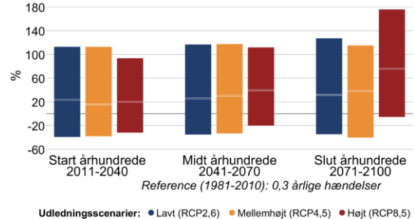
Figur 7 Procentvis ændring af ekstremnedbør hen over året mellem 1981-2010 og fremtidsperioderne 2011-2040, 2041-2070 og 2071-2100 under forskellige udledningsscenarier i Allerød Kommune. Til venstre 10-årshændelsen for døgnet nedbør, til højre frekvensen af skybrud.
