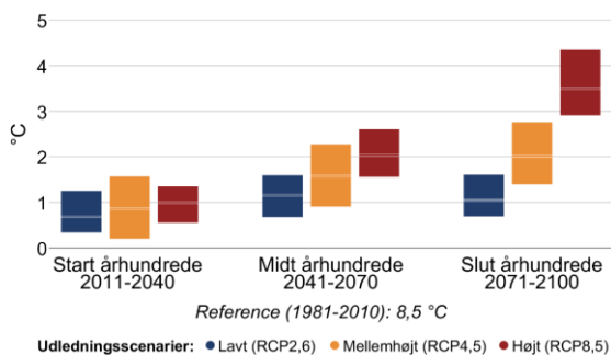
Figur 3 Ændring af gennemsnitstemperatur og antallet af hedebløgedage hen over året mellem 1981-2010 og fremtidsperioderne 2011-2040, 2041-2070 og 2071-2100 under forskellige udledningsscenarier i Allerød Kommune.
