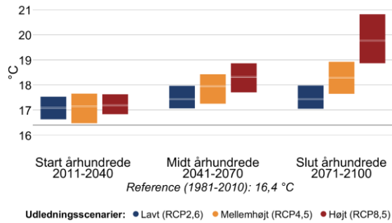
Figur 4 Gennemsnitstemperatur for sommer (jun-aug) og vinter (dec-feb) i fremtidsperioderne 2011-2040, 2041-2070 og 2071-2100 under forskellige udledningsscenarier i Albertslund Kommune. Den grå linje viser referenceværdien for nutiden (1981-2010).
