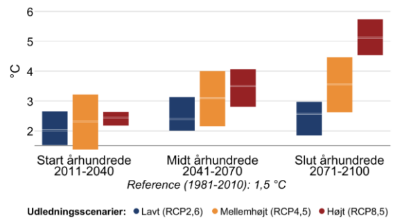
Figur 4 Gennemsnitstemperatur for sommer (jun-aug) og vinter (dec-feb) i fremtidsperioderne 2011-2040, 2041-2070 og 2071-2100 under forskellige udledningsscenarier i Albertslund Kommune. Den grå linje viser referenceværdien for nutiden (1981-2010).
