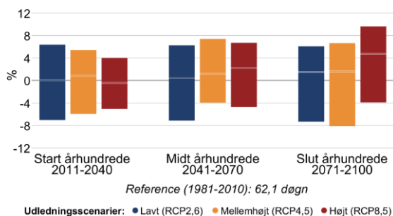
Figur 8 Procentvis ændring af tørre dage om sommeren (jun-aug) mellem 1981-2010 og fremtidsperioderne 2011-2040, 2041-2070 og 2071-2100 under forskellige udledningsscenarier i Albertslund Kommune. Til venstre antallet af tørre dage med mindre end 1 mm nedbør, til højre længden af den længste sammenhængende tørre periode.
