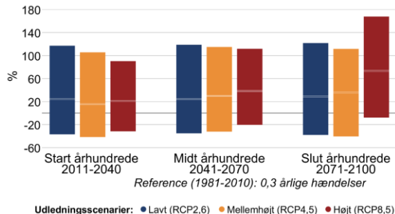
Figur 7 Procentvis ændring af ekstremnedbør hen over året mellem 1981-2010 og fremtidsperioderne 2011-2040, 2041-2070 og 2071-2100 under forskellige udledningsscenarier i Albertslund Kommune. Til venstre 10-årshændelsen for døgnnedbør, til højre frekvensen af skybrud.
