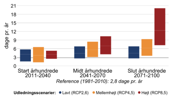
Figur 3 Ændring af gennemsnitstemperatur og antallet af hedebløgedage hen over året mellem 1981-2010 og fremtidsperioderne 2011-2040, 2041-2070 og 2071-2100 under forskellige udledningsscenarier i Albertslund Kommune.
