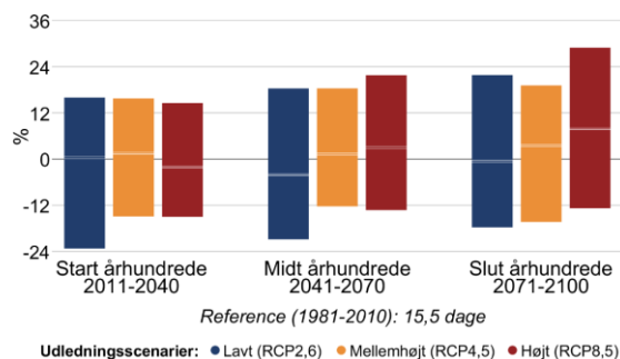
Figur 8 Procentvis ændring af tørre dage om sommeren (jun-aug) mellem 1981-2010 og fremtidsperioderne 2011-2040, 2041-2070 og 2071-2100 under forskellige udledningsscenarier i Albertslund Kommune. Til venstre antallet af tørre dage med mindre end 1 mm nedbør, til højre længden af den længste sammenhængende tørre periode.
