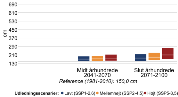
Figur 11 Højden af 20- (venstre) og 100-års (højre) stormflodhændelser for Århus Bugt i fremtidsperioderne 2041-2070 og 2071-2100 under forskellige udledningsscenarier. Den grå linje viser referenceværdien for nutiden (1981-2010).
