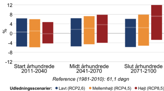
Figur 8 Procentvis ændring af tørre dage om sommeren (jun-aug) mellem 1981-2010 og fremtidsperioderne 2011-2040, 2041-2070 og 2071-2100 under forskellige udledningsscenarier i Aarhus Kommune. Til venstre antallet af tørre dage med mindre end 1 mm nedbør, til højre længden af den længste sammenhængende tørre periode.
