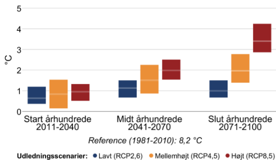
Figur 3 Ændring af gennemsnitstemperatur og antallet af hedebølgedage hen over året mellem 1981-2010 og fremtidsperioderne 2011-2040, 2041-2070 og 2071-2100 under forskellige udledningsscenarier i Aarhus Kommune.
