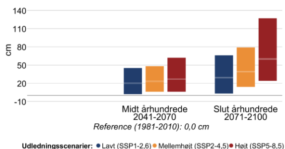
Figur 10 Ændring i middelvandstand (venstre) og hyppigheden af stormflod for Århus Bugt i fremtidsperioderne 2041-2070 og 2071-2100 under forskellige udledningsscenerier. Den grå linje viser referenceværdien for nutiden (1981-2010). En stormflod defineres her som en forhøjet vandstand, der statistisk set kun forekommer én gang hvert 20. år i perioden 1981-2010. Bemærk også at denne indikator kappes ved 60 stormfloder per 20 år.
