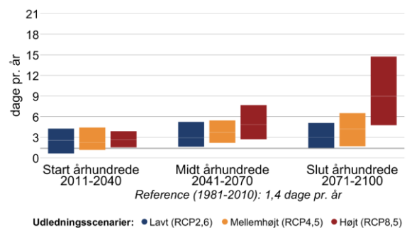
Figur 3 Ændring af gennemsnitstemperatur og antallet af hedebølgedage hen over året mellem 1981-2010 og fremtidsperioderne 2011-2040, 2041-2070 og 2071-2100 under forskellige udledningsscenarier i Aarhus Kommune.
