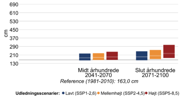
Figur 11 Højden af 20- (venstre) og 100-års (højre) stormflodhændelser for Århus Bugt i fremtidsperioderne 2041-2070 og 2071-2100 under forskellige udledningsscenarier. Den grå linje viser referenceværdien for nutiden (1981-2010).
