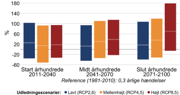
Figur 7 Procentvis ændring af ekstremnedbør hen over året mellem 1981-2010 og fremtidsperioderne 2011-2040, 2041-2070 og 2071-2100 under forskellige udledningsscenarier i Aarhus Kommune. Til venstre 10-årshændelsen for døgnet, til højre frekvensen af skybrud.
