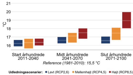
Figur 4 Gennemsnitstemperatur for sommer (jun-aug) og vinter (dec-feb) i fremtidsperioderne 2011-2040, 2041-2070 og 2071-2100 under forskellige udledningsscenarier i Aarhus Kommune. Den grå linje viser referenceværdien for nutiden (1981-2010).
