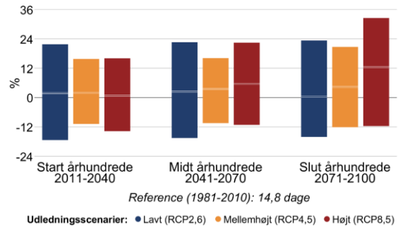
Figur 8 Procentvis ændring af tørre dage om sommeren (jun-aug) mellem 1981-2010 og fremtidsperioderne 2011-2040, 2041-2070 og 2071-2100 under forskellige udledningsscenarier i Aarhus Kommune. Til venstre antallet af tørre dage med mindre end 1 mm nedbør, til højre længden af den længste sammenhængende tørre periode.
