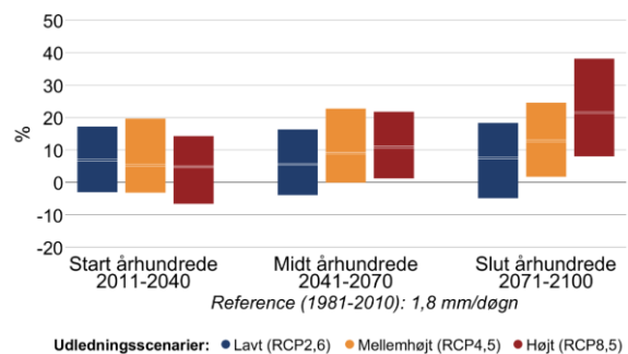
Figur 6 Procentvis ændring af middelnedbør mellem 1981-2010 og fremtidsperioderne 2011-2040, 2041-2070 og 2071-2100 under forskellige udledningsscenarier i Aarhus Kommune. Til venstre sommer (jun-aug), til højre vinter (dec-feb).
