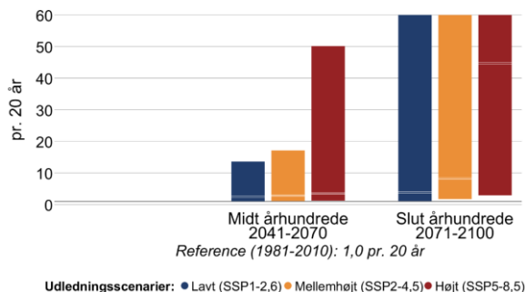
Figur 10 Ændring i middelvandstand (venstre) og hyppigheden af stormflod for Århus Bugt i fremtidsperioderne 2041-2070 og 2071-2100 under forskellige udledningsscenerier. Den grå linje viser referenceværdien for nutiden (1981-2010). En stormflod defineres her som en forhøjet vandstand, der statistisk set kun forekommer én gang hvert 20. år i perioden 1981-2010. Bemærk også at denne indikator kappes ved 60 stormfloder per 20 år.
