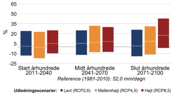
Figur 7 Procentvis ændring af ekstremnedbør hen over året mellem 1981-2010 og fremtidsperioderne 2011-2040, 2041-2070 og 2071-2100 under forskellige udledningsscenarier i Aarhus Kommune. Til venstre 10-årshændelsen for døgnet, til højre frekvensen af skybrud.
