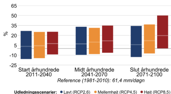
Figur 7 Procentvis ændring af ekstremnedbør hen over året mellem 1981-2010 og fremtidsperioderne 2011-2040, 2041-2070 og 2071-2100 under forskellige udledningsscenarier i Aalborg Kommune. Til venstre 10-årshændelsen for døgnnedbør, til højre frekvensen af skybrud.
