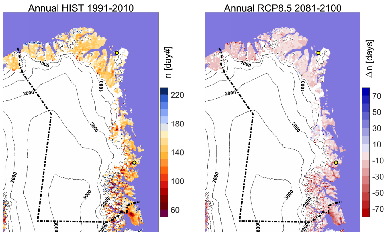
Figur 27. Snedækkets sæsonophør (kalenderdag) i Nationalparken i referenceperioden 1991-2010 til venstre. Til højre ses ændringen i antal dage i 2081-2100 i forhold til 1991-2010 beregnet for RCP8.5-scenariet.
