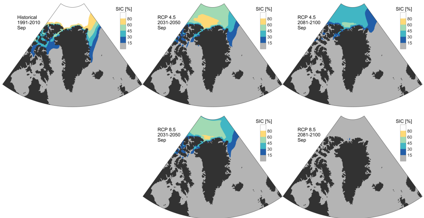
Figur 13 Gennemsnitlig september havisudbredelse i % baseret på klimamodeller i CMIP5. Der er lavet en middelværdi over i alt 29 modeller. Øverst til venstre: repræsenterende periode 1991-2010; øverst midt for: RCP 4.5 2031-2050; øverst til højre: RCP 4.5 2081-2100; nederst til venstre RCP8.5 2031-2050; nederst til højre: RCP8.5 2081-2100. Kilde: CMIP5 og DMI.
