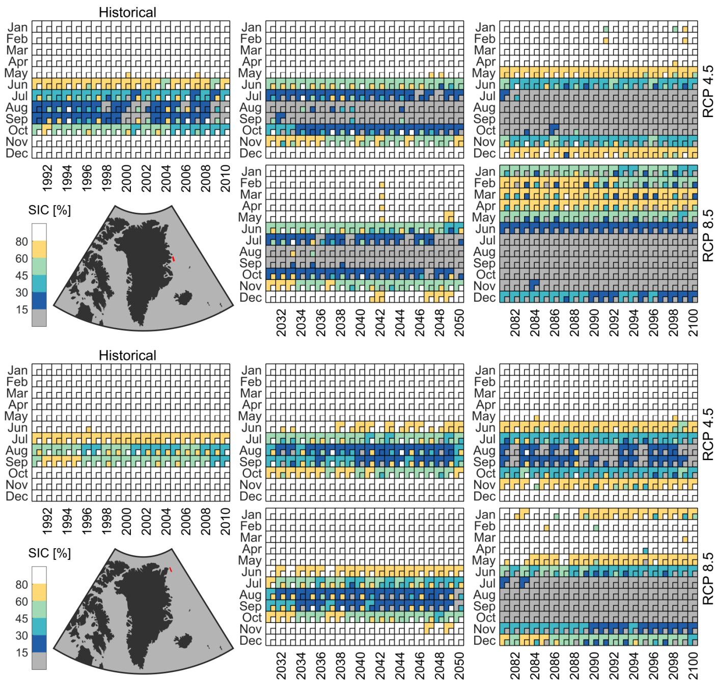
Figur 14. Forekomsten af havis for 73°N, 34°W (øverst) og for 80°N, 35°W (nederst) fordelt på måneds basis. Stor firkant repræsenterer information baseret på alle modeller, lille firkant (indsat) er for DMI's model. Kilde CMIP5 og DMI.
