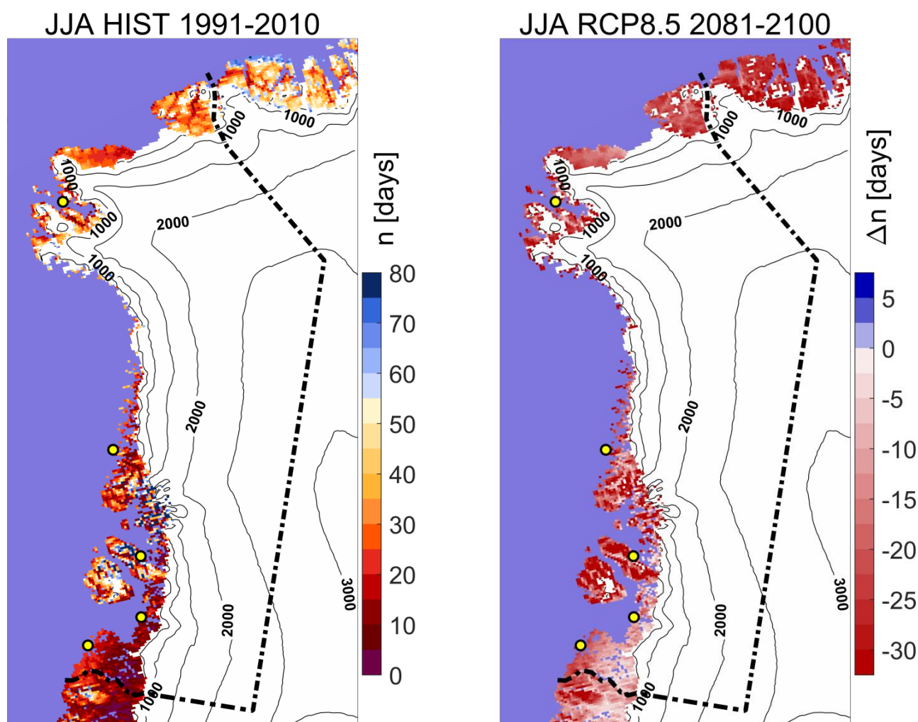
Figur 15. Forekomst af sommerfrost. Antallet af døgn i løbet juni-juli-august med minimum temperatur under 0 °C 1991-2010 til venstre. Til højre er vist ændringen i antal døgn i 2081-2100 i forhold til 1991-2010 beregnet for RCP8.5-scenariet.
