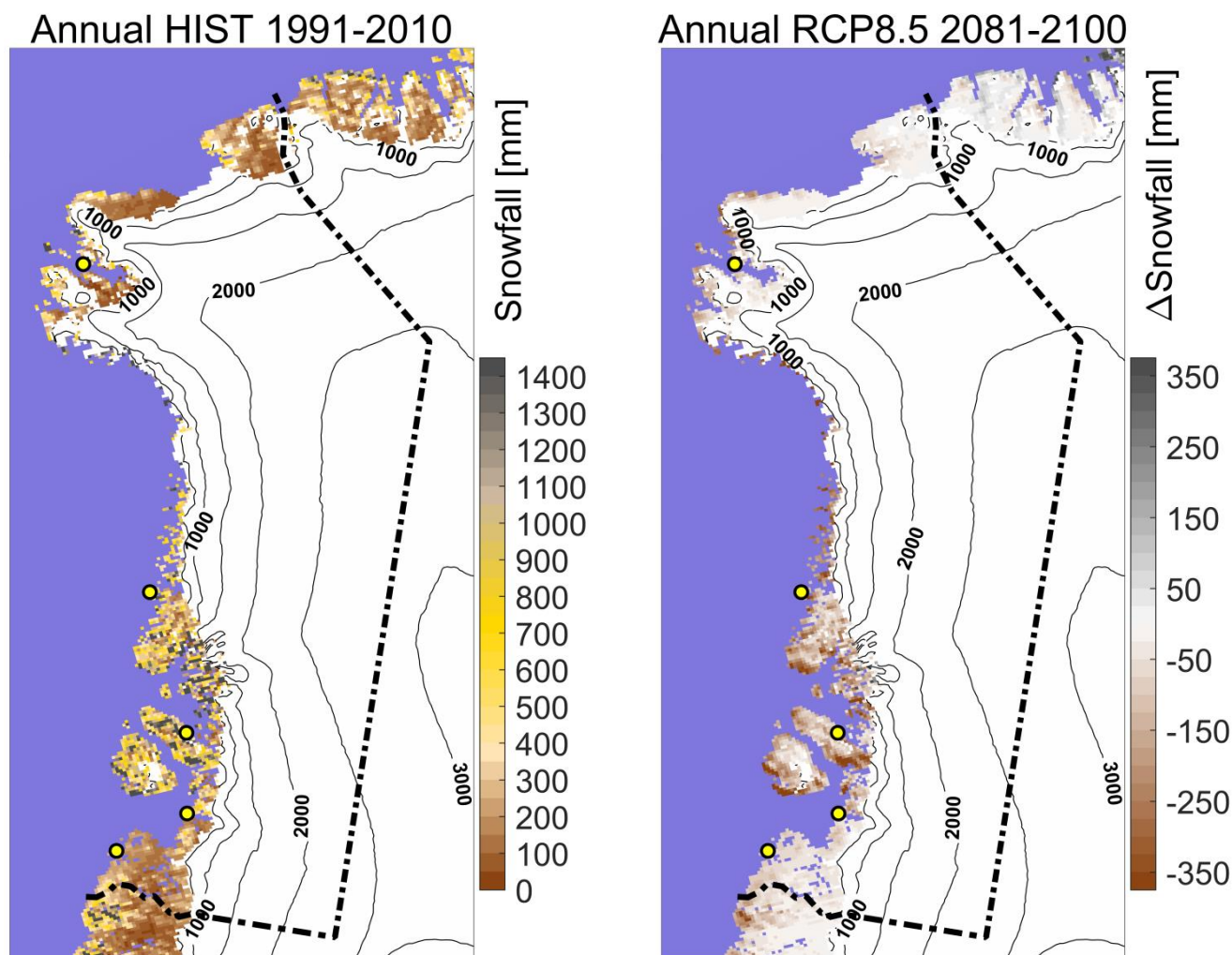
Figur 18. Årligt snefald. Mængden af sne der falder i løbet af et år i referenceperioden 1991-2010 til venstre angivet i mm per år. Til højre er vist ændringen i årligt snefald i 2081-2100 i forhold til 1991-2010 beregnet for RCP8.5-scenariet.
