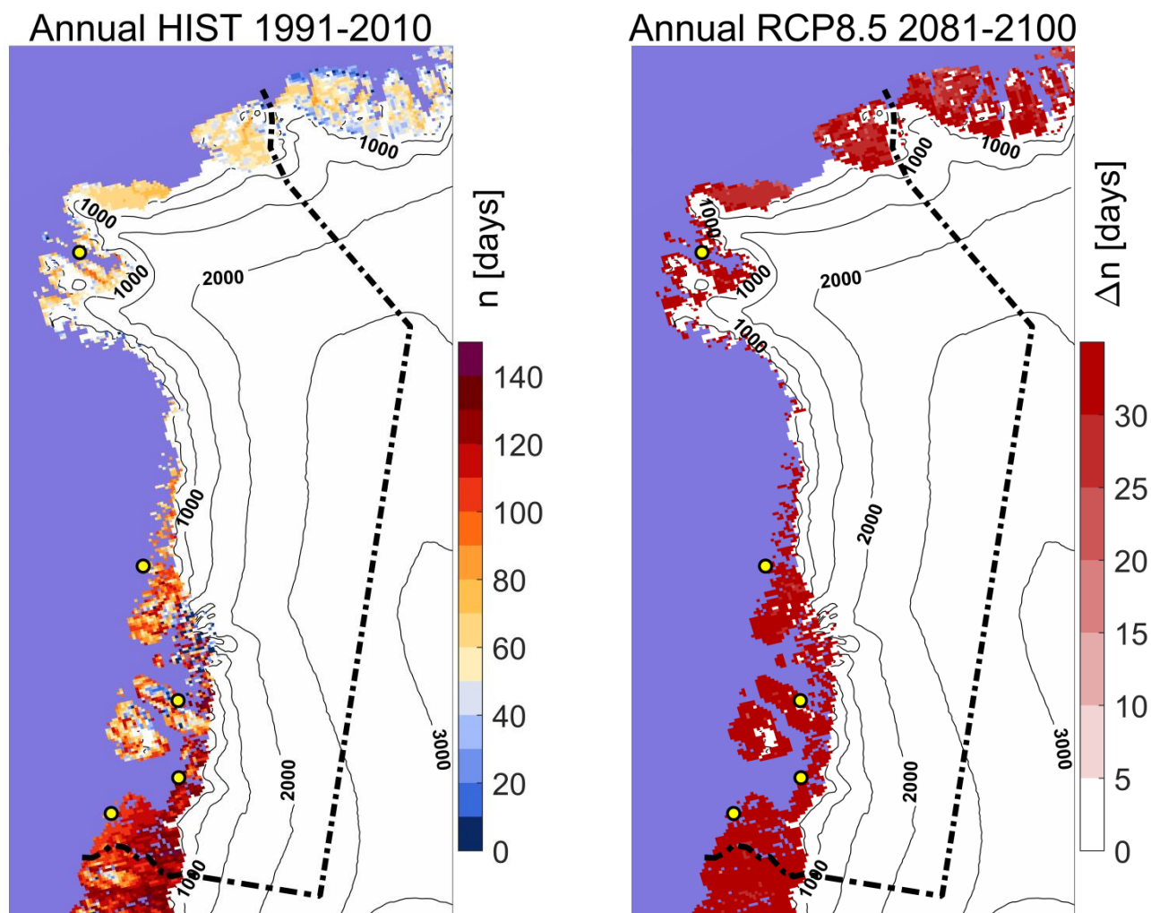
Figur 23. Vækstsæsonens længde i Qaasuitsup Kommune i referenceperioden 1991-2010 til venstre. Til højre ses ændringen i vækstsæsonens længde (antal dage) i 2081-2100 i forhold til 1991-2010 beregnet for RCP8.5-scenariet.
