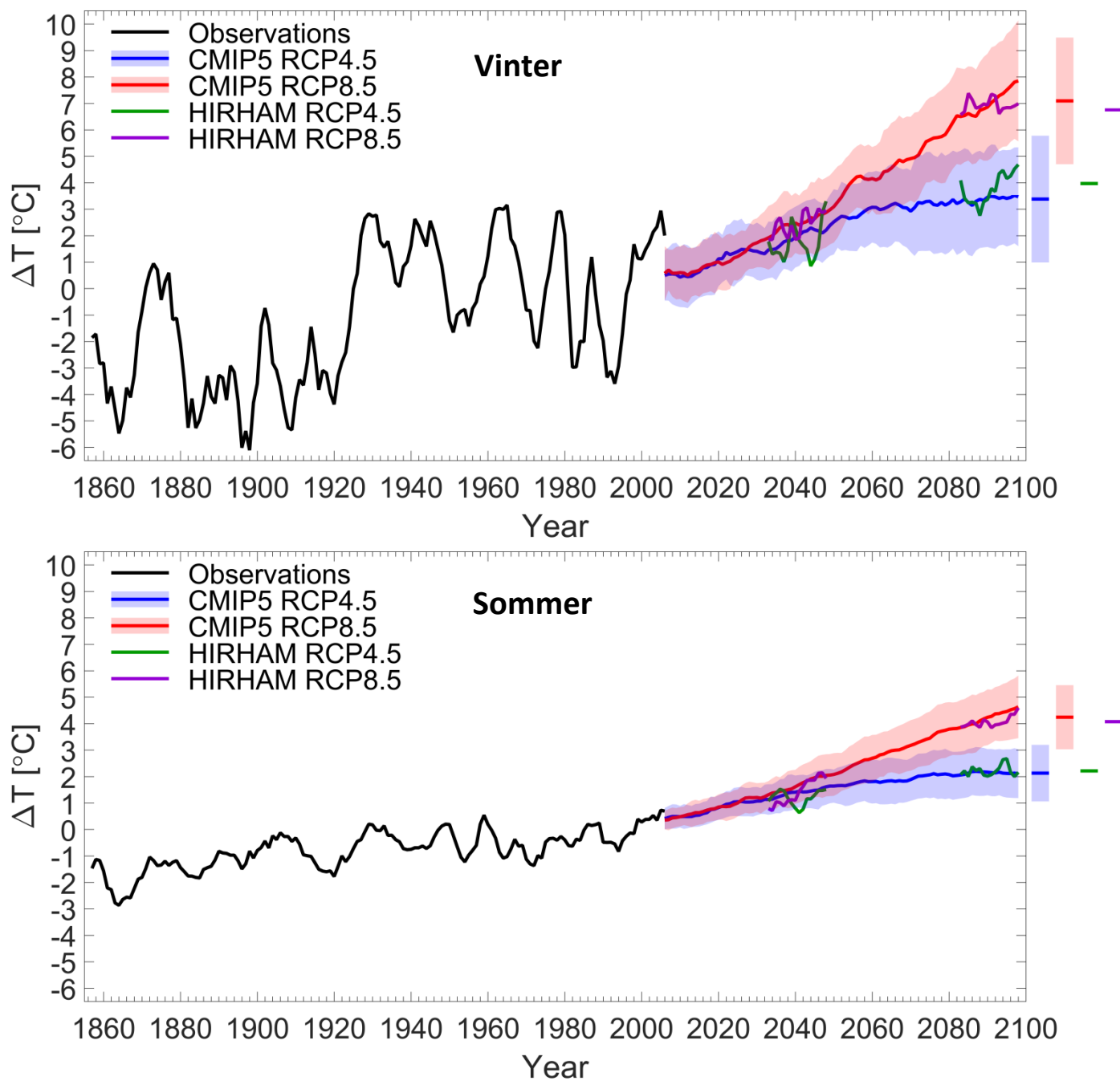
Figur 4. Temperaturændringer i Qaasuitsup Kommune som i figur 3 men for vinter (øverst) og sommer (nederst).
