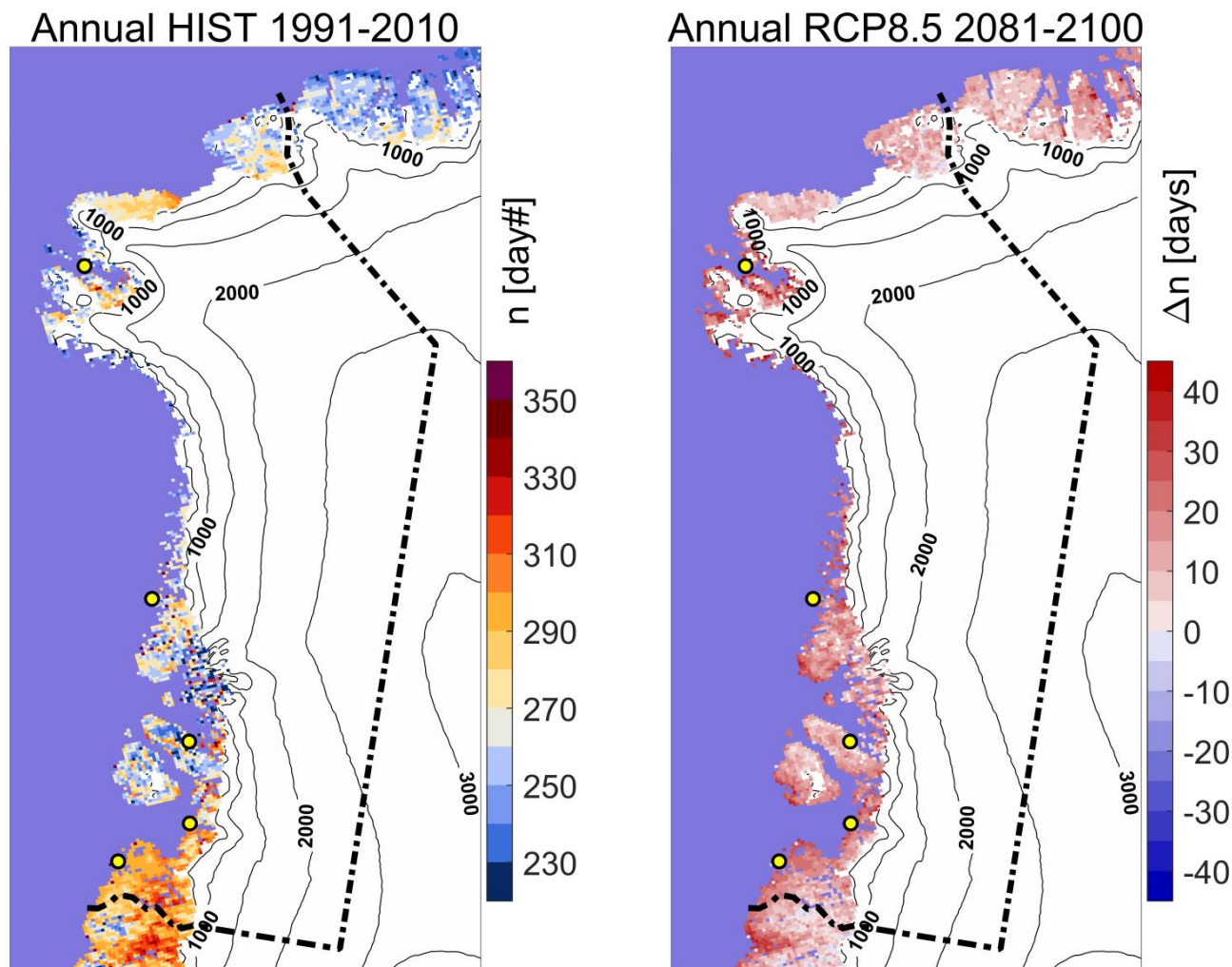
Figur 26. Snedækkets sæsonstart (kalenderdag) i Qaasuitsup Kommune i referenceperioden 1991-2010 til venstre. Til højre ses forskydningen i antal dage i 2081-2100 i forhold til 1991-2010 beregnet for RCP8.5-scenariet.
