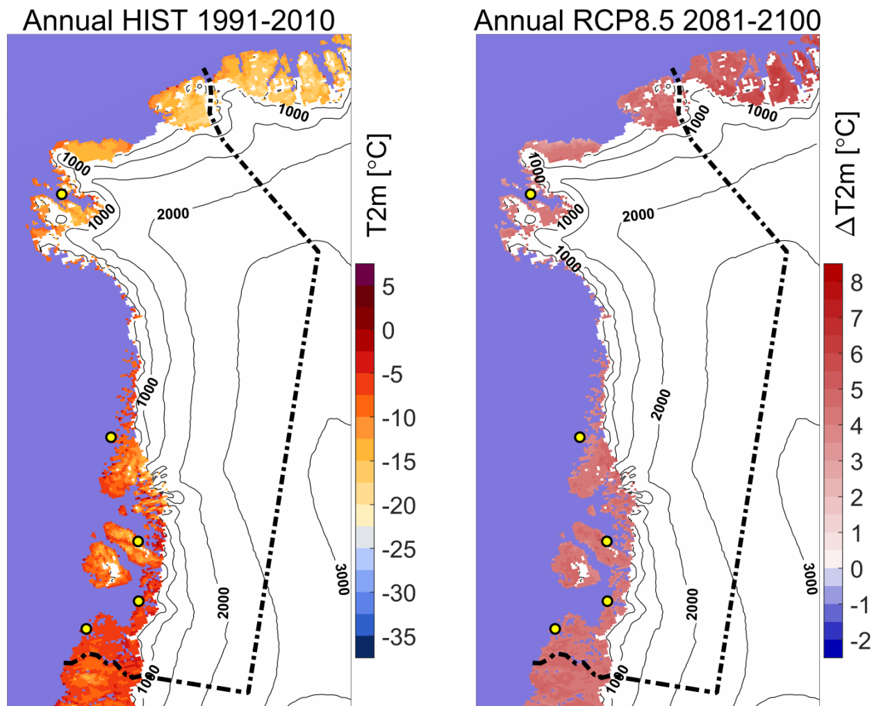
Figur 5. Modelleret årlig middeltemperatur for Qaasuitsup Kommune. Middeltemperaturen i referenceperioden 1991-2010 til venstre. Til højre er vist ændringen i middeltemperatur i 2081-2100 i forhold til 1991-2010 beregnet for RCP8.5-scenariet.
