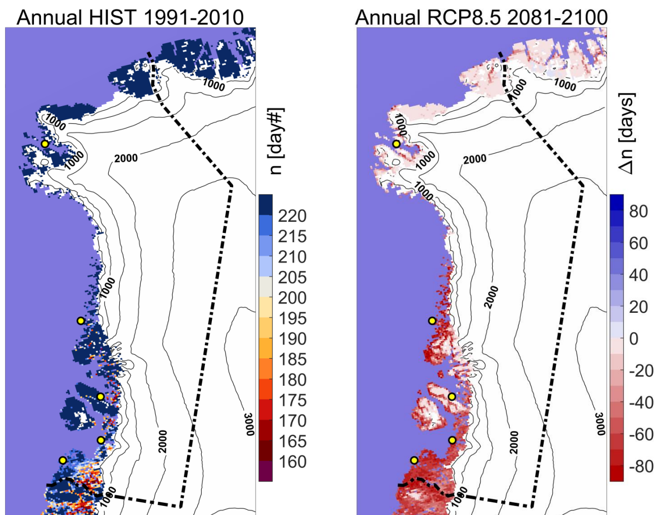
Figur 22. Årets sidste dag med forårsfrost (kalenderdag) i referenceperioden 1991-2010 til venstre. Til højre ses ændringen i sidste forårsfrostdag (antal dage) i 2081-2100 i forhold til 1991-2010 beregnet for RCP8.5-scenariet.
