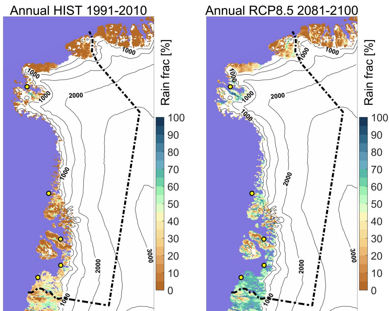
Figur 19. Årlig andel af nedbøren, der falder som regn i det nuværende klima 1991-2010 til venstre angivet i procent. Til højre ses den procentvise andel for 2081-2100 beregnet for RCP8.5-scenariet.
