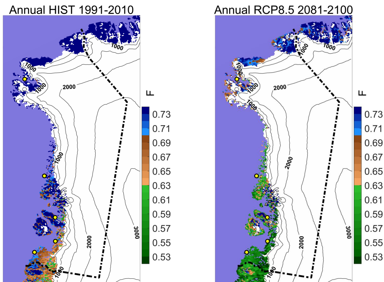
Figur 24. Permafrostindeks i Qaasuitsup Kommune i referenceperioden 1991-2010 til venstre. Til højre ses Permafrostindekset i 2081-2100 beregnet for RCP8.5-scenariet.
