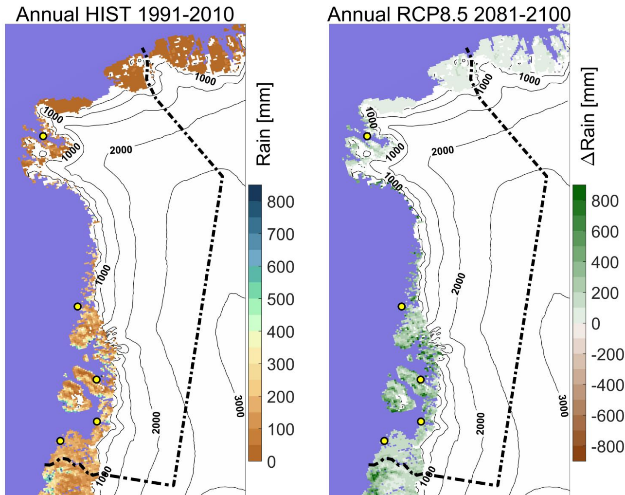
Figur 17. Årlig regnmængde opsummeret. Mængden af regn i løbet af et år i referenceperioden 1991-2010 til venstre i mm. Til højre er vist ændringen i årlig regnmængde i 2081-2100 i forhold til 1991-2010 beregnet for RCP8.5-scenariet.
