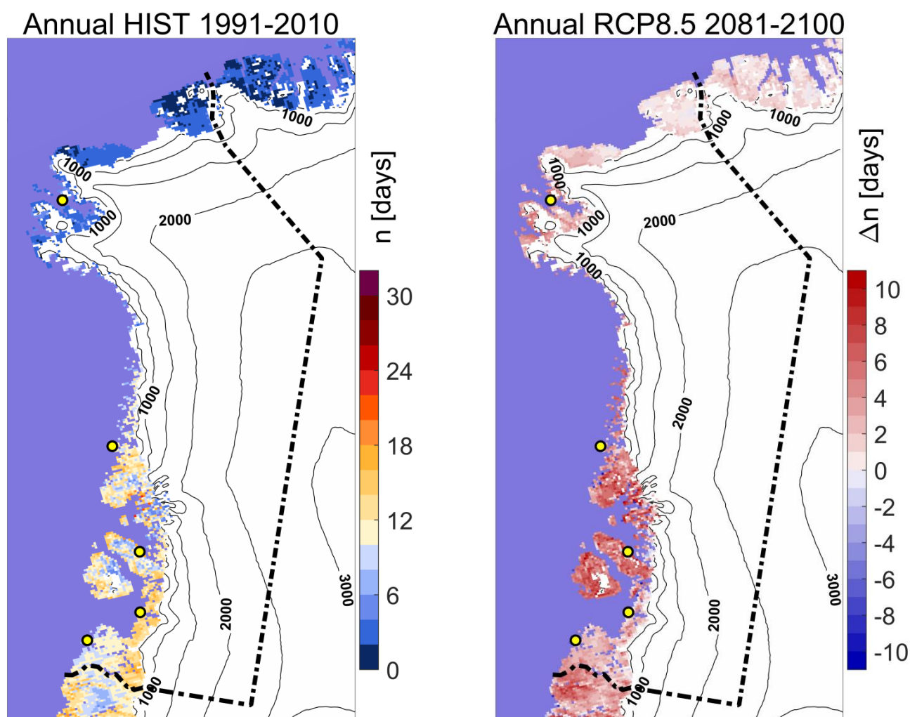
Figur 25. Antallet af vintersmeltedage i Qaasuitsup Kommune i referenceperioden 1991-2010 til venstre. Til højre ses ændringen i antallet i 2081-2100 i forhold til 1991-2010 beregnet for RCP8.5-scenariet.
