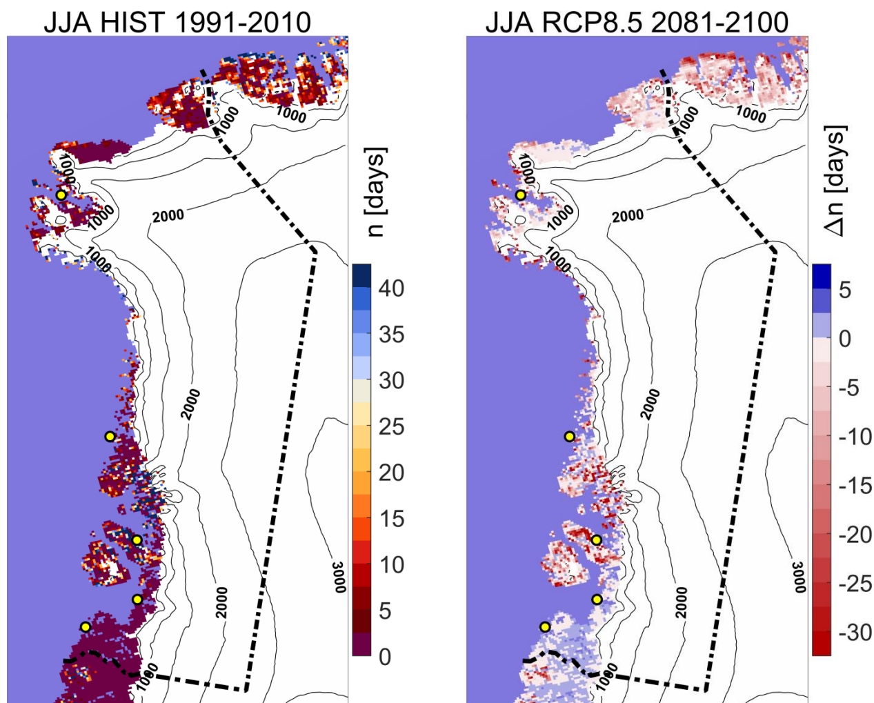
Figur 20. Sommersnedækkets længde i det nuværende klima 1991-2010 til venstre angivet i dage. Til højre er vist ændringen i antal dage med sommersnedække i 2081-2100 i forhold til 1991-2010 beregnet for RCP8.5-scenariet. En dag med snedække er defineret med en snedække af 2 cm eller mere.
