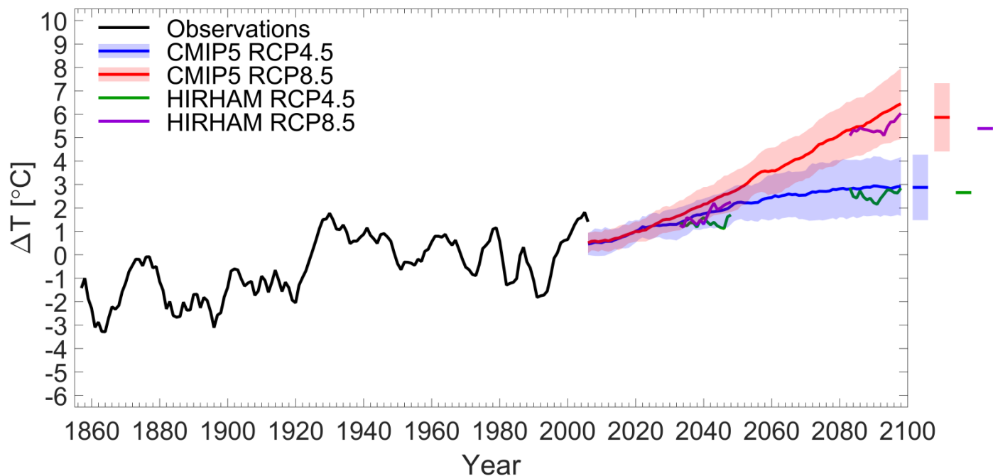
Figur 3. Årlig udvikling i middeltemperatur for Qaasuitsup Kommune i forhold til referenceperioden 1986-2005. Sort kurve: Observationer fra 1855 til 2005 i Ilulissat. Blå og rød kurve: Modellsimulering for perioden 2006-2100 for henholdsvis RCP4.5-scenariet og RCP8.5-scenariet. De skraverede lysere farvede områder angiver vurderede nøjagtigheder på temperaturstigningerne. For de samme scenarier er med hhv. grøn og violet angivet resultater baseret på DMI's detaljerede klimamodel for Grønland, som kun har regnet for forskellige tidsudsnit. For alle scenariekurverne er der anvendt et glidende 5-års-middel. Til højre ses middeltemperaturstigningerne for de sidste 20 år (2081 – 2100) af simuleringerne. Kilde: Observationsdata: DMI; Modellsimuleringer: CMIP5 og DMI.
