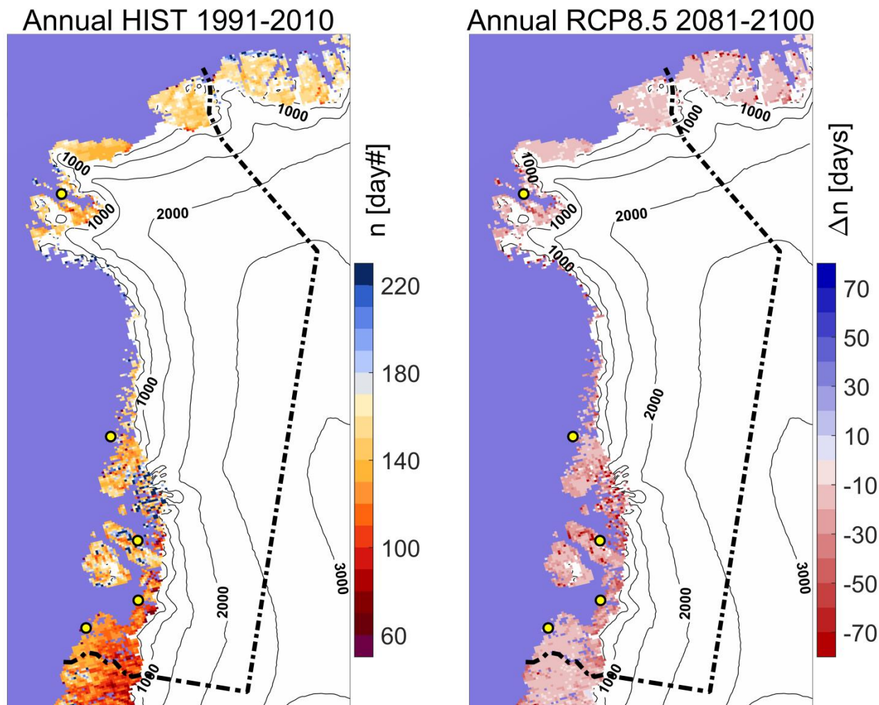
Figur 27. Snedækkets sæsonophør (kalenderdag) i Qaasuitsup Kommune i referenceperioden 1991-2010 til venstre. Til højre ses ændringen i antal dage i 2081-2100 i forhold til 1991-2010 beregnet for RCP8.5-scenariet.
