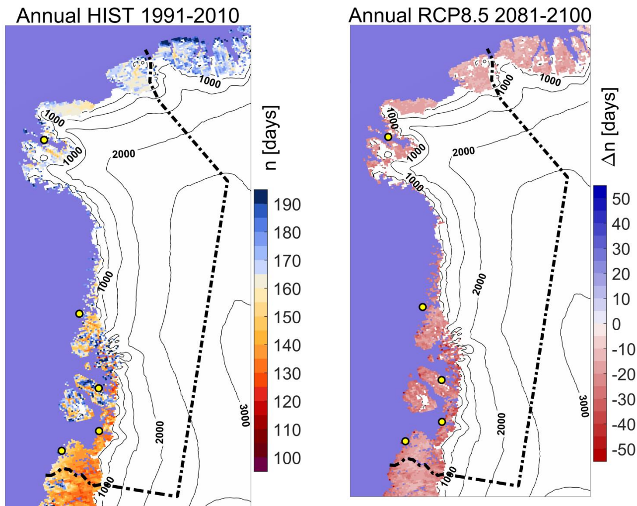
Figur 21. Vækstsæsonens begyndelsestidspunkt i referenceperioden 1991-2010 som kalenderdag til venstre. Til højre ses ændringen i vækstsæsonens begyndelsestidspunkt (antal dage) i 2081-2100 i forhold til 1991-2010 beregnet for RCP8.5-scenariet.
