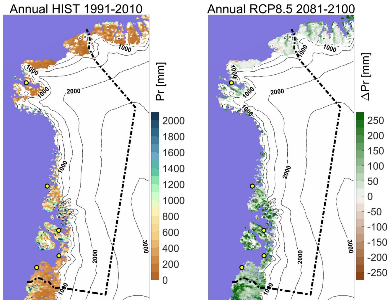
Figur 9. Nedbørssum. Den modelbaserede samlede årlige nedbørssum i referenceperioden 1991-2010 til venstre. Til højre er vist ændringen i årlig nedbørssum i 2081-2100 i forhold til 1991-2010 beregnet for RCP8.5-scenariet.
