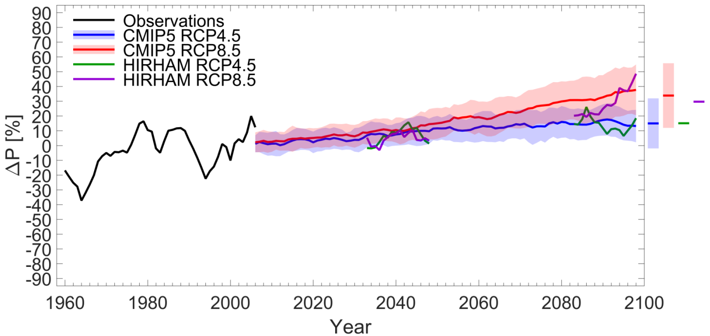
Figur 7. Procentvise årlige nedbørsændringer i Qaasuitsup Kommune i forhold til referenceperioden 1986-2005. Sort kurve: Observationer fra 1958 til 2005 i Aasiaat. Blå og rød kurve: Modellsimulering for perioden 2006-2100 for henholdsvis RCP4.5-scenariet og RCP8.5-scenariet. De skraverede lysere farvede områder omkring angiver vurderede nøjagtigheder på nedbørændringerne. For de samme scenarier er med hhv. grøn og violet angivet resultater baseret på DMI's detaljerede klimamodel for Grønland, som kun har beregnet forskellige tidsudsnit. For alle scenarie-kurverne er der anvendt et glidende 5-års-middel. Til højre ses middelændringerne for de sidste 20 år (2081 – 2100) af simuleringerne. Kilde: Observationsdata: DMI; Modellsimuleringer: CMIP5 og DMI.
