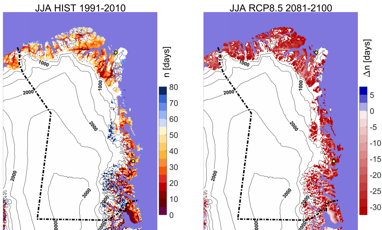
Figur 15. Forekomst af sommerfrost. Antallet af døgne i løbet juni-juli-august med minimum temperatur under 0^{\circ}\text{C} 1991-2010 til venstre. Til højre er vist ændringen i antal døgne i 2081-2100 i forhold til 1991-2010 beregnet for RCP8.5-scenariet.
