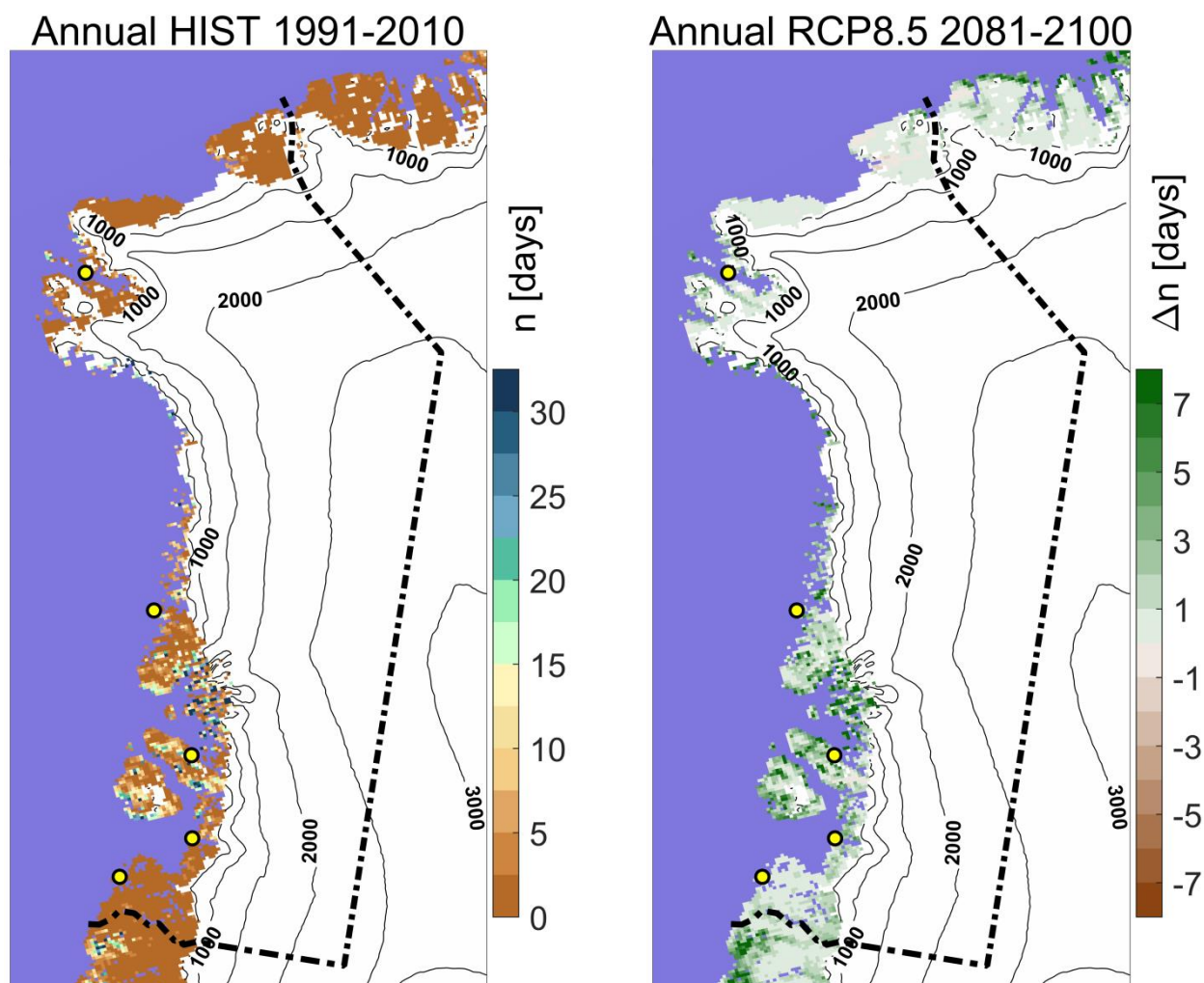
Figur 16. Ekstremnedbør. Antallet af døgnet i løbet af et år med mere end 25mm nedbør i referenceperioden 1991-2010 til venstre. Til højre er vist ændringen i antal døgnet med mere end 25 mm nedbør i 2081-2100 i forhold til 1991-2010 beregnet for RCP8.5-scenariet.
