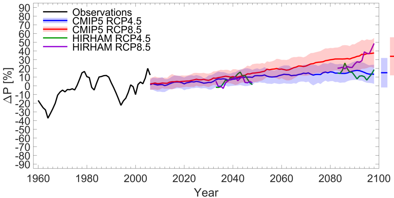
Figur 7. Procentvise årlige nedbørsændringer i Qaasuitsup Kommune i forhold til referenceperioden 1986-2005. Sort kurve: Observationer fra 1958 til 2005 i Aasiaat. Blå og rød kurve: Modellsimulering for perioden 2006-2100 for henholdsvis RCP4.5-scenariet og RCP8.5-scenariet. De skraverede lysere farvede områder omkring angiver vurderede nøjagtigheder på nedbørændringerne. For de samme scenarier er med hhv. grøn og violet angivet resultater baseret på DMI's detaljerede klimamodel for Grønland, som kun har beregnet forskellige tidsudsnit. For alle scenarie-kurverne er der anvendt et glidende 5-års-middel. Til højre ses middelændringerne for de sidste 20 år (2081 – 2100) af simuleringerne. Kilde: Observationsdata: DMI; Modellsimuleringer: CMIP5 og DMI.
