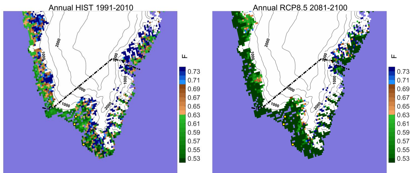
Figur 24. Permafrostindeks i Sydgrønland i referenceperioden 1991-2010 til venstre. Til højre ses Permafrostindekset i 2081-2100 beregnet for RCP8.5-scenariet.
