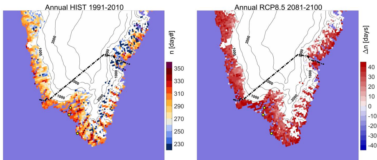
Figur 26. Snedækkets sæsonstart (kalenderdag) i Sydgrønland i referenceperioden 1991-2010 til venstre. Til højre ses forskydningen i antal dage i 2081-2100 i forhold til 1991-2010 beregnet for RCP8.5-scenariet.
