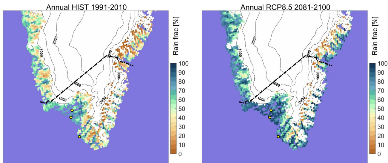
Figur 20. Årlig andel af nedbøren, der falder som regn i det nuværende klima 1991-2010 til venstre angivet i procent. Til højre ses den procentvise andel for 2081-2100 beregnet for RCP8.5-scenariet.
