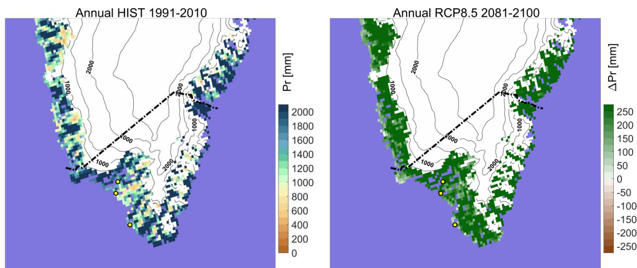
Figur 9. Nedbørssum. Den modelbaserede samlede årlige nedbørssum i referenceperioden 1991-2010 til venstre. Til højre er vist ændringen i årlig nedbørssum i 2081-2100 i forhold til 1991-2010 beregnet for RCP8.5-scenariet.
