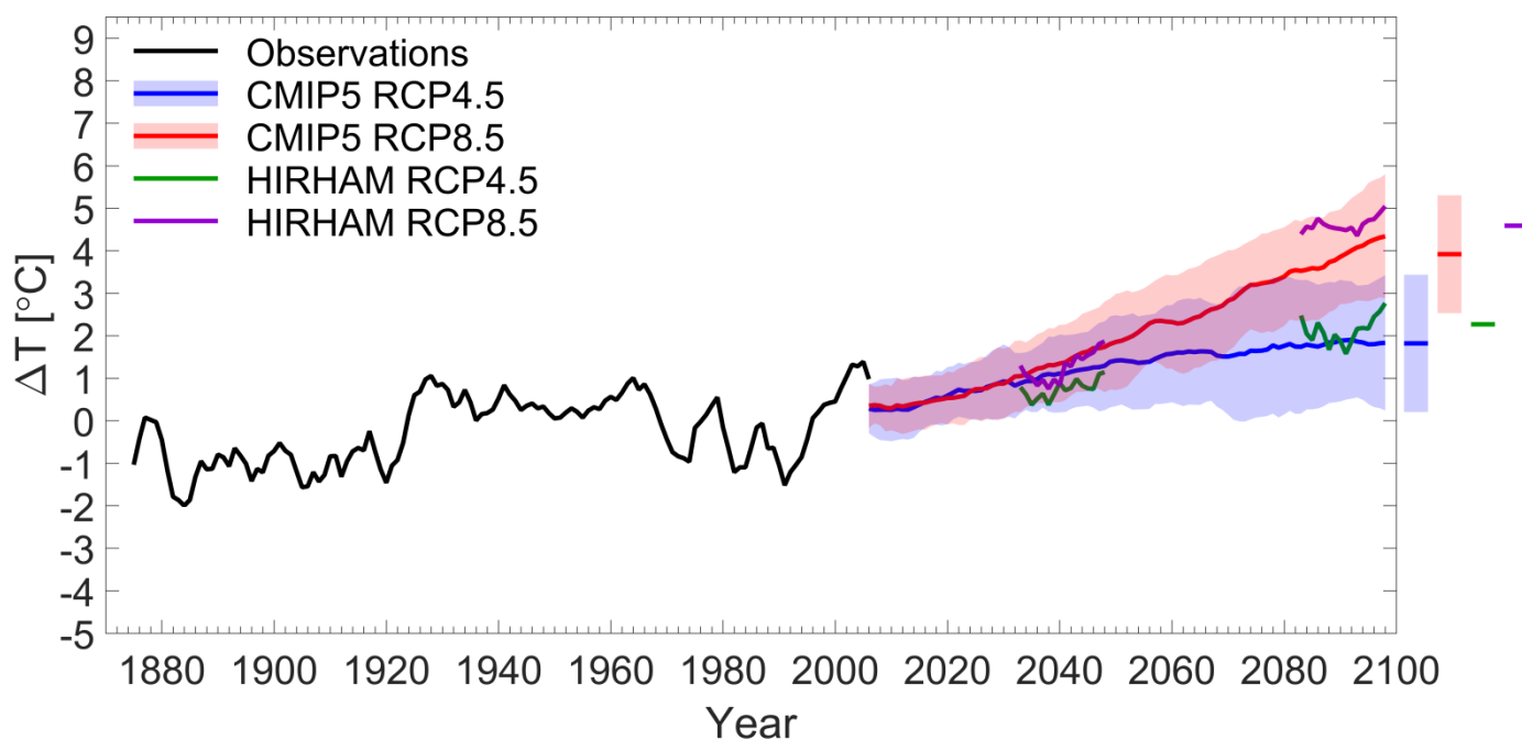
Figur 3. Årlig udvikling i middeltemperatur for Sydgrønland i forhold til referenceperioden 1986-2005. Sort kurve: Observationer fra 1873 til 2005 i Qaqortoq. Blå og rød kurve: Modellsimulering for perioden 2006-2100 for henholdsvis RCP4.5-scenariet og RCP8.5-scenariet. De skraverede lysere farvede områder angiver vurderede nøjagtigheder på temperaturstigningerne. For de samme scenarier er med hhv. grøn og violet angivet resultater baseret på DMI's detaljerede klimamodel for Grønland, som kun har regnet for forskellige tidsudsnit. For alle scenarie-kurverne er der anvendt et glidende 5-års-middel. Til højre ses middeltemperaturstigningerne for de sidste 20 år (2081 – 2100) af simuleringerne. Kilde: Observationsdata: DMI; Modellsimuleringer: CMIP5 og DMI.
