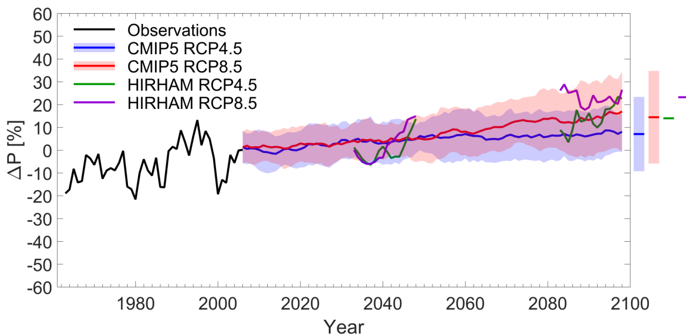
Figur 7. Procentvise årlige nedbørsændringer i Sydgrønland i forhold til referenceperioden 1986-2005. Sort kurve: Observationer fra 1961 til 2005 i Narsarsuaq. Blå og rød kurve: Modelsimulering for perioden 2006-2100 for henholdsvis RCP4.5-scenariet og RCP8.5-scenariet. De skraverede lysere farvede områder omkring angiver vurderede nøjagtigheder på nedbørændringerne. For de samme scenarier er med hhv. grøn og violet angivet resultater baseret på DMI's detaljerede klimamodel for Grønland, som kun har beregnet forskellige tidsudsnit. For alle scenarie-kurverne er der anvendt et glidende 5-års-middel. Til højre ses middelændringerne for de sidste 20 år (2081 – 2100) af simuleringerne. Kilde: Observationsdata: DMI; Modelsimuleringer: CMIP5 og DMI.
