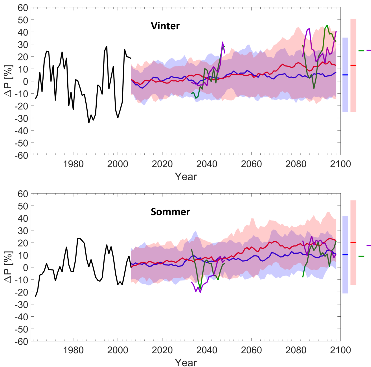
Figur 8. Procentvise nedbørsændringer i Sydgrønland som i figur 7 men for vinter (øverst) og sommer (nederst). Farvekoderne for de enkelte kurver kan ses på figur 7.
