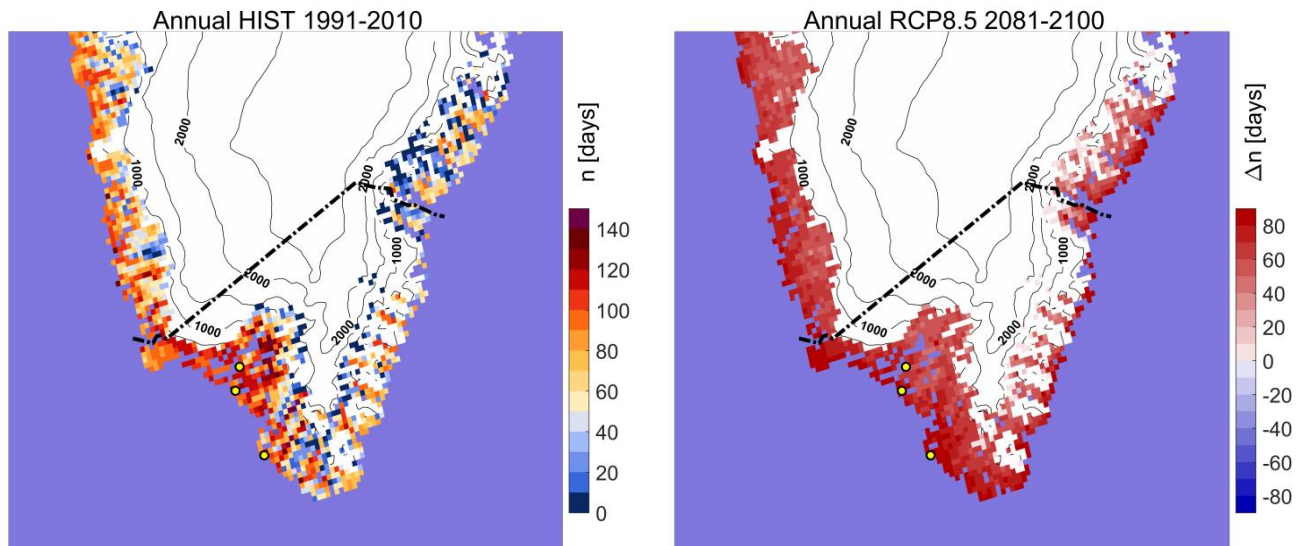
Figur 23. Vækstsæsonens længde i Sydgrønland i referenceperioden 1991-2010 til venstre. Til højre ses ændringen i vækstsæsonens længde (antal dage) i 2081-2100 i forhold til 1991-2010 beregnet for RCP8.5-scenariet.
