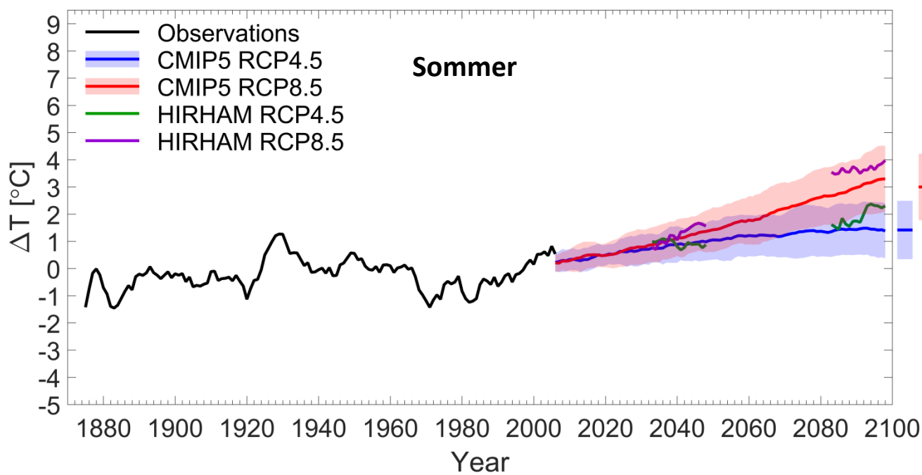
Figur 4. Temperaturændringer i Sydgrønland som i figur 3 men for vinter (øverst) og sommer (nederst).
