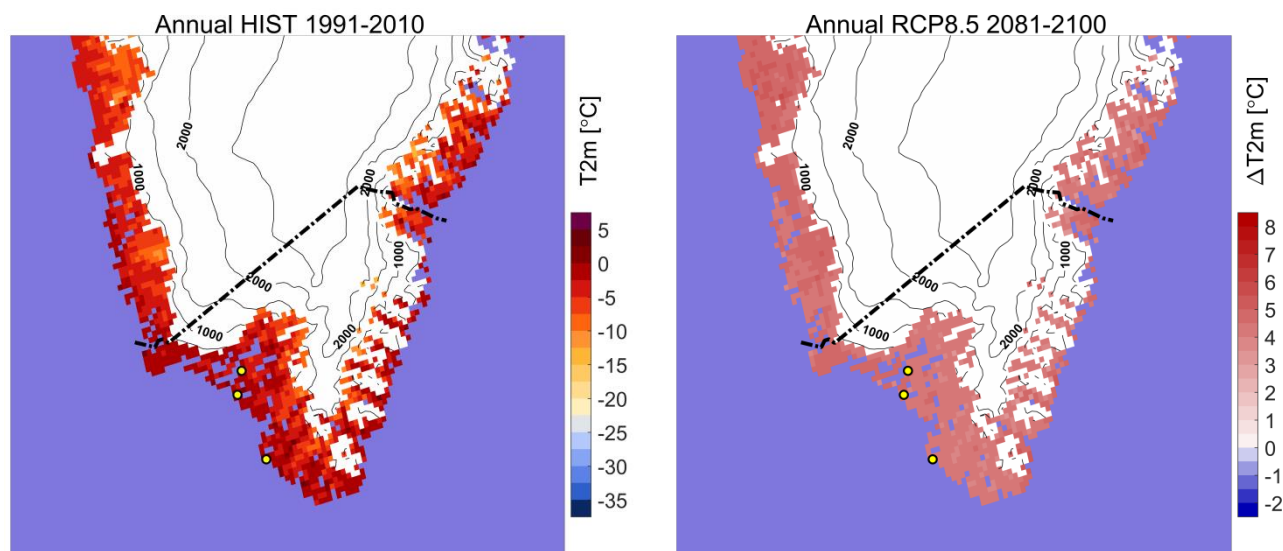
Figur 5. Modelleret årlig middeltemperatur for Sydgrønland. Middeltemperaturen i referenceperioden 1991-2010 til venstre. Til højre er vist ændringen i middeltemperatur i 2081-2100 i forhold til 1991-2010 beregnet for RCP8.5-scenariet.
