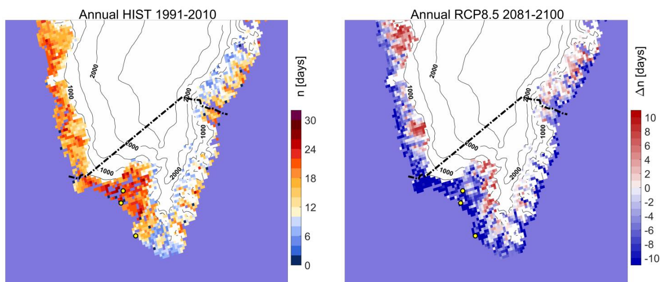
Figur 25. Antallet af vintersmeltedage i Sydgrønland i referenceperioden 1991-2010 til venstre. Til højre ses ændringen i antallet i 2081-2100 i forhold til 1991-2010 beregnet for RCP8.5-scenariet.
