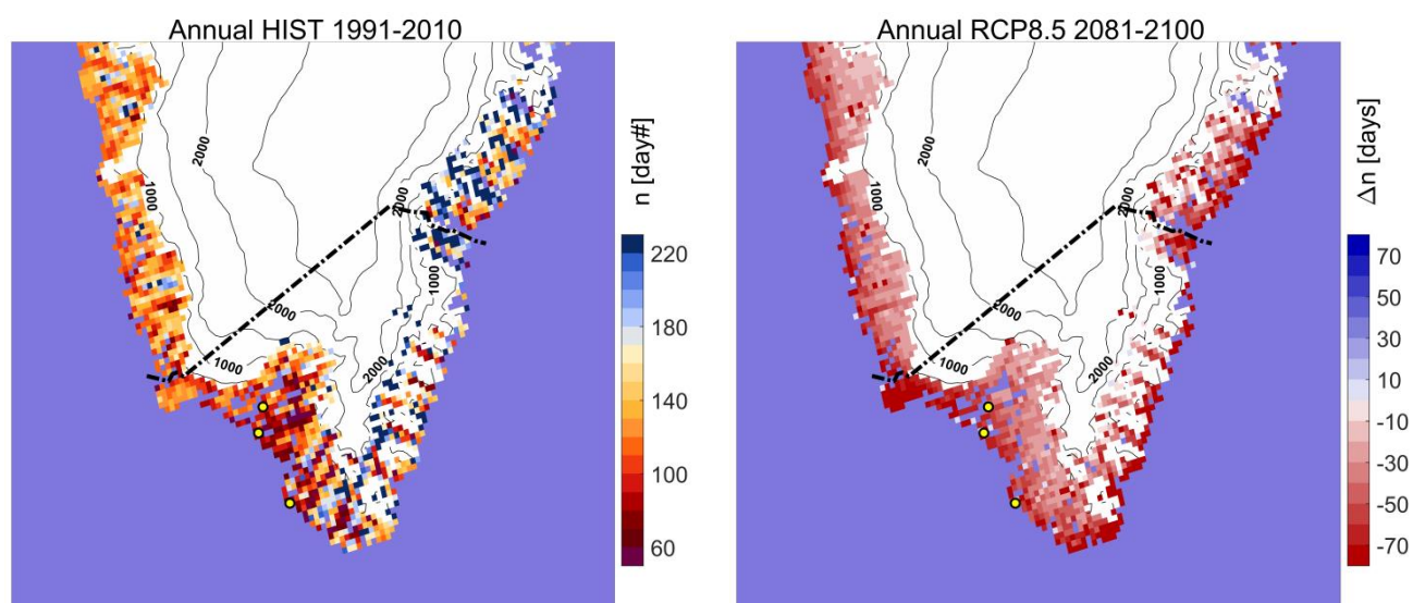
Figur 27. Snedækkets sæsonophør (kalenderdag) i Sydgrønland i referenceperioden 1991-2010 til venstre. Til højre ses ændringen i antal dage i 2081-2100 i forhold til 1991-2010 beregnet for RCP8.5-scenariet.
