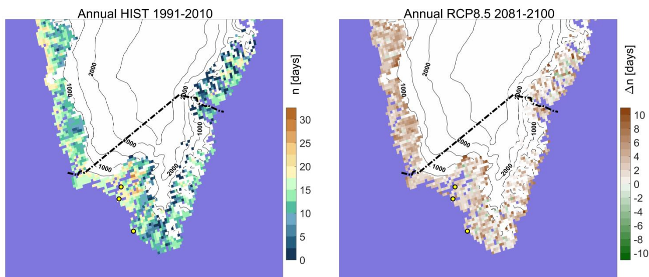
Figur 28. Den længste tørkeperiode (antal døgn) i Sydgrønland i løbet af vækstsæsonen i det nuværende klima (1991-2010) til venstre. Til højre er vist ændringen i antal dage i 2081-2100 i forhold til 1991-2010 beregnet for RCP8.5-scenariet.
