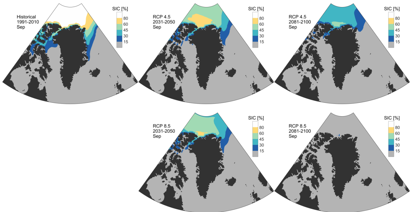
Figur 14. Gennemsnitlig september havisudbredelse i % baseret på klimamodeller i CMIP5. Der er lavet en middelværdi over i alt 29 modeller. Øverst til venstre: repræsenterende periode 1991-2010; øverst midt for: RCP 4.5 2031-2050; øverst til højre: RCP 4.5 2081-2100; nederst til venstre RCP8.5 2031-2050; nederst til højre: RCP8.5 2081-2100. Kilde: CMIP5 og DMI.
