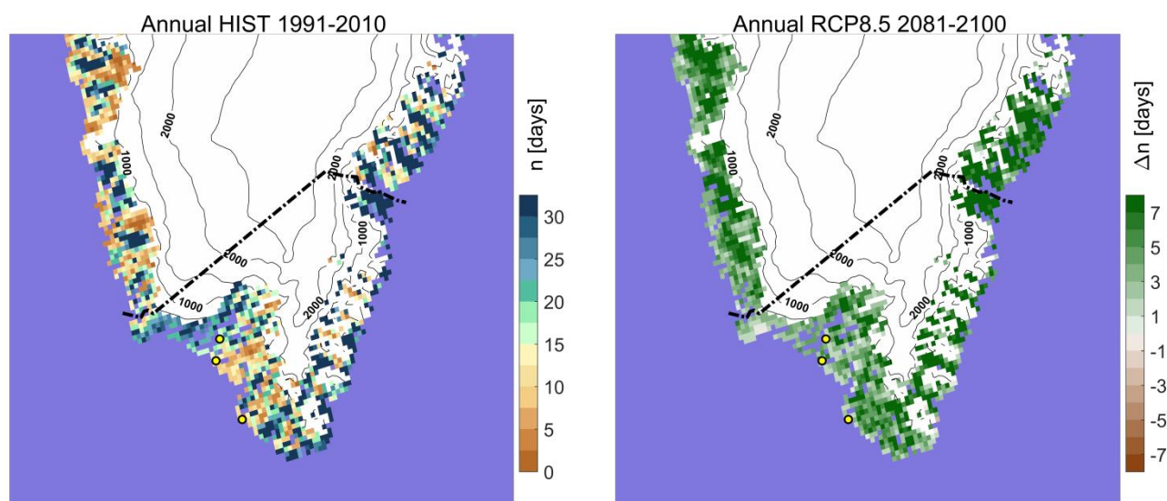
Figur 17. Ekstremnedbør. Antallet af døgne i løbet af et år med mere end 25mm nedbør i referenceperioden 1991-2010 til venstre. Til højre er vist ændringen i antal døgne med mere end 25 mm nedbør i 2081-2100 i forhold til 1991-2010 beregnet for RCP8.5-scenariet.
