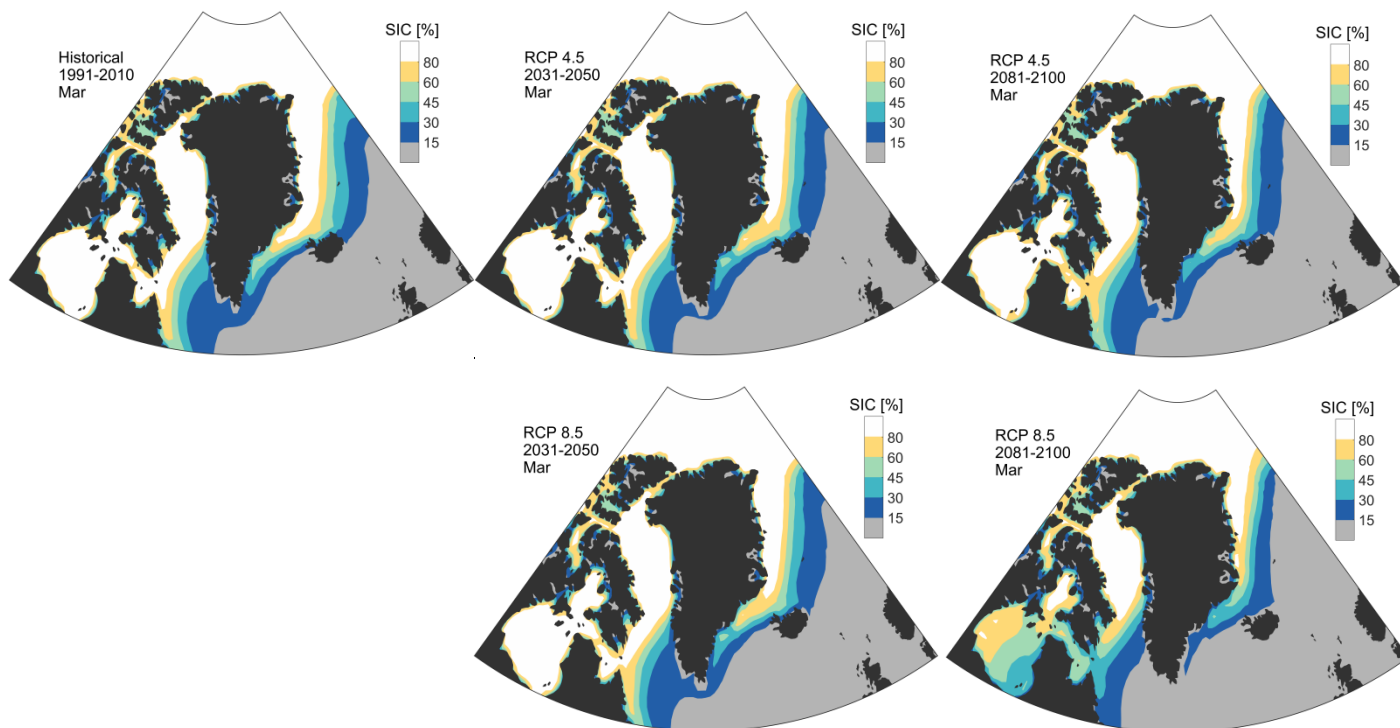
Figur 13. Gennemsnitlig marts havisudbredelse i % baseret på klimamodeller i CMIP5. Der er lavet en middelværdi over i alt 29 modeller. Øverst til venstre: repræsenterende periode 1991-2010; øverst midt for: RCP 4.5 2031-2050; øverst til højre: RCP4.5 2081-2100; nederst til venstre: RCP 8.5 2031-2050; nederst til højre: RCP8.5 2081-2100. Kilde CMIP5 og DMI
