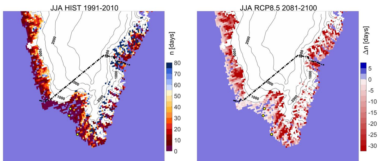
Figur 16. Forekomst af sommerfrost. Antallet af døgn i løbet juni-juli-august med minimum temperatur under 0 °C 1991-2010 til venstre. Til højre er vist ændringen i antal døgn i 2081-2100 i forhold til 1991-2010 beregnet for RCP8.5-scenariet.
