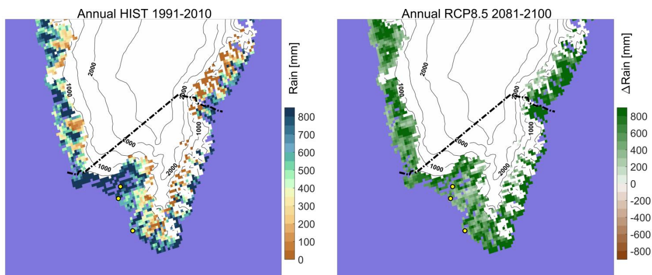
Figur 18. Årlig regnmængde opsummeret. Mængden af regn i løbet af et år i referenceperioden 1991-2010 til venstre i mm. Til højre er vist ændringen i årlig regnmængde i 2081-2100 i forhold til 1991-2010 beregnet for RCP8.5-scenariet.
