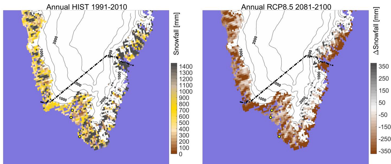
Figur 19. Årligt snefald. Mængden af sne der falder i løbet af et år i referenceperioden 1991-2010 til venstre angivet i mm per år. Til højre er vist ændringen i årligt snefald i 2081-2100 i forhold til 1991-2010 beregnet for RCP8.5-scenariet.
