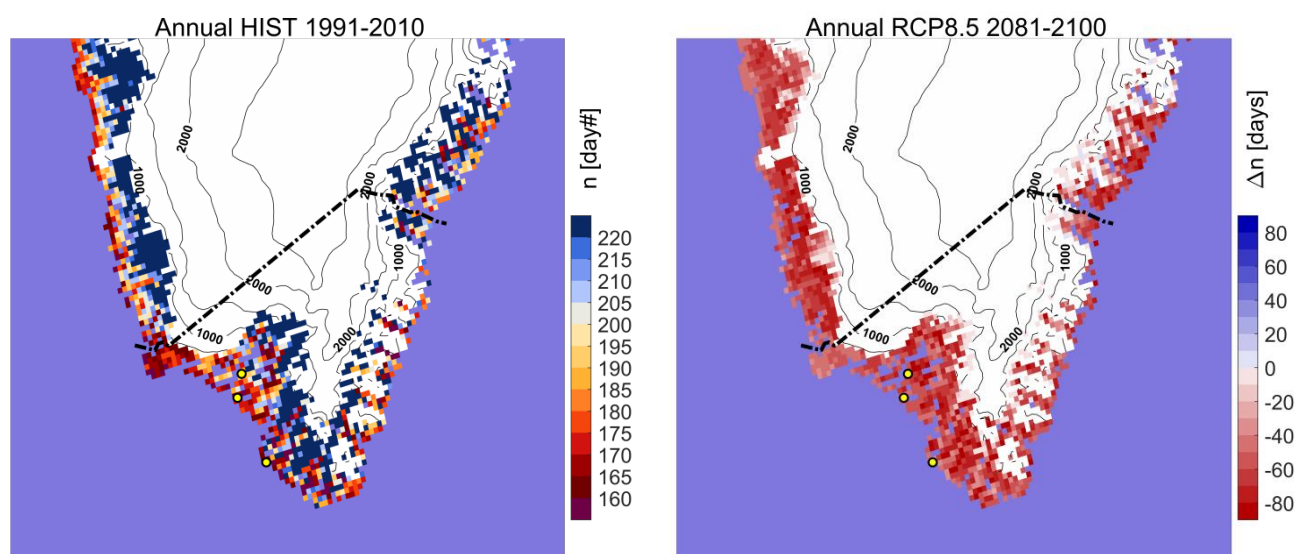
Figur 22. Årets sidste dag med forårsfrost (kalenderdag) i referenceperioden 1991-2010 til venstre. Til højre ses ændringen i sidste forårsfrost (antal dage) i 2081-2100 i forhold til 1991-2010 beregnet for RCP8.5-scenariet.
