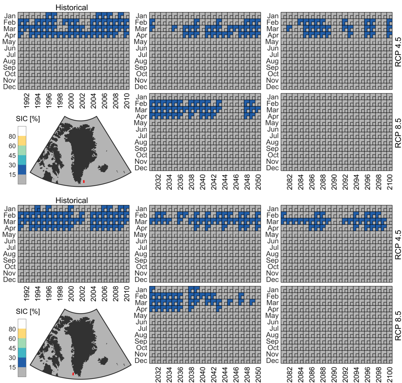
Figur 15. Forekomsten af storis øst for Sydgrønland (øverst) og vest for Sydgrønland (nederst) fordelt på måneds basis. Stor firkant repræsenterer information baseret på alle modeller, lille firkant (indsat) er for DMI's model. Kilde CMIP5 og DMI.
