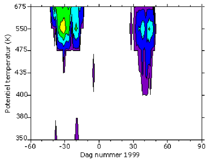
Figur 24b. Areal af den nordlige halvkugle dækket af PSC'ere i højdeinterval 350-675 K potentiel temperatur, svarende til ca. 14-26 km gennem vintrene 1999-2003.
