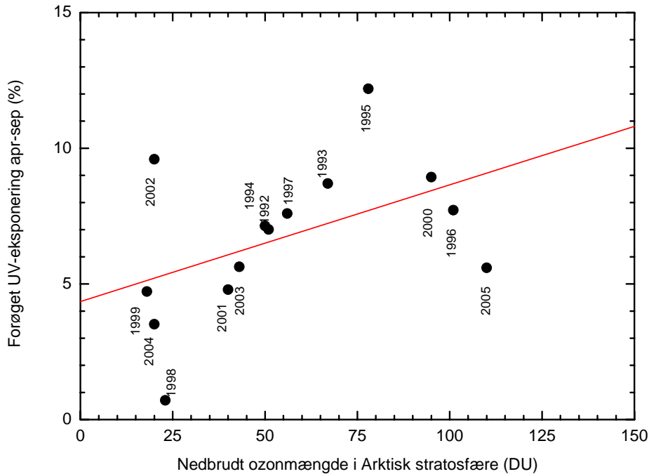
Figur 27. Beregnet sammenhæng mellem den ozonmængde der er nedbrudt i den arktiske stratosfære (14-24 km's højde) i perioden januar-marts og den forøgede UV-eksponering i Danmark i de efterfølgende 5 måneder (april-september). Som referenceniveau er anvendt middelværdien af ozonlaget tykkelse i 10-års perioden 1979-1988 (figur 4 og 5).
