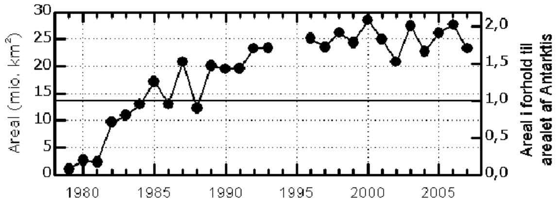
Figur 30. Det maksimale areal af det antarktiske ozonhul i perioden 1979-2007.
