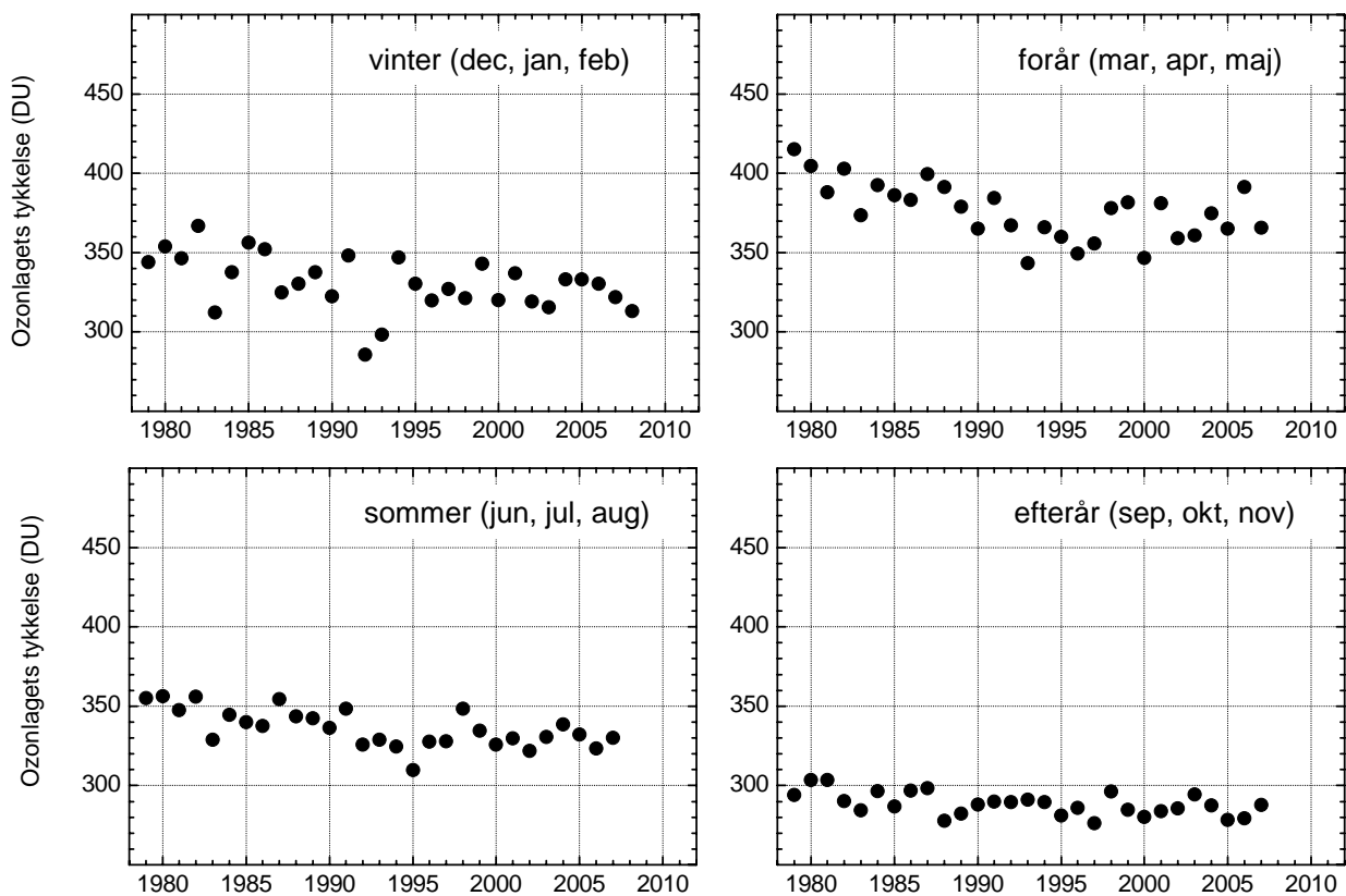
Figur 3. Ozonlagets sæsonmæssige middeltykkelse over Danmark for perioden 1979-2007. Data fra før 1993 er data fra NASA's TOMS-instrument på Nimbus7- satellitten. Data fra og med 1993 er DMI's målinger i København med et Brewer-instrument.
