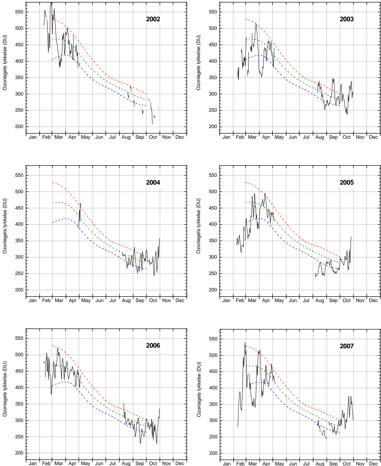
Figur 18. Ozonlagets tykkelse over Pituffik 2002-2007. Daglige målinger (sorte prikker) er DMI's målinger med SAOZ-spektrometeret. Den grønne linie angiver middelværdien af daglige målinger i ti-års perioden 1979-1988 målt med TOMS-instrumentet ombord på Nimbus7-satellitten. De blå og røde stiplede linier angiver plus og minus en standard afvigelse fra middelværdien. Det betyder, at 2/3 af alle målinger i perioden 1979-1988 ligger mellem den blå og den røde linie.
