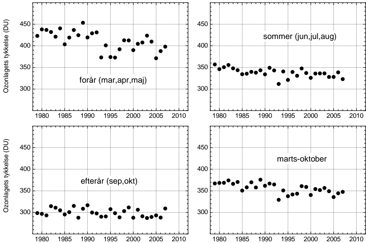
Figur 9. Ozonlagets sæsonmæssige middeltykkelse for Kangerlussuaq for perioden 1979-2007. Der kan kun måles i perioden fra midt i februar til slutningen af oktober. Efterår er derfor begrænset til to måneder, og den årlige middeltykkelse kan ikke bestemmes. En simpel lineær tilpasning af data for perioden 1979-2007 viser en signifikant nedadgående tendens for forår, sommer og hele måleperioden, men ikke for efteråret. Data fra før 1991 er data fra NASA's TOM- instrument på Nimbus7-satellitten, mens data fra og med 1991 er DMI's målinger med et Brewer-instrument.
