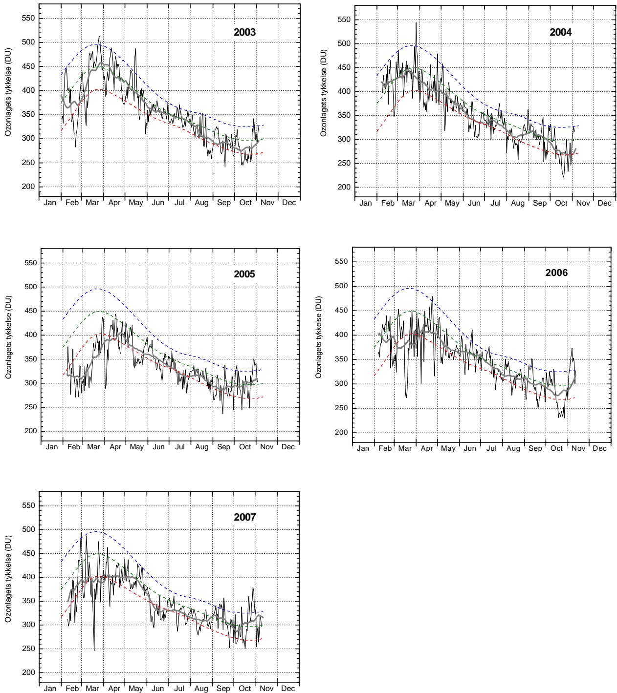
Figur 14. Ozonlagets tykkelse over Kangerlussuaq 2003-2007. Daglige målinger (tynd, sort linie) er DMI's målinger i Kangerlussuaq. Den grønne stiplede linie angiver middelværdien af daglige målinger i 10-års perioden 1979-1988, mens de blå og røde stiplede linier angiver henholdsvis middelværdien plus (blå) eller minus (rød) en standardafvigelse fra middelværdien. Det betyder, at ca. 2/3 af alle målinger i perioden 1979-1988 ligger mellem den blå og den røde linie. Den tykke grå linie er en 31-dages løbende middelværdi af de daglige målinger. En forholdsvis varm polar stratosfære i vintrene 2002-2003 og (især) 2003-2004 medfører ringe ozonnedbrydning.
