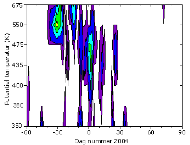
Figur 24c. Areal af den nordlige halvkugle dækket af PSC'ere i højdeinterval 350-675 K potentiel temperatur, svarende til ca. 14-26 km gennem vintrene 2004-2008.
