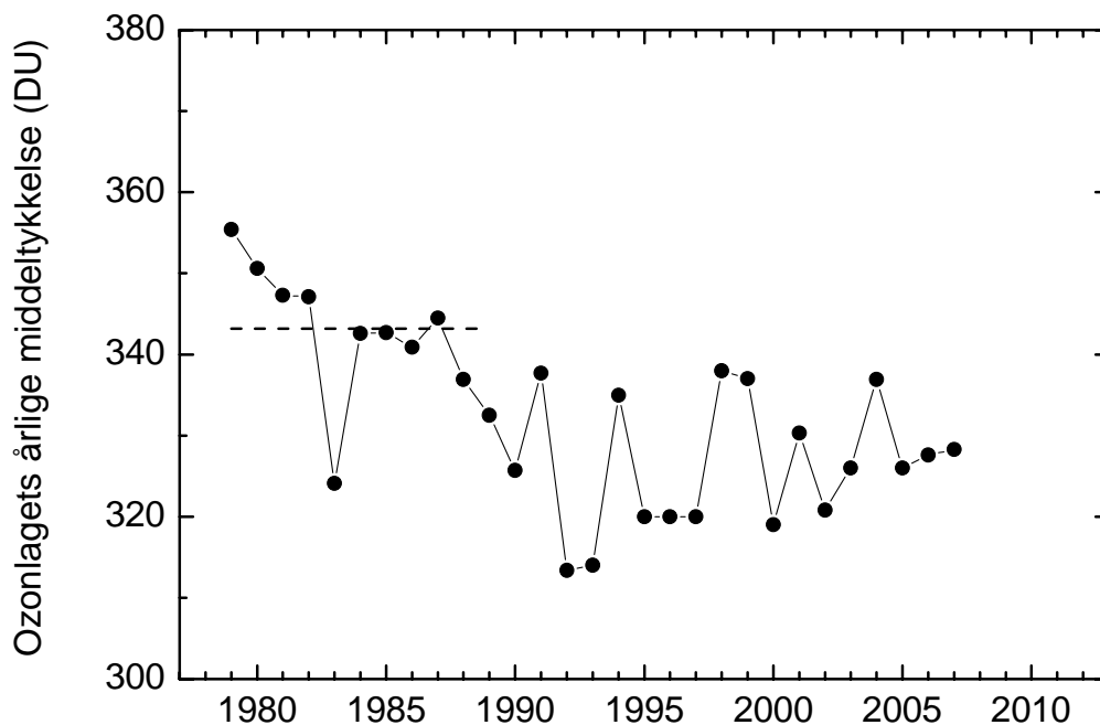
Figur 2. Ozonlagets årlige middeltykkelse over Danmark for perioden 1979-2007. Den gennemsnitlige årlige middelværdi for 10-års perioden 1979-1988 er 344 DU, vist med den stiplede linie. Betragtes alene de sidste 10 års data ses ingen tendens. Data fra før 1993 er data fra NASA's TOMS instrument på Nimbus7- satellitten. Data fra og med 1993 er DMI's målinger i København med et Brewer-instrument.
