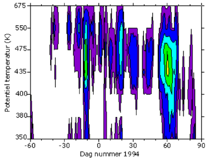
Figur 24a. Areal af den nordlige halvkugle dækket af PSC'ere i højdeinterval 350-675 K potentiel temperatur, svarende til ca. 14-26 km gennem vintrene 1994-1998.
