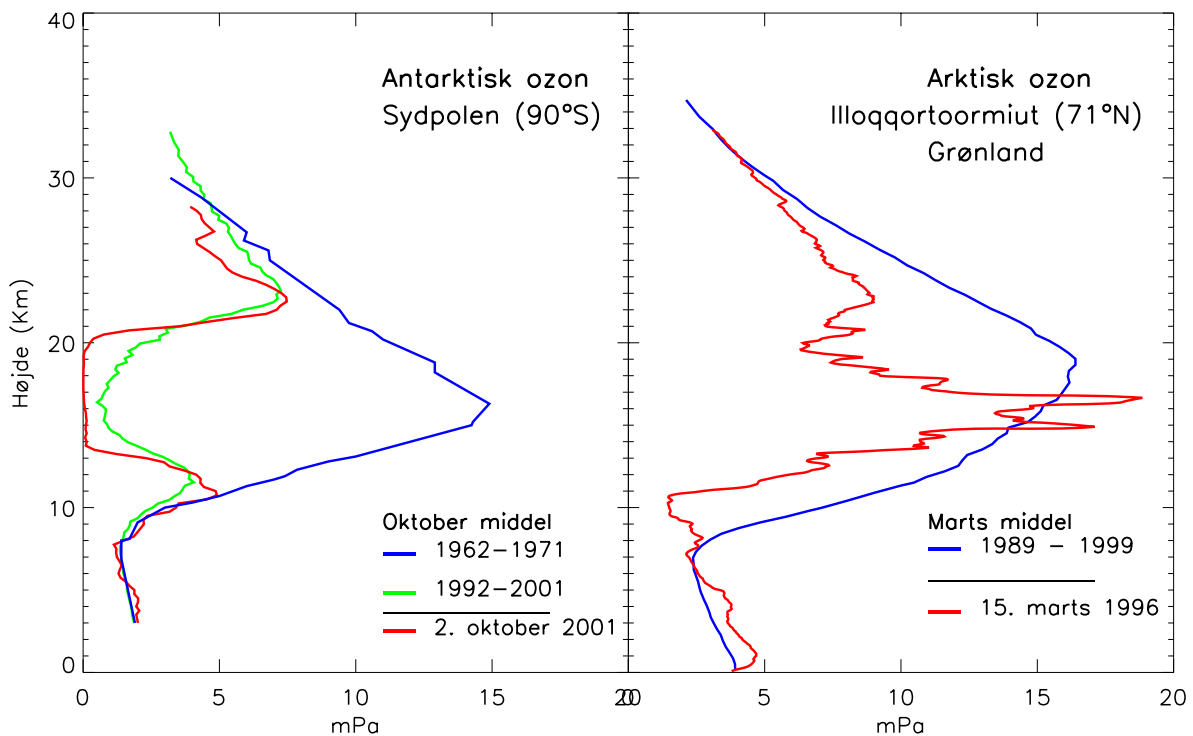
Figur 28. Højdeprofil af ozonnedbrydningen over Antarktis (til venstre) og Arktis (til højre). (WMO Assessment, 2002)
