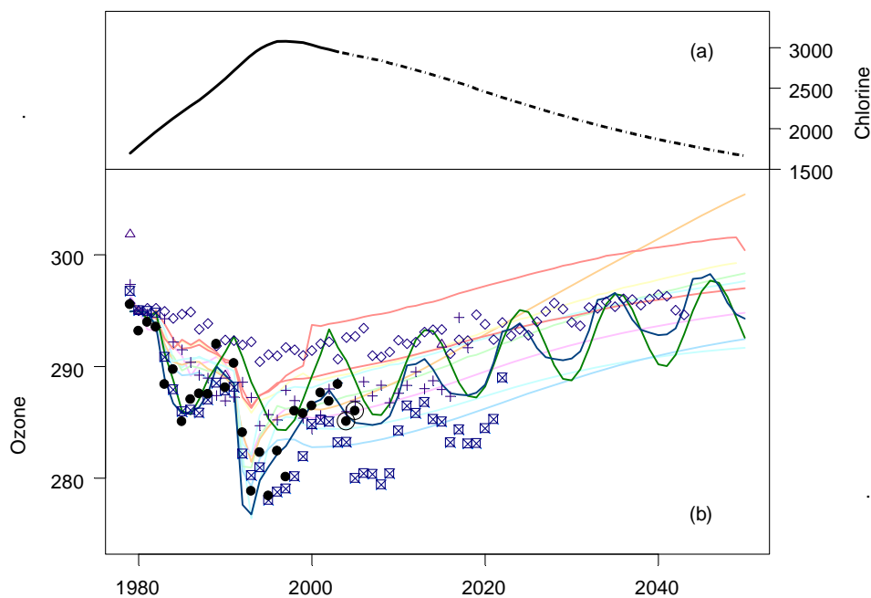
Figur A7. Øverst: Mængden af ozonnedbrydende stoffer som funktion af tiden. Den fuldt optrukne linie baserer sig på målinger, mens den stiplede linie viser den forventede udvikling, hvis Montreal-protokollen med tilføjelser overholdes. Nederst: Modelforudsigelser af fremtidens ozonlag midlet fra 60°S til 60°N. Linierne viser resultaterne fra to-dimensionelle modeller, symbolerne fra tre-dimensionelle modeller, og de sorte prikker er satellitobservationer. De meget lave værdier omkring 1993 skyldes udbruddet af vulkanen Mount Pinatubo på Filippinerne. Figuren er fra Weatherhead og Andersen, 2006.
