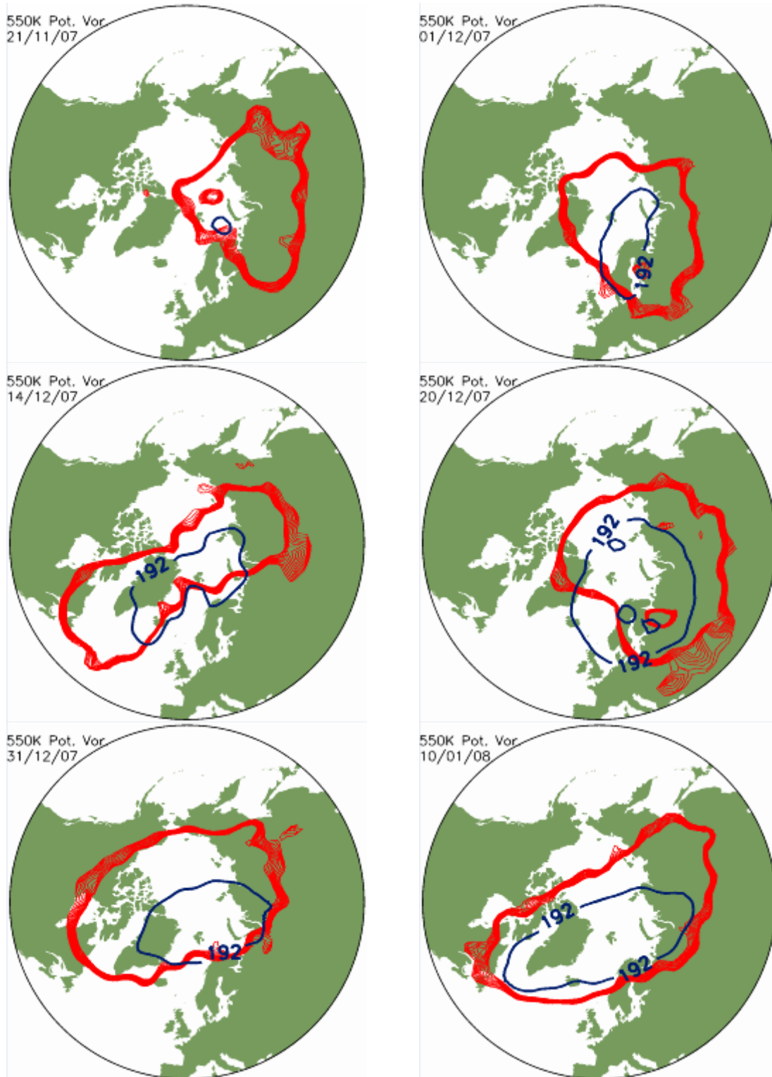
Figur 23 a. Røde konturlinier viser grænsen for den polare vortex i 550 K potentiel temperatur's højde, svarende til ca. 23 km, i perioden 21. november 2007-10. januar 2008. Blå konturlinier viser isothermen for dannelse af type 1 polar-stratosfæriske skyer.
