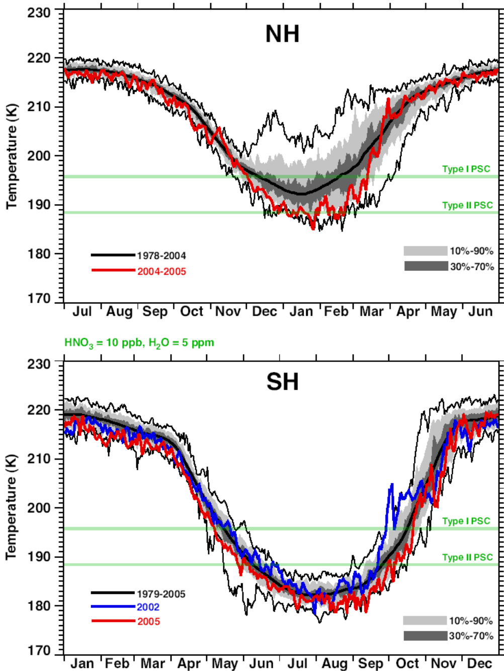
Figur 29. Årlig stratosfærisk temperatur cyklus og variabilitet i Arktis (NH) og Antarktis (SH). De grønne linier angiver temperaturen, hvorunder PSC'er kan dannes. Den sorte kurve angiver middeltemperaturen i perioden 1979-2004 (NH) og 1979-2005 (SH) med angivelse af rekordværdier (tynde sorte kurver). Den røde linie angiver udviklingen i Arktis (2004/2005) og Antarktis (2005) og 2002 (blå). Det grå areal angiver det interval, inden for hvilket procentdelen af observationerne falder. (WMO Assessment, 2007).
