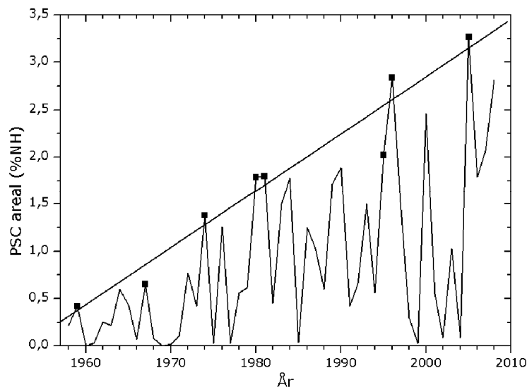
Figur 25. Det gennemsnitlige geografiske areal, dækket af polar-stratosfæriske skyer, i procent af den nordlige halvkugles areal siden 1958. Vintrene med de største PSC-arealer er markeret med kvadrater og danner grundlaget for regressionslinien.
