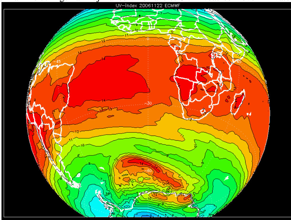
Figur 32. Beregnede UV-indices over det sydlige Atlanterhav 22. november 2006. Bemærk de kraftigt forhøjede UV-niveauer ved 60°S i forbindelse med det antarktiske ozonhul.
