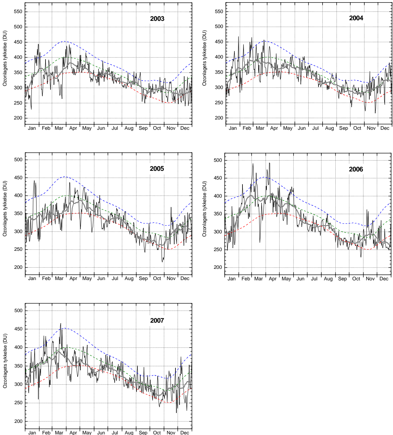
Figur 8. Ozonlagets tykkelse over Danmark 2003-2007. Daglige målinger (tynd, sort linie) er DMI's målinger i København. Den grønne stiplede linie angiver middelværdien af daglige målinger i 10-års perioden 1979-1988, mens de blå og røde stiplede linier angiver henholdsvis middelværdien plus (blå) eller minus (rød) en standardafvigelse fra middelværdien. Det betyder, at ca. 2/3 af alle målinger i perioden 1979-1988 ligger mellem den blå og den røde linie. Den tykke grå linie er en 31-dages løbende middelværdi af de daglige målinger. En forholdsvis varm polar stratosfære i vintrene 2002-2003 og (især) 2003-2004 med deraf følgende ringe ozonnedbrydning sætter sine spor i de følgende forår og somre med forholdsvis normalt ozonlag.
