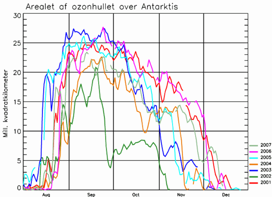
Figur 31. Udviklingen i det antarktiske ozonhuls areal de seneste 7 år.
