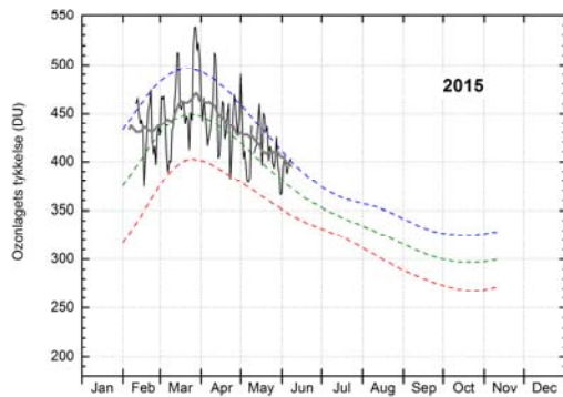
Figur A2g. Ozonlagets tykkelse over Kangerlussuaq forår 2015. Daglige målinger (tynd, sort linje) er DMI's målinger i Kangerlussuaq. Den grønne stiplede linje angiver middelværdien af daglige målinger i 10-års perioden 1979-1988, mens de blå og røde stiplede linjer angiver henholdsvis middelværdien plus (blå) eller minus (rød) en standardafvigelse fra middelværdien. Det betyder, at ca. 2/3 af alle målinger i perioden 1979-1988 ligger mellem den blå og den røde linje. Den tykke grå linje er en 31-dages løbende middelværdi af de daglige målinger.
