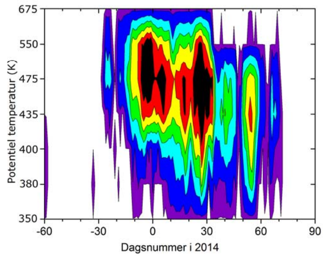
Figur A4e. Areal af den nordlige halvkugle dækket af PSC'ere i højdeinterval 350-675 K potentiel temperatur, svarende til ca. 14-26 km gennem vinteren 2014-2015.
