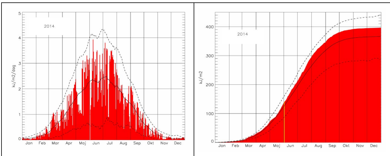
Figur 11 . (Venstre panel) Den dagligt målte totale dosis af hudskadelig UV stråling i 2014 i København i kJ/m 2 /dag. Fuldt optrukken kurve er den tilsvarende middel-dosis for 2000-2010. Øvre og nedre punkterede kurver viser hhv. +2 og -2 standardafvigelser. (Højre panel) Den totale dosis i løbet af året af hudskadelig UV stråling i 2014 i København i kJ/m 2 . Fuldt optrukken kurve er den tilsvarende middel-dosis for 2000-2010. Øvre og nedre punkterede kurver viser hhv. +2 og -2 standardafvigelser.
