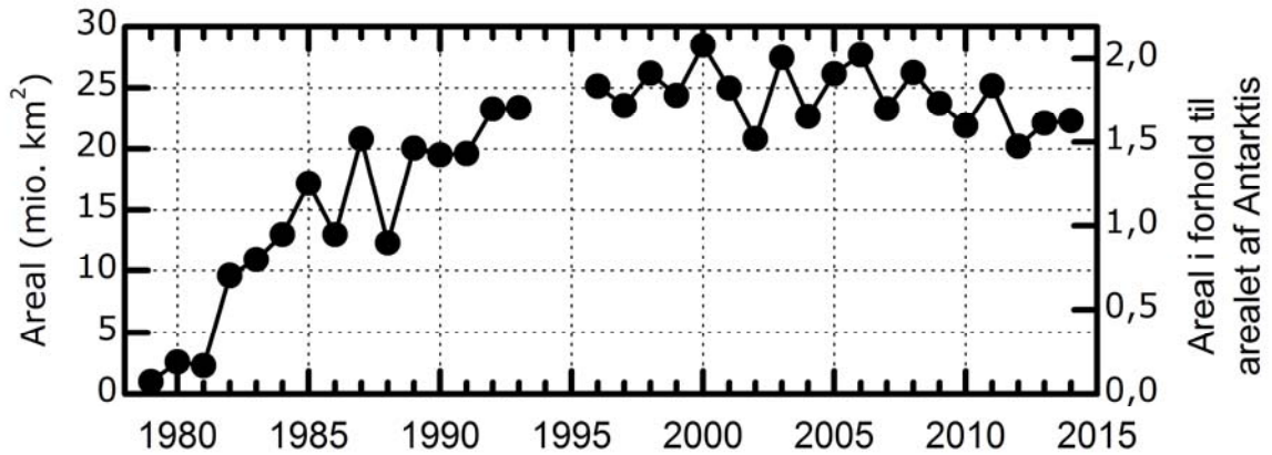
Figur14. Det maksimale areal af det antarktiske ozonhul i perioden 1979-2014.
