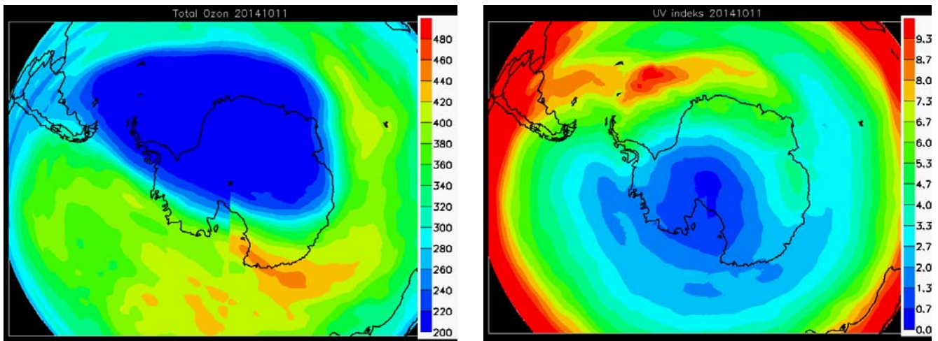
Figur 16. Beregnede UV-indices over det sydlige Amerika 11.oktober 2014 (højre panel) i forbindelse med det antarktiske ozonhul (venstre panel, DU).
