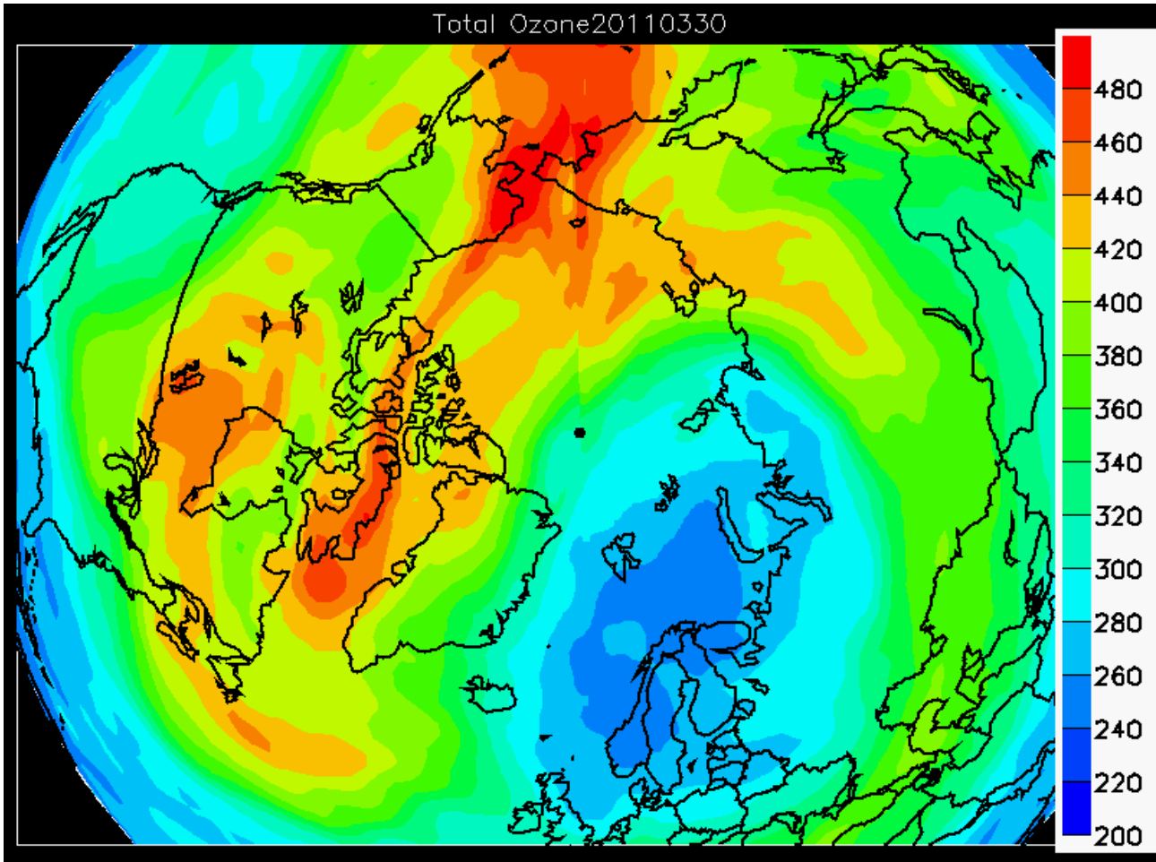
Figur E3. Ozonlagets tykkelse (DU) over den nordlige halvkugle 30. marts 2011, observeret fra Gome-2 instrument ombord på Eumetsat's MetOp satellit. Vorticitet er drejet ind over Skandinavien, og inden for vorticitet måles de lave tykkelser af ozonlaget ned til omkring 250 DU.
