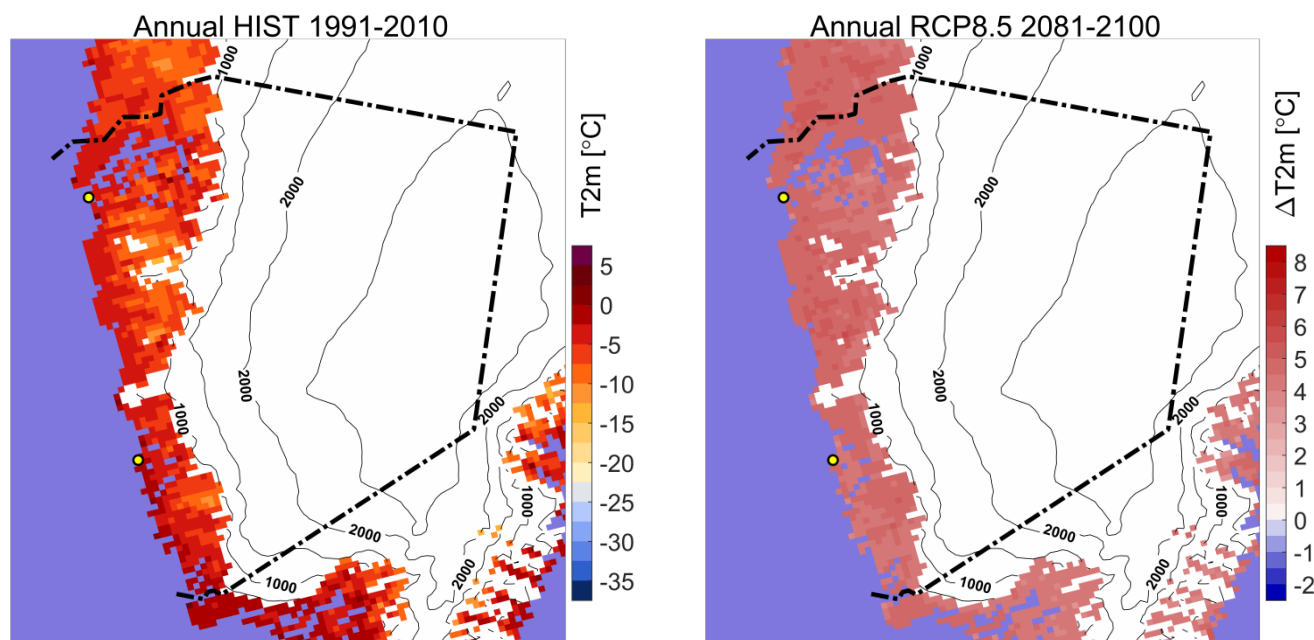
Figur 5. Modelleret årlig middeltemperatur for Nuuk-Paamiut området. Middeltemperaturen i referenceperioden 1991-2010 til venstre. Til højre er vist ændringen i middeltemperatur i 2081-2100 i forhold til 1991-2010 beregnet for RCP8.5-scenariet.
