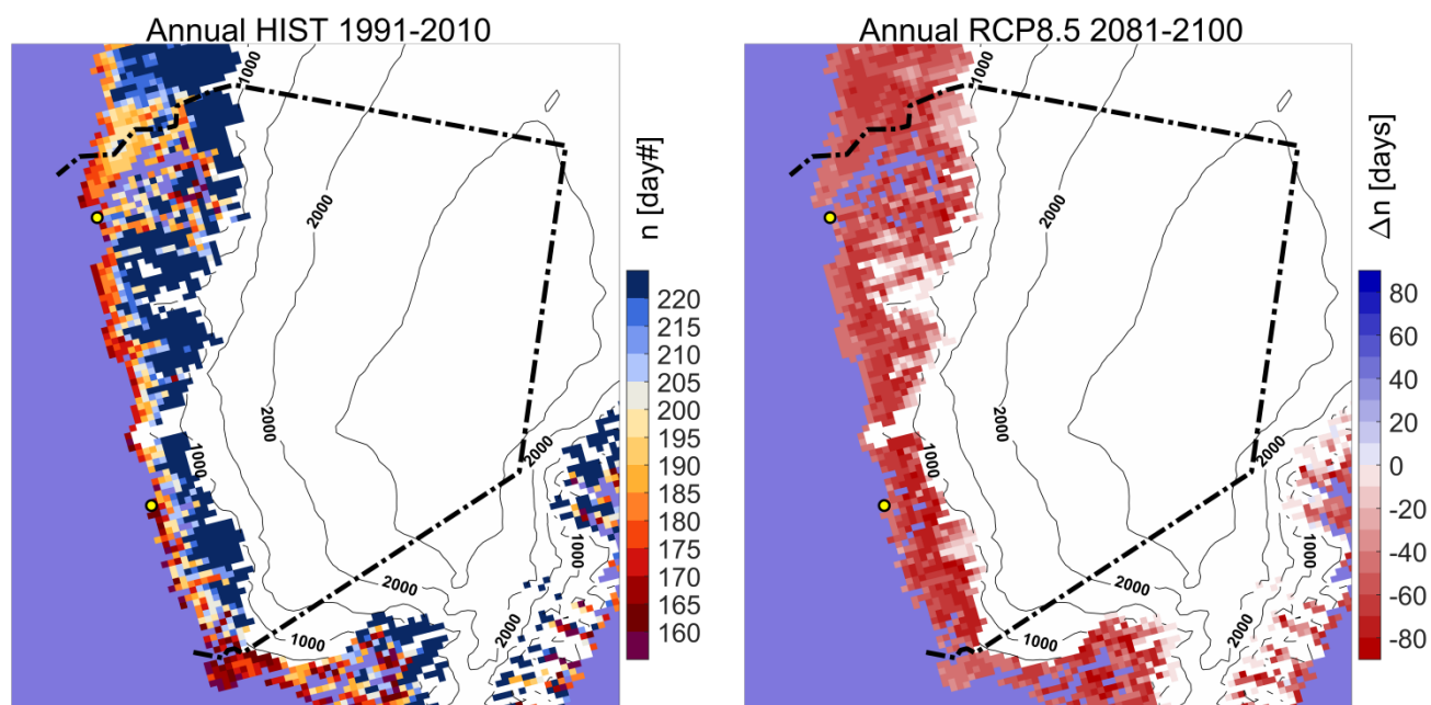
Figur 21. Årets sidste dag med forårsfrost (kalenderdag) i referenceperioden 1991-2010 til venstre. Til højre ses ændringen i sidste forårsfrostdag (antal dage) i 2081-2100 i forhold til 1991-2010 beregnet for RCP8.5-scenariet.
