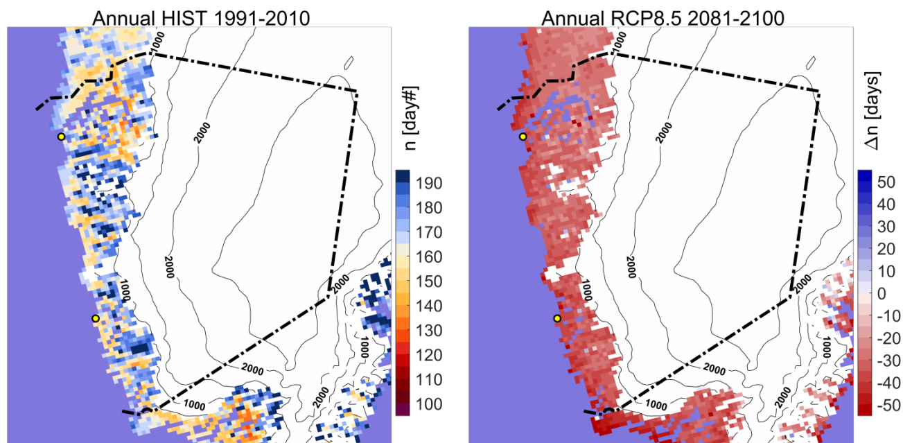
Figur 20. Vækstsæsonens begyndelsestidspunkt i referenceperioden 1991-2010 som kalenderdag til venstre. Til højre ses ændringen i vækstsæsonens begyndelsestidspunkt (antal dage) i 2081-2100 i forhold til 1991-2010 beregnet for RCP8.5-scenariet.
