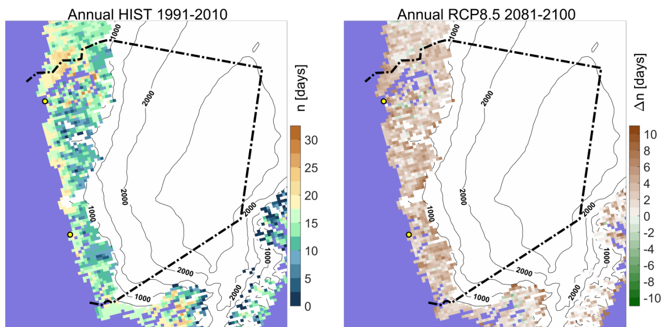
Figur 27. Den længste tørkeperiode (antal døgn) i Nuuk-Paamiut området i løbet af vækstsæsonen i det nuværende klima (1991-2010) til venstre. Til højre er vist ændringen i antal dage i 2081-2100 i forhold til 1991-2010 beregnet for RCP8.5-scenariet.
