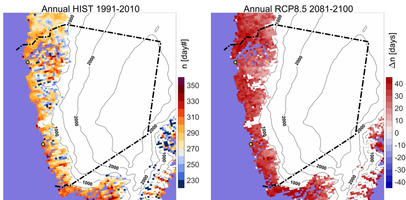
Figur 25. Snedækkets sæsonstart (kalenderdag) i Nuuk-Paamiut området i referenceperioden 1991-2010 til venstre. Til højre ses forskydningen i antal dage i 2081-2100 i forhold til 1991-2010 beregnet for RCP8.5-scenariet.
