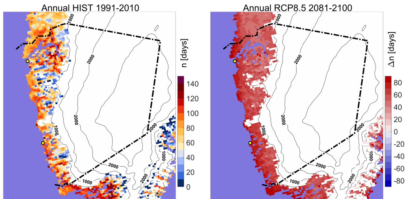
Figur 22. Vækstsæsonens længde i Nuuk-Paamiut området i referenceperioden 1991-2010 til venstre. Til højre ses ændringen i vækstsæsonens længde (antal dage) i 2081-2100 i forhold til 1991-2010 beregnet for RCP8.5-scenariet.
