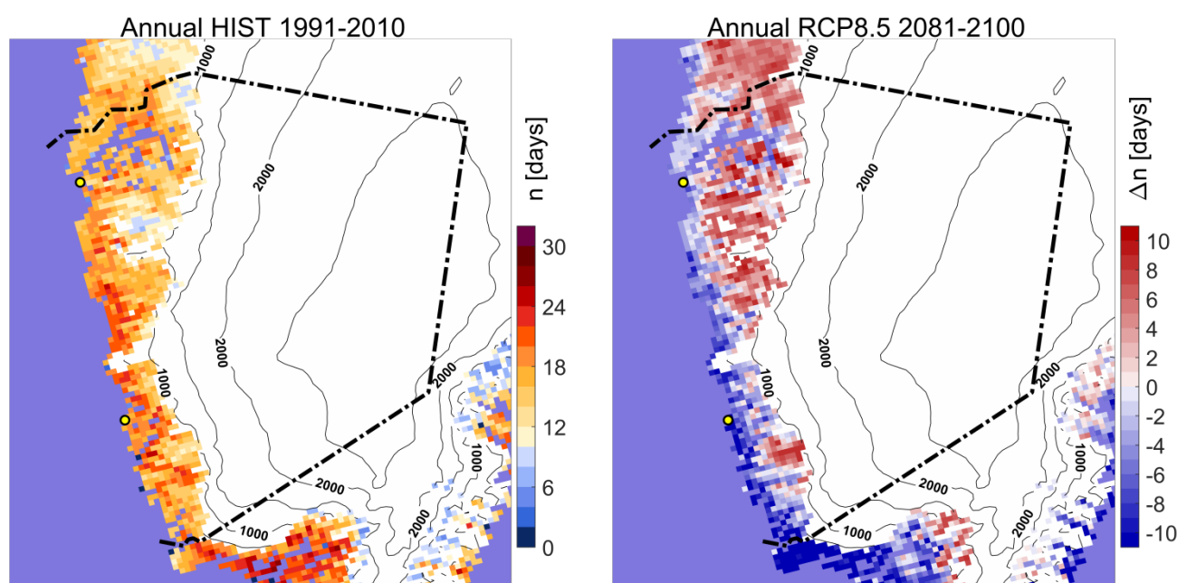
Figur 24. Antallet af vintersmeltedage i Nuuk-Paamiut området i referenceperioden 1991-2010 til venstre. Til højre ses ændringen i antallet i 2081-2100 i forhold til 1991-2010 beregnet for RCP8.5-scenariet.
