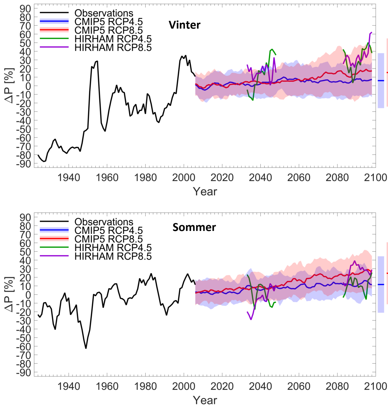
Figur 8. Procentvise nedbørsændringer i Nuuk-Paamiut området som i figur 7 men for vinter (øverst) og sommer (nederst).
