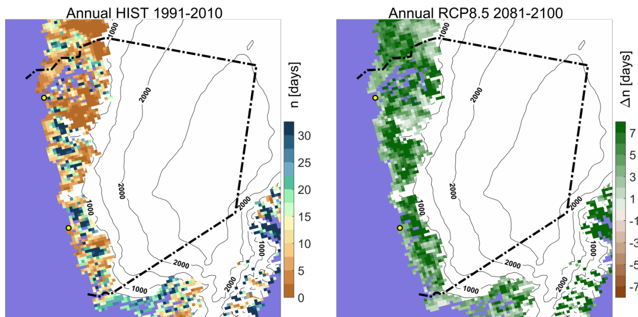
Figur 16. Ekstremnedbør. Antallet af døgnetil i løbet af et år med mere end 25 mm nedbør i referenceperioden 1991-2010 til venstre. Til højre er vist ændringen i antal døgnetil med mere end 25 mm nedbør i 2081-2100 i forhold til 1991-2010 beregnet for RCP8.5-scenariet.
