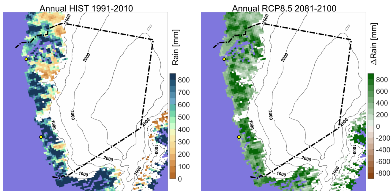
Figur 17. Årlig regnmængde opsummeret. Mængden af regn i løbet af et år i referenceperioden 1991-2010 til venstre i mm. Til højre er vist ændringen i årlig regnmængde i 2081-2100 i forhold til 1991-2010 beregnet for RCP8.5-scenariet.
