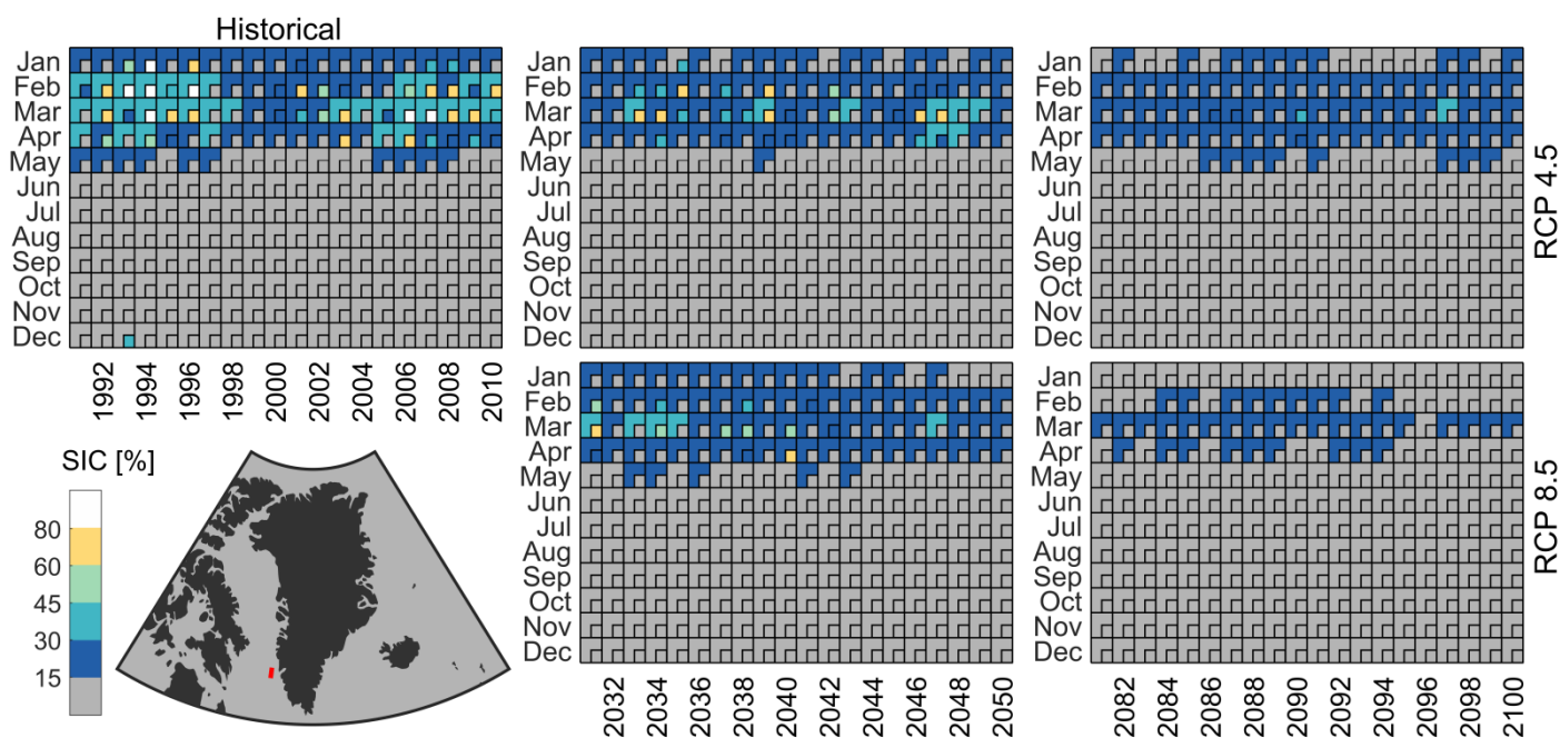
Figur 14. Forekomsten af havis vest for Nuuk fordelt på måneds basis. Stor firkant repræsenterer information baseret på alle modeller, lille firkant (indsat) er for DMI's model. Kilde CMIP5 og DMI.
