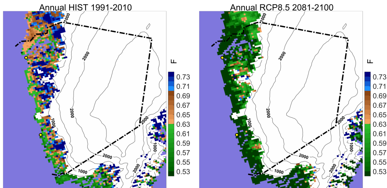
Figur 23. Permafrostindeks i Nuuk-Paamiut området i referenceperioden 1991-2010 til venstre. Til højre ses Permafrostindekset i 2081-2100 beregnet for RCP8.5-scenariet.
