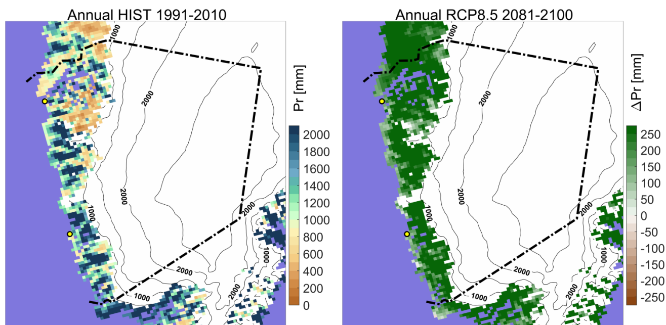
Figur 9. Nedbørsum. Den modelbaserede samlede årlige nedbørsum i referenceperioden 1991-2010 til venstre. Til højre er vist ændringen i årlig nedbørsum i 2081-2100 i forhold til 1991-2010 beregnet for RCP8.5-scenariet.
