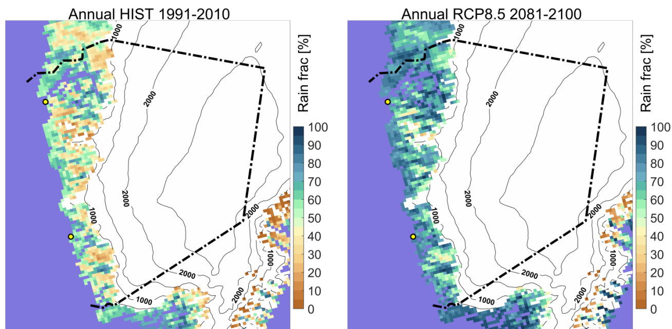
Figur 19. Årlig andel af nedbøren, der falder som regn i det nuværende klima 1991-2010 til venstre angivet i procent. Til højre ses den procentvise andel for 2081-2100 beregnet for RCP8.5-scenariet.
