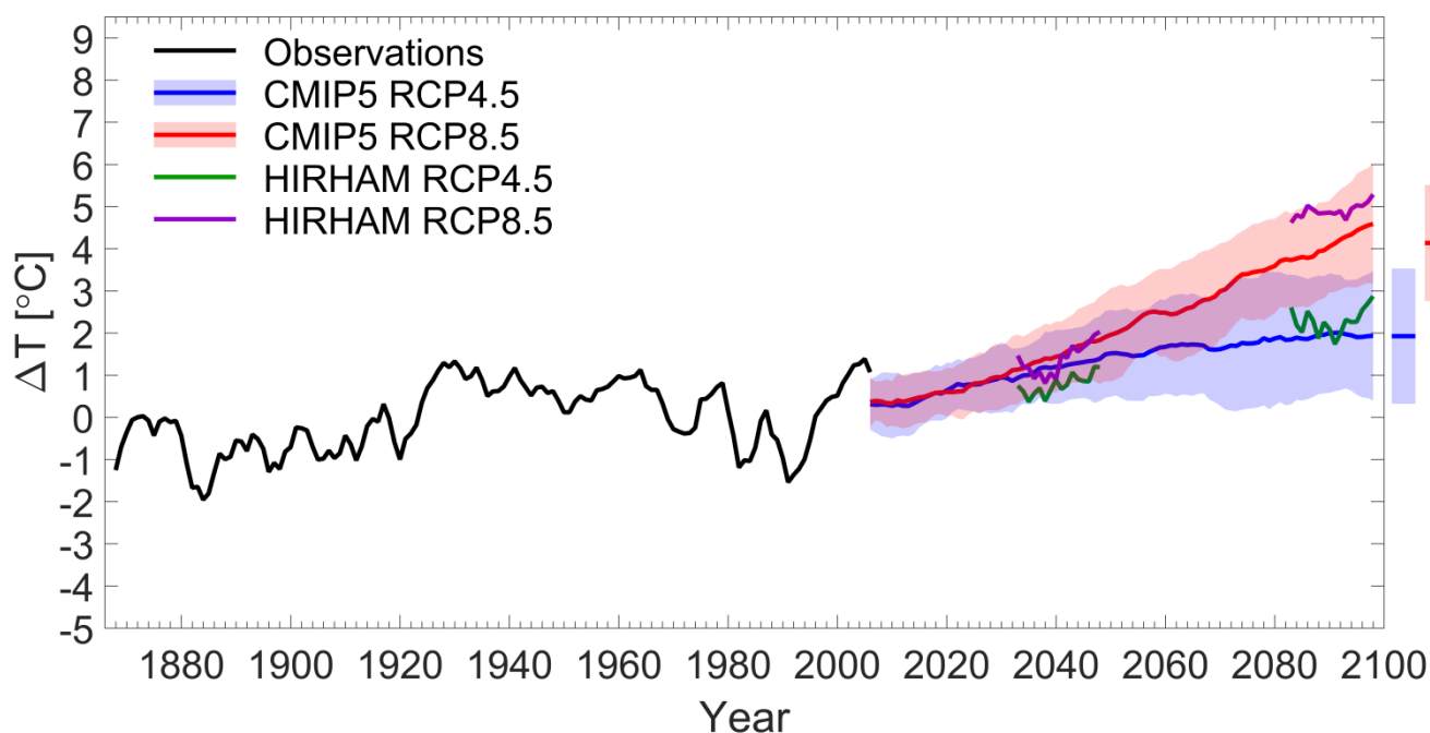
Figur 3. Årlig udvikling i middeltemperatur for Nuuk-Paamiut området i forhold til referenceperioden 1986-2005. Sort kurve: Observationer fra 1866 til 2005 i Nuuk. Blå og rød kurve: Modellsimulering for perioden 2006-2100 for henholdsvis RCP4.5-scenariet og RCP8.5-scenariet. De skraverede lysere farvede områder angiver vurderede nøjagtigheder på temperaturstigningerne. For de samme scenarier er med hhv. grøn og violet angivet resultater baseret på DMI's detaljerede klimamodel for Grønland, som kun har regnet for forskellige tidsudsnit. For alle scenariekurverne er der anvendt et glidende 5-års-middel. Til højre ses middeltemperaturstigningerne for de sidste 20 år (2081 – 2100) af simuleringerne. Kilde: Observationsdata: DMI; Modellsimuleringer: CMIP5 og DMI.
