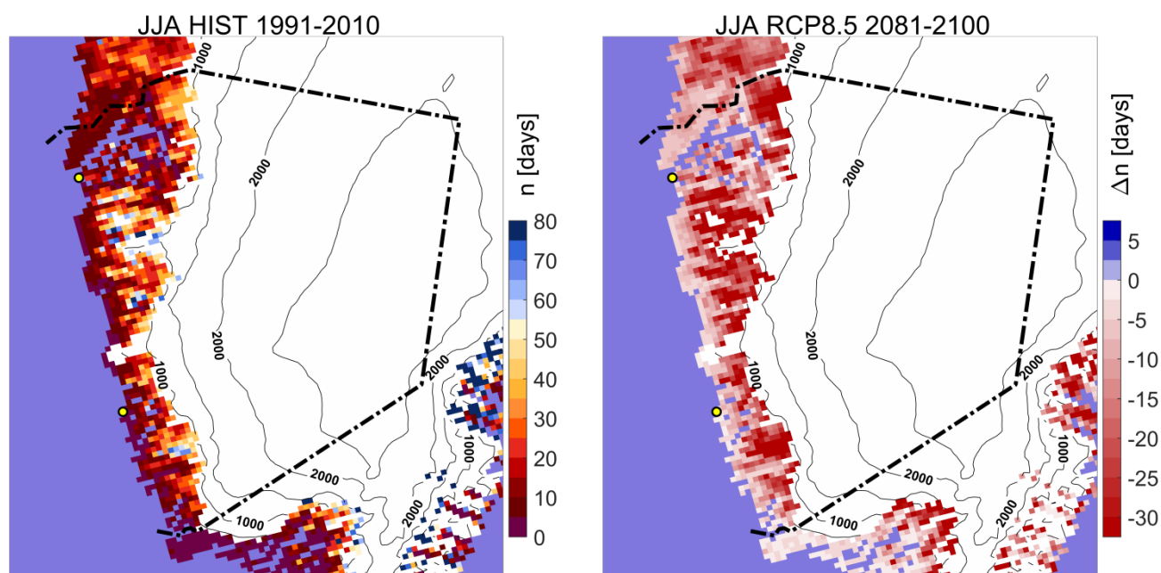
Figur 15. Forekomst af sommerfrost. Antallet af døgn i løbet juni-juli-august med minimum temperatur under 0 °C 1991-2010 til venstre. Til højre er vist ændringen i antal døgn i 2081-2100 i forhold til 1991-2010 beregnet for RCP8.5-scenariet.
