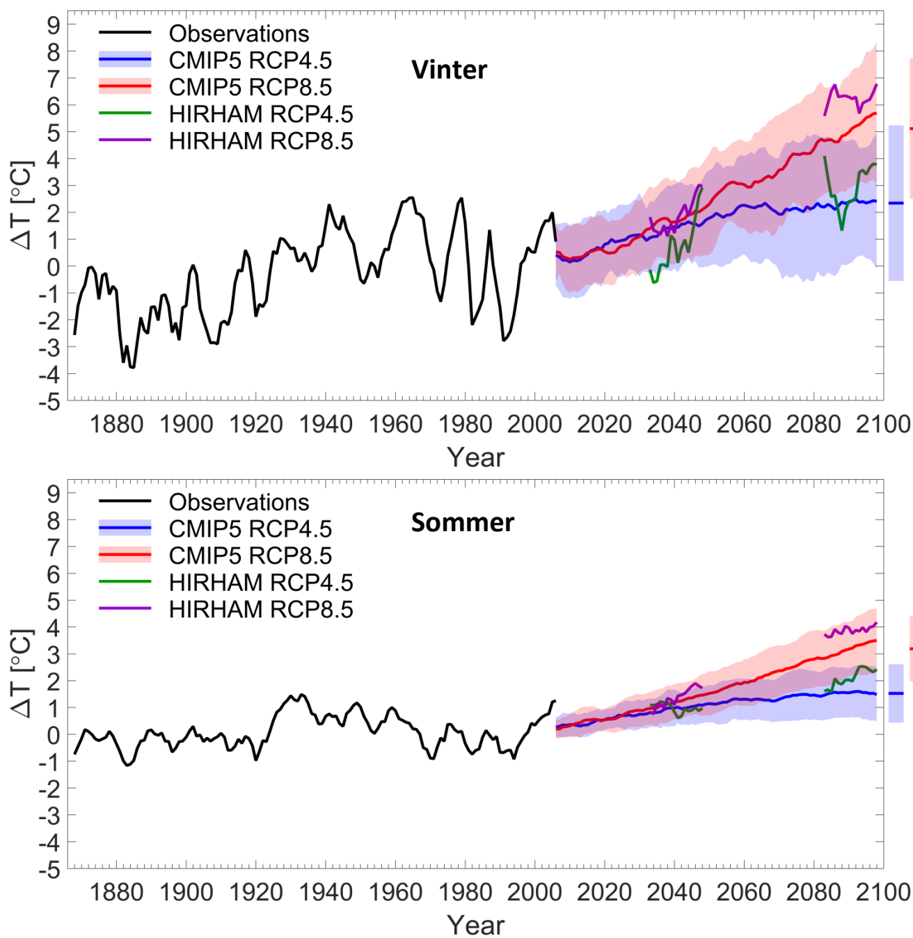
Figur 4. Temperaturændringer i Nuuk-Paamiut området som i figur 3 men for vinter (øverst) og sommer (nederst).
