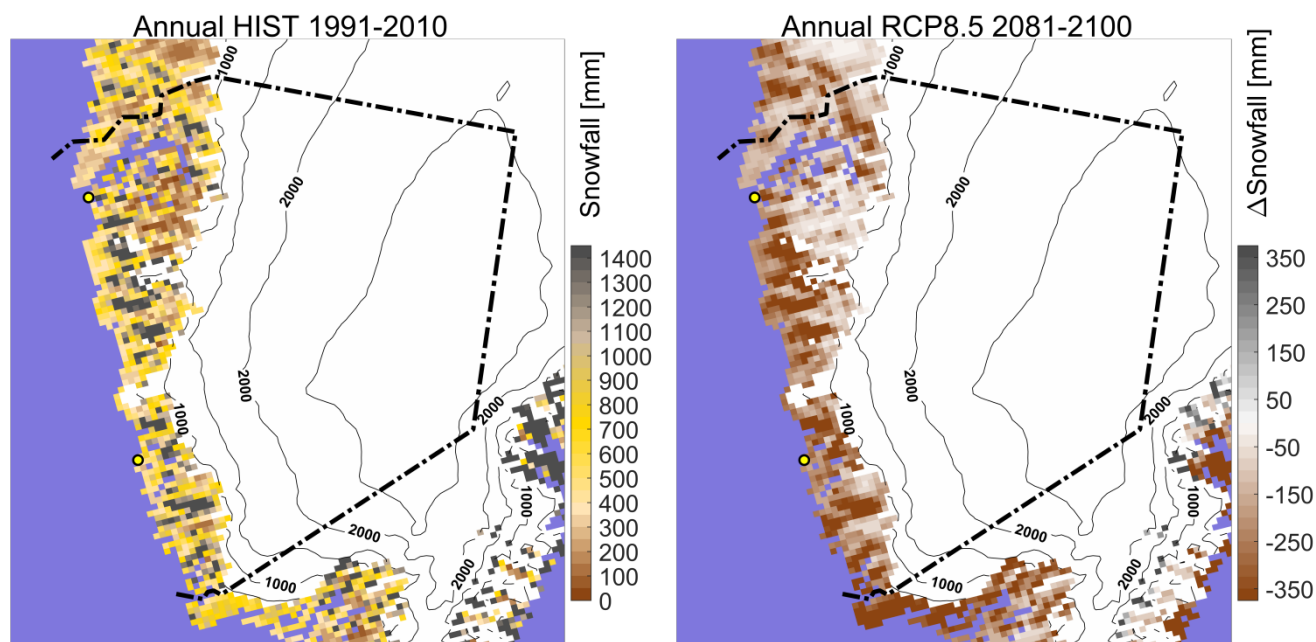
Figur 18. Årligt snefald. Mængden af sne der falder i løbet af et år i referenceperioden 1991-2010 til venstre angivet i mm per år. Til højre er vist ændringen i årligt snefald i 2081-2100 i forhold til 1991-2010 beregnet for RCP8.5-scenariet.
