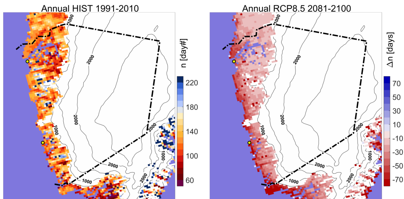
Figur 26. Snedækkets sæsonophør (kalenderdag) i Nuuk-Paamiut området i referenceperioden 1991-2010 til venstre. Til højre ses ændringen i antal dage i 2081-2100 i forhold til 1991-2010 beregnet for RCP8.5-scenariet.
