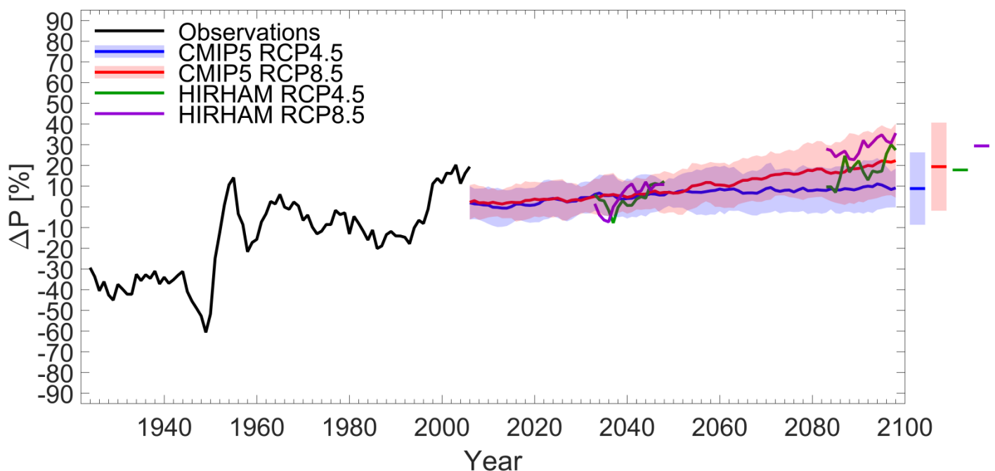
Figur 7. Procentvise årlige nedbørsændringer i Nuuk-Paamiut området i forhold til referenceperioden 1986-2005. Sort kurve: Observationer fra 1922 til 2005 i Nuuk. Blå og rød kurve: Modelsimulering for perioden 2006-2100 for henholdsvis RCP4.5-scenariet og RCP8.5-scenariet. De skraverede lysere farvede områder omkring angiver vurderede nøjagtigheder på nedbørændringerne. For de samme scenarier er med hhv. grøn og violet angivet resultater baseret på DMI's detaljerede klimamodel for Grønland, som kun har beregnet forskellige tidsudsnit. For alle scenarie-kurverne er der anvendt et glidende 5-års-middel. Til højre ses middelændringerne for de sidste 20 år (2081 – 2100) af simuleringerne. Kilde: Observationsdata: DMI; Modelsimuleringer: CMIP5 og DMI.
