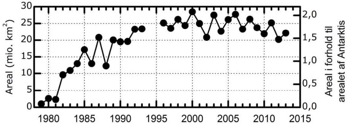
Figur14. Det maksimale areal af det antarktiske ozonhul i perioden 1979-2013.
