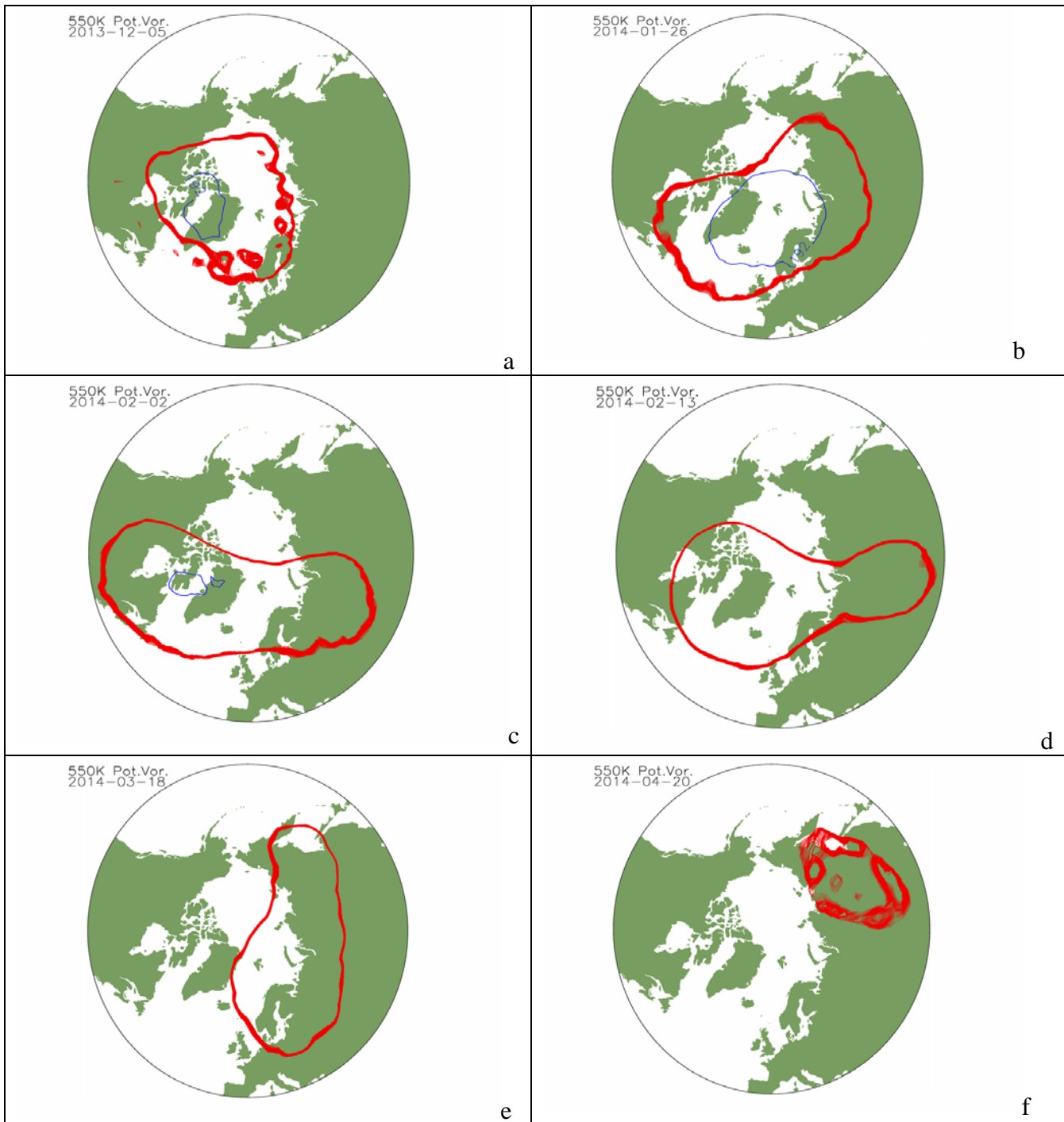
Figur 7. Røde konturlinjer viser grænsen for den polare vortex i 550 K potentiel temperaturs højde, svarende til ca. 23 km, i perioden 5. december 2013 – 20. april 2014. Blå konturlinjer viser isotermerne for dannelse af type 1 polar-stratosfæriske skyer.
