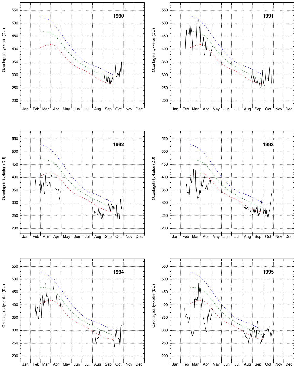
Figur A3a. Ozonlagets tykkelse over Pituffik 1990-1995. Daglige målinger med SAOZ-spektrometeret. Den grønne linje angiver middelværdien af daglige målinger i ti-års perioden 1979-1988 målt med TOMS-instrumentet ombord på Nimbus7-satellitten. De blå og røde stiplede linjer angiver plus og minus en standardafvigelse fra middelværdien. Det betyder, at 2/3 af alle målinger i perioden 1979-1988 ligger mellem den blå og den røde linje.
