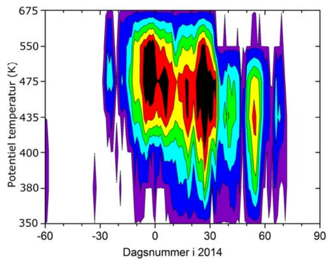
Figur A4e. Areal af den nordlige halvkugle dækket af PSC'ere i højdeinterval 350-675 K potentiel temperatur, svarende til ca. 14-26 km gennem vinteren 2014.
