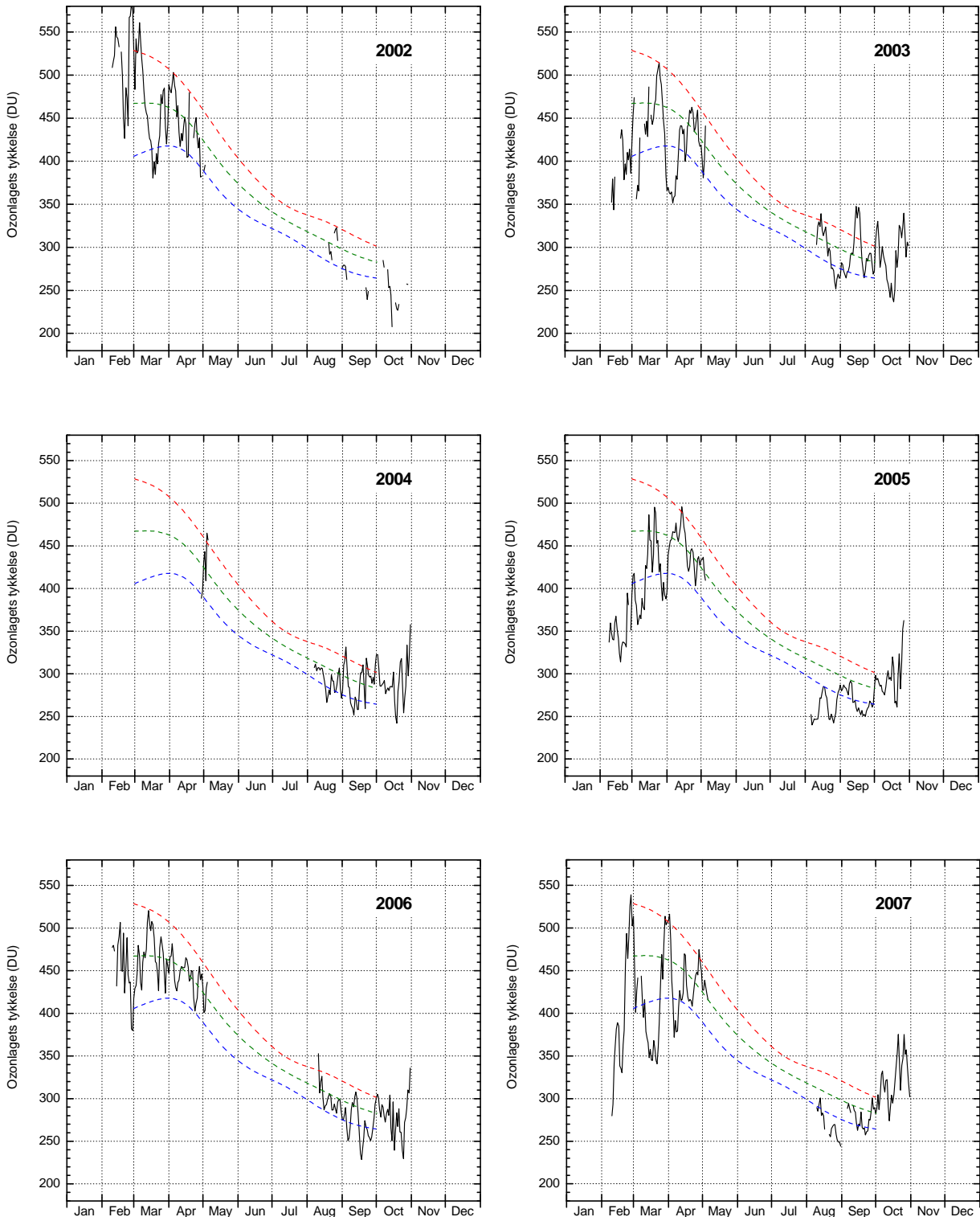
Figur A3c. Ozonlagets tykkelse over Pituffik 2002-2007. Daglige målinger med SAOZ-spektrometeret. Den grønne linje angiver middelværdien af daglige målinger i ti-års perioden 1979-1988 målt med TOMS-instrumentet ombord på Nimbus7-satellitten. De blå og røde stiplede linjer angiver plus og minus en standard afvigelse fra middelværdien. Det betyder, at 2/3 af alle målinger i perioden 1979-1988 ligger mellem den blå og den røde linje.
