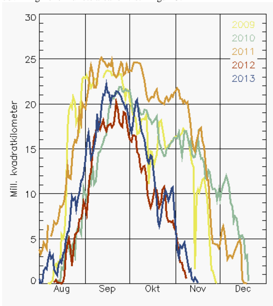
Figur 15. Udviklingen i det antarktiske ozonhuls areal de seneste 5 år.
