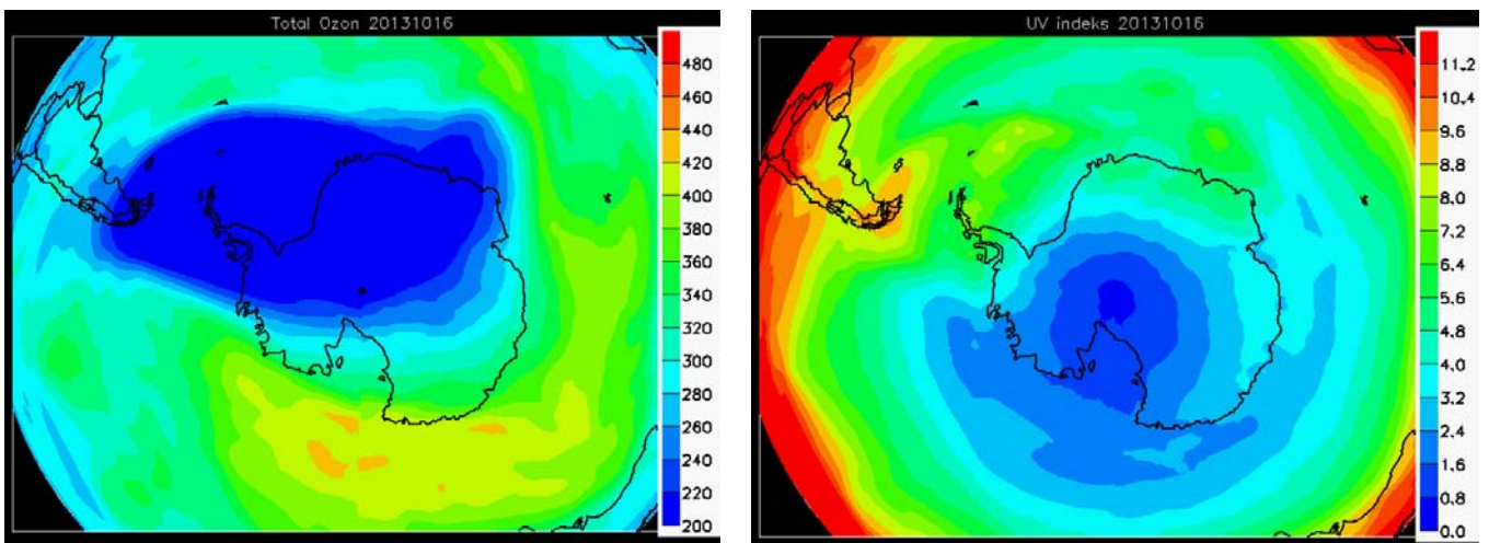
Figur 16. Beregnede UV-indices over det sydlige Amerika 16.oktober 2013 (højre panel) i forbindelse med det antarktiske ozonhul (venstre panel, DU).
