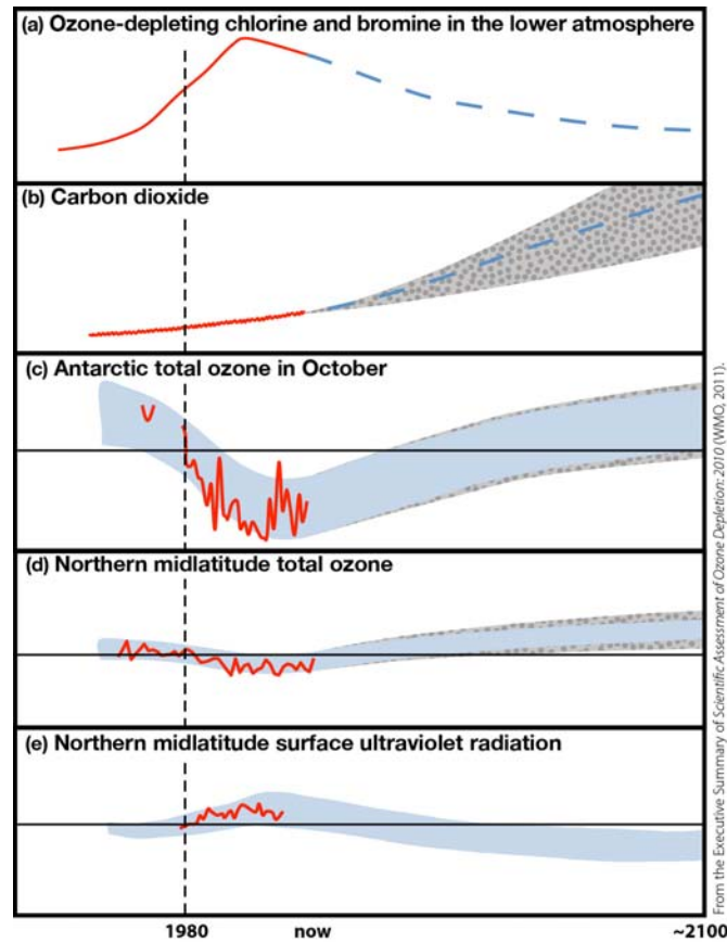
Figur B7. Skematisk udvikling i ozonlaget. De røde kurver repræsenterer observationer op til nu-tiden. De blå stiplede kurver repræsenterer et generelt accepteret scenarie for fremtiden. Skyggede områder repræsenterer årlig variabilitet og usikkerheder i målinger og simuleringer. Den stiplede lodrette linie ved 1980 repræsenterer året, hvor problemerne med nedbrydningen af ozonlaget viste sig for første gang. Kurven for CO 2 er vist, fordi forøgede koncentrationer påvirker temperaturen og vinde (transport) i stratosfæren af betydning for ozonlaget. (WMO, 2011)
