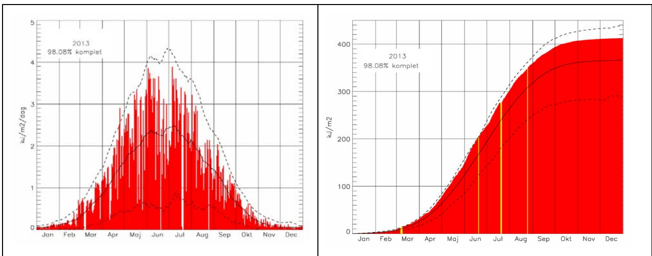
Figur 11 . (Venstre panel) Den dagligt målte totale dosis af hudskadelig UV stråling i 2013 i København i kJ/m 2 /dag. Fuldt optrukken kurve er den tilsvarende middel-dosis for 2000-2010. Øvre og nedre punkterede kurver viser hhv. +2 og -2 standardafvigelser. (Højre panel) Den totale dosis i løbet af året af hudskadelig UV stråling i 2013 i København i kJ/m 2 . Fuldt optrukken kurve er den tilsvarende middel-dosis for 2000-2010. Øvre og nedre punkterede kurver viser hhv. +2 og -2 standardafvigelser.
