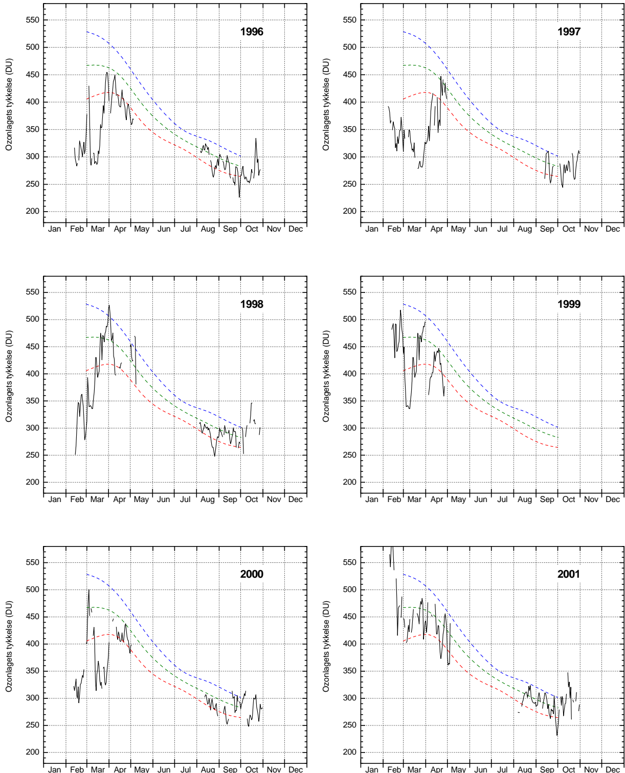
Figur A3b. Ozonlagets tykkelse over Pituffik 1996-2001. Daglige målinger med SAOZ-spektrometeret. Den grønne linje angiver middelværdien af daglige målinger i ti-års perioden 1979-1988 målt med TOMS-instrumentet ombord på Nimbus7-satellitten. De blå og røde stiplede linjer angiver plus og minus en standardafvigelse fra middelværdien. Det betyder, at 2/3 af alle målinger i perioden 1979-1988 ligger mellem den blå og den røde linje.
